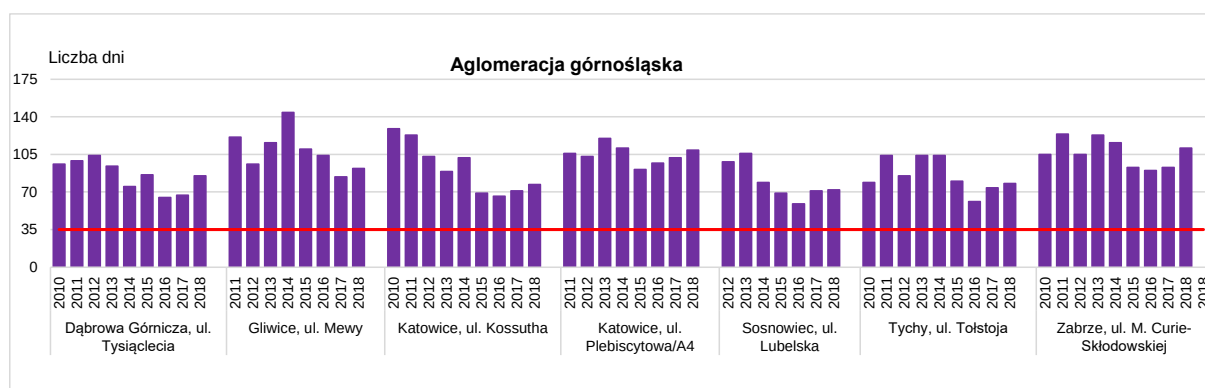
Rysunek 7.51. Liczba dni z przekroczeniem stężeń dobowych pyłu PM10 powyżej 50 µg/m³ w aglomeracji górnośląskiej w latach 2010-2018
