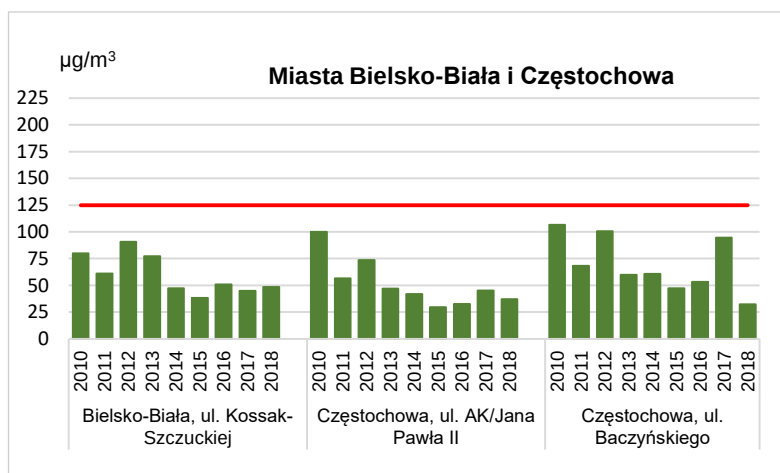
Rysunek 7.6. Stężenia 24-godzinne dwutlenku siarki (4 maksymalne) w strefach miejskich w Bielsku-Białej i w Częstochowie w latach 2010-2018 (poziom dopuszczalny stężenia 24-godz. 125 \mu\text{g}/\text{m}^3 )
