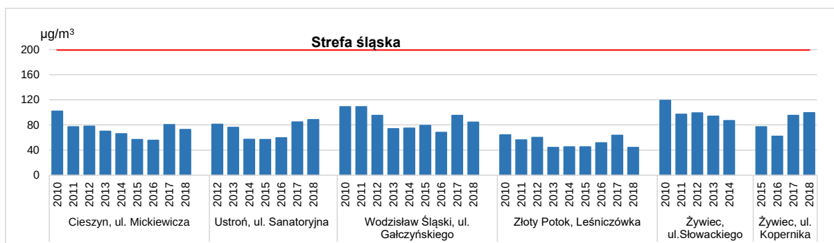
Rysunek 7.22. Stężenia 1-godzinne dwutlenku azotu (19 maksymalne) w strefie śląskiej w latach 2010-2018 (poziom dopuszczalny stężenia 1-godz. 200 µg/m³)
