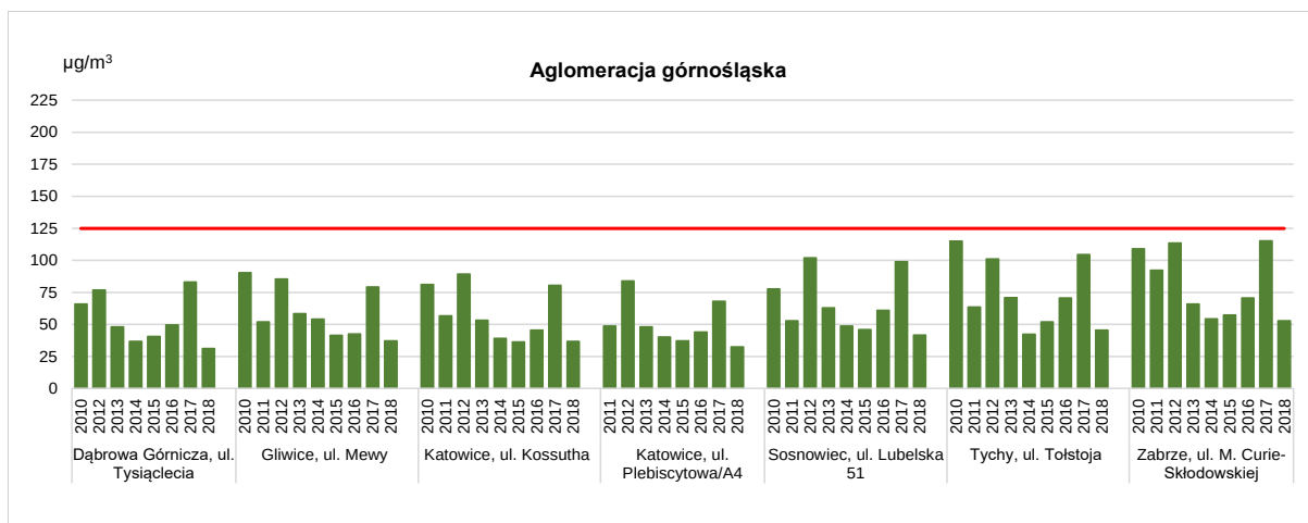
Rysunek 7.7. Stężenia 24-godzinne dwutlenku siarki (4 maksymalne) w aglomeracji górnośląskiej w latach 2010-2018 (poziom dopuszczalny stężenia 24-godz. 125 µg/m³)
