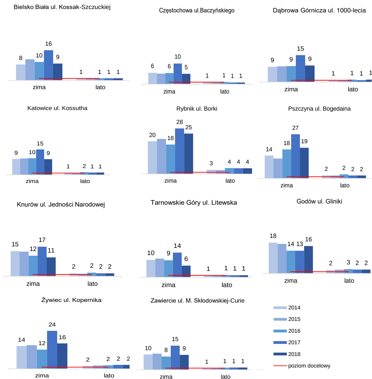
Rysunek 7.83. Średnie stężenia benzo(a)pirenu w ng/m³ w sezonach zimowych i letnich w latach 2014-2018
