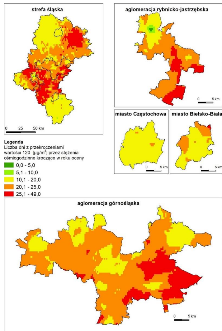
Rysunek 7.42. Rozkład przestrzenny liczby dni, w których najwyższa ośmiogodzinna średnia krocząca stężenie ozonu jest wyższe niż 120 \text{ } \mu\text{g}/\text{m}^3 na obszarze województwa śląskiego w 2018 roku
