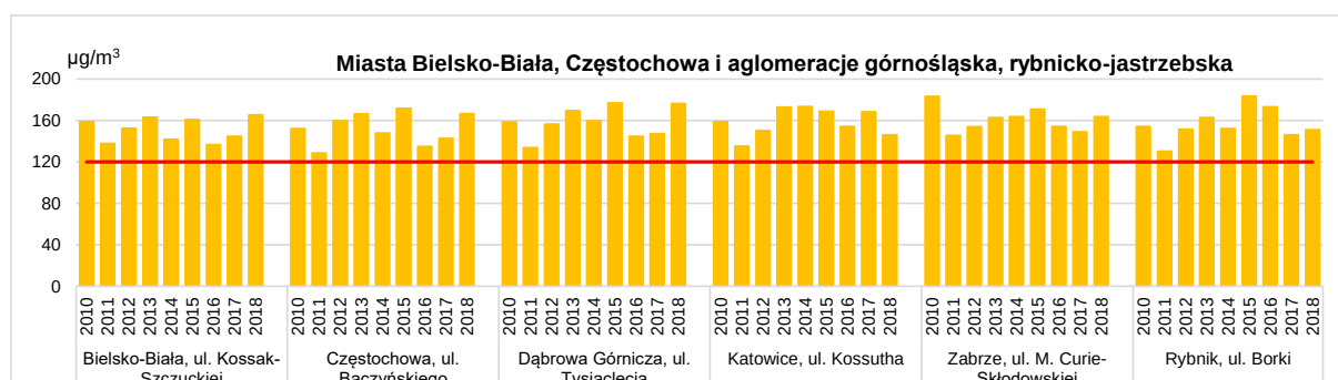
Rysunek 7.40. Najwyższa ośmiogodzinna średnia krocząca stężen ozonu w Bielsku-Białej, Częstochowie, aglomeracjach górnośląskiej i rybnicko-jastrzębskiej w latach 2010-2018
