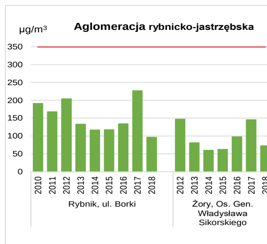
Rysunek 7.4. Stężenia 1-godzinne dwutlenku siarki (25 maksymalne) w aglomeracji rybnicko-jastrzębskiej w latach 2010-2018 (poziom dopuszczalny stężenia 1-godz. 350 \mu\text{g}/\text{m}^3 )
