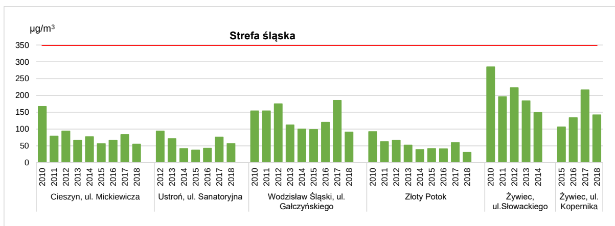
Rysunek 7.5. Stężenia 1-godzinne dwutlenku siarki (25 maksymalne) w strefie śląskiej w latach 2010-2018 (poziom dopuszczalny stężenia 1-godz. 350 \mu\text{g}/\text{m}^3 )
