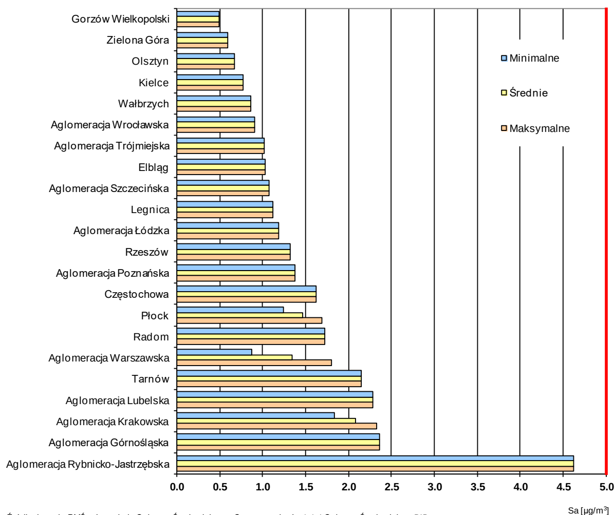
Rys. 3.4-1. Średnie roczne stężenia benzenu uzyskane z pomiarów (automatycznych i manualnych) prowadzonych w 2016 r. na terenie aglomeracji i miast powyżej 100 tys. mieszkańców (poziom dopuszczalny – 5 µg/m³)
