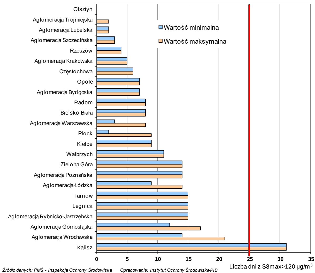
Rys. 3.5-1. Liczba dni z przekroczeniami poziomu docelowego 120 µg/m³ przez stężenia 8-godz. kroczące ozonu w 2016 roku, określona na podstawie pomiarów na terenie aglomeracji i miast powyżej 100 tys. mieszkańców
