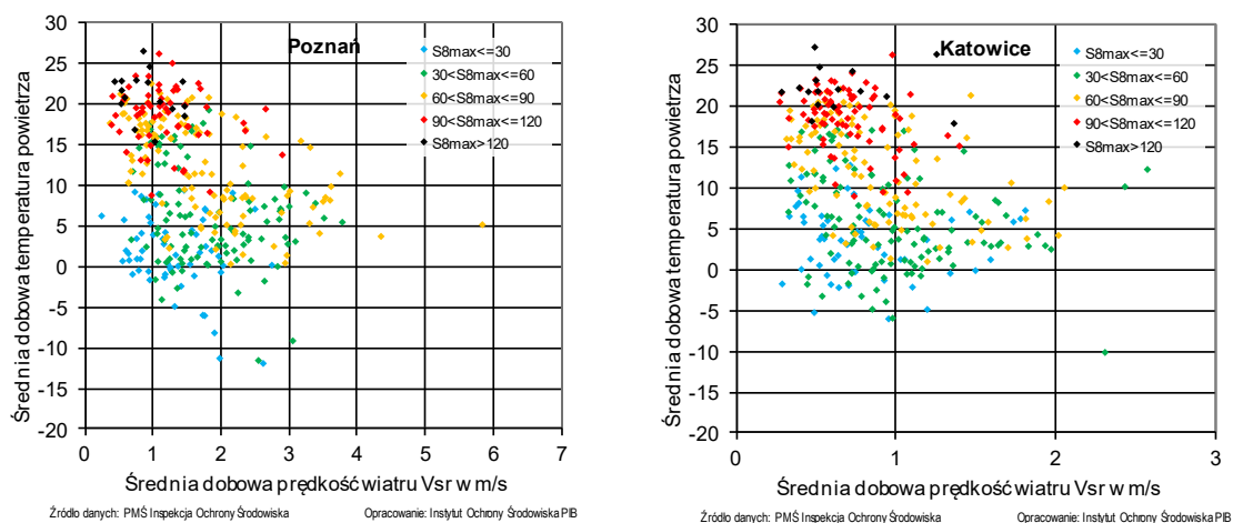
Rys. 4.2-14. Maksyma dobowe stężeń 8-godz. ozonu w 2016 r. w zależności od średniej dobowej prędkości wiatru i średniej dobowej temperatury powietrza
