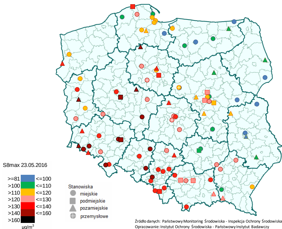
Rys. 4.2-8. Maksima dzienne ze stężeń 8-godz. kroczących ozonu w dniu 23.05.2016 r.
