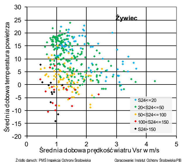
Rys. 5.2-14. Stężenia 24-godz. pyłu PM10 w 2016 r. w zależności od średniej dobowej prędkości wiatru i średniej dobowej temperatury powietrza na stacji w Żywcu (SlŻywieKoper)
