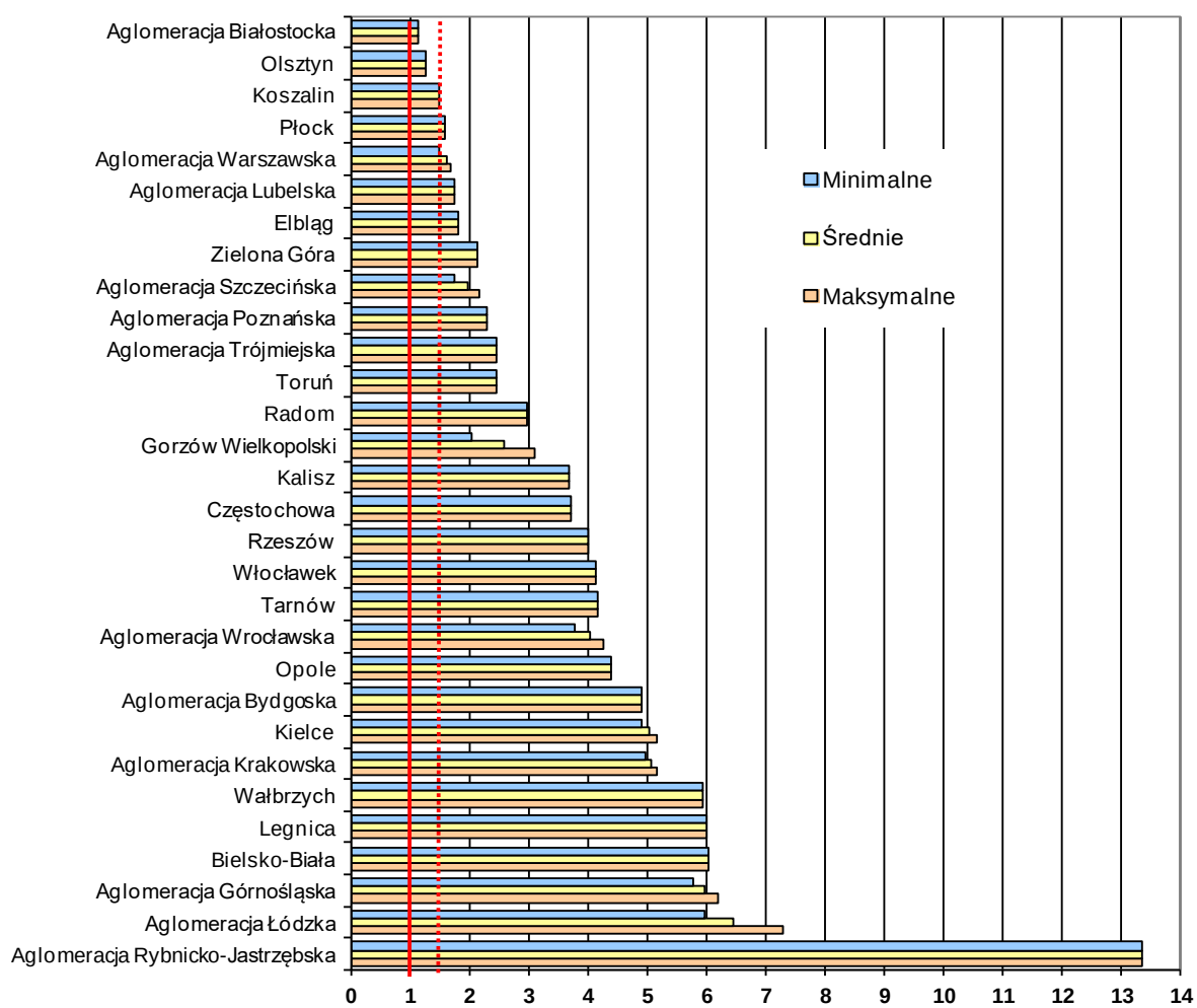
Rys. 3.11-1. Wartości średnich rocznych stężeń benzo(a)pirenu (BaP) uzyskane w 2016 r. z pomiarów na terenie aglomeracji i miast powyżej 100 tys. mieszkańców
