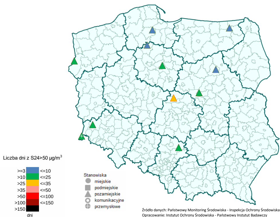
Rys. 5.4-6. Liczba dni w 2016 r. ze stężeniem 24-godz. pyłu PM10 wyższym od 50 µg/m 3 określona na podstawie pomiarów na stanowiskach pozamiejskich
