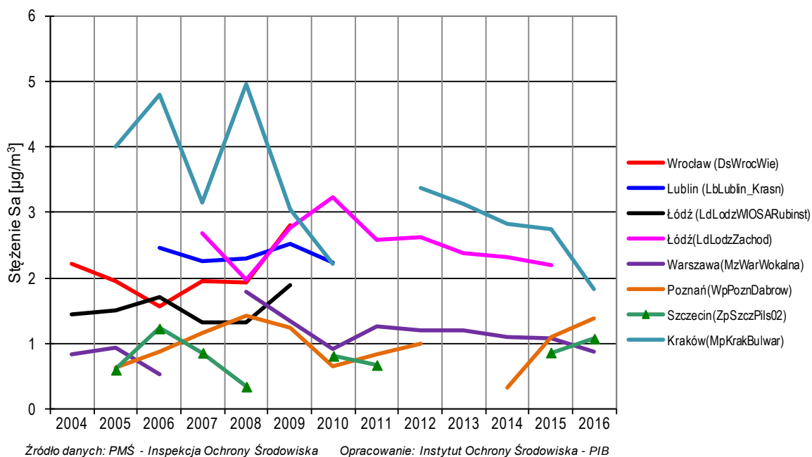
Rys. 3.4-2. Stężenie średnie roczne benzenu w latach 2004-2016 na wybranych stanowiskach w aglomeracjach w Polsce (poziom dopuszczalny – 5 µg/m 3 )
