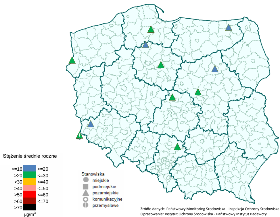
Rys. 5.4-4. Stężenia średnie roczne pyłu PM10 w 2016 r. na stanowiskach pozamiejskich
