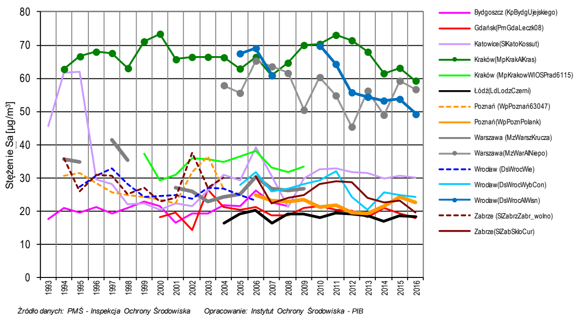
Rys. 3.2-3. Stężenie średnie roczne dwutlenku azotu w latach 1993-2016 na wybranych stanowiskach w aglomeracjach w Polsce (linie z kropkami oznaczają stanowiska „komunikacyjne”)
