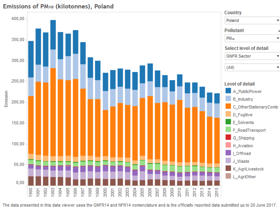
Rys. 5.5-2. Emisja pyłu PM 10 z Polski w latach 1990-2015.
