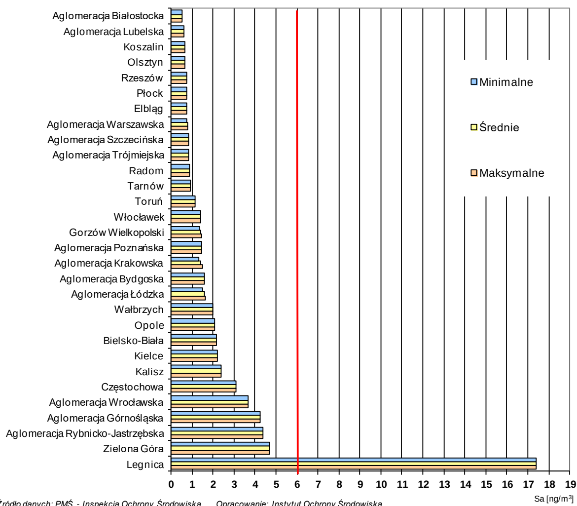
Rys. 3.8-1. Wartości średnich rocznych stężeń arsenu (As) uzyskane w 2016 r. z pomiarów na terenie aglomeracji i miast powyżej 100 tys. mieszkańców
