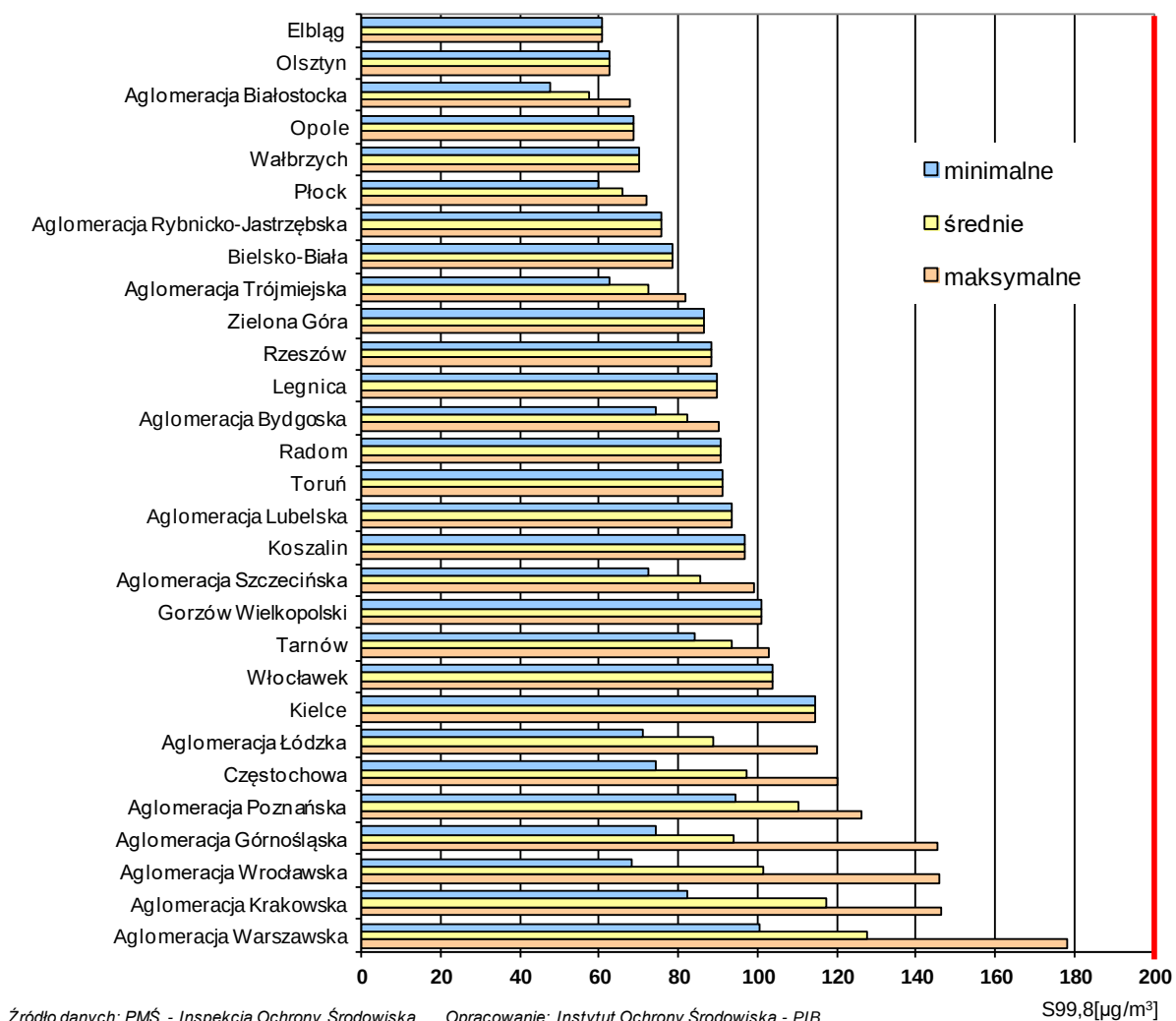
Rys. 3.2-2. Wartości percentyla S99.8 ze stężeń 1-godzinnych \text{NO}_2 uzyskane z pomiarów prowadzonych w 2016 r. na terenie aglomeracji i miast powyżej 100 tys. mieszkańców
