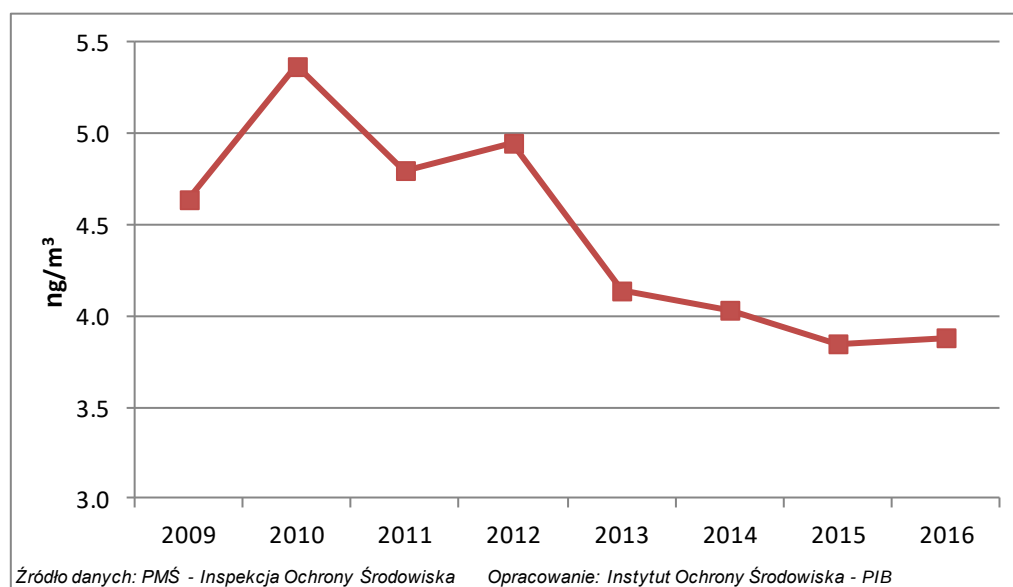
Rys. 3.11-2. Stężenie średnie roczne B(a)P w latach 2009-2016, uśrednione dla wszystkich stanowisk uwzględnionych w analizach (zlokalizowanych na terenie aglomeracji i dużych miast)
