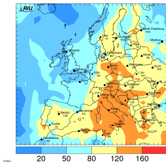
Rys. 4.2-10. Prognoza dobowych stężeń maksymalnych 8-godz. ozonu w Europie na dzień 23.05.2016 r. Źródło: http://www.uni-koeln.de/math-nat-fak/geomet/eurad/index_e.html
