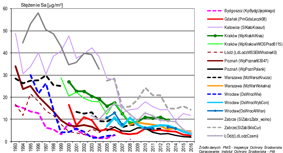
Rys. 3.1-3. Stężenie średnie roczne dwutlenku siarki w latach 1993-2016 na wybranych stanowiskach w aglomeracjach w Polsce
