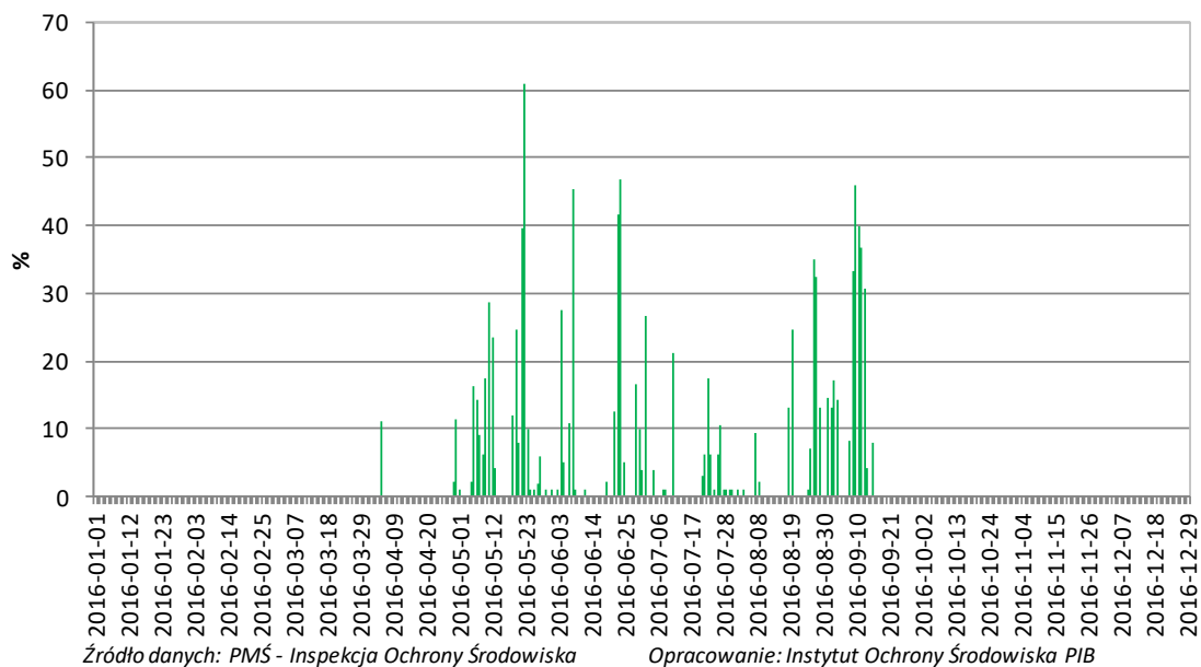
Rys. 4.2-7. Procent stanowisk, na których w danym dniu 2016 r. wystąpiło stężenie 8 godz. ozonu wyższe od 120 \mu\text{g}/\text{m}^3
