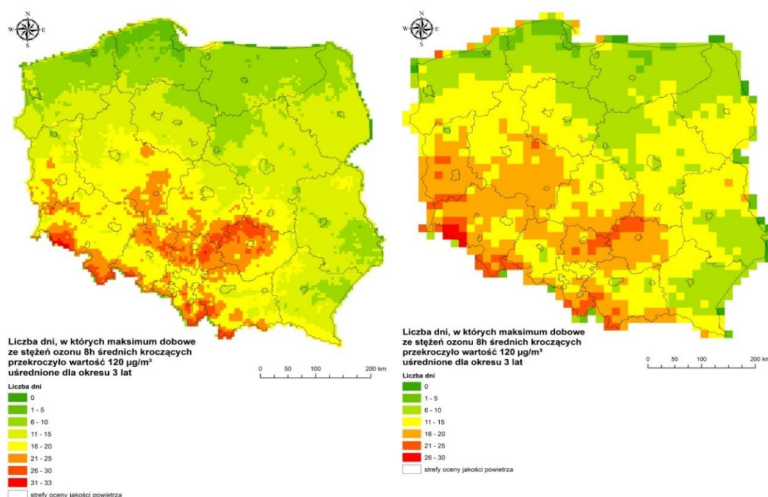
Rys. 4.4-4. Uśredniona liczba dni z przekroczeniami wartości 120 µg/m³ przez stężenia 8-godz. ozonu w latach 2014-2016 r. oszacowana na podstawie wyników modelowania (w węzłach siatki kwadratów o boku 5 km – lewy rysunek i 15 km – prawy rysunek) i pomiarów. Źródło: Wyniki modelowania stężeń ozonu troposferycznego na potrzeby rocznej oceny jakości powietrza dla roku 2016. GIOŚ 2017a
