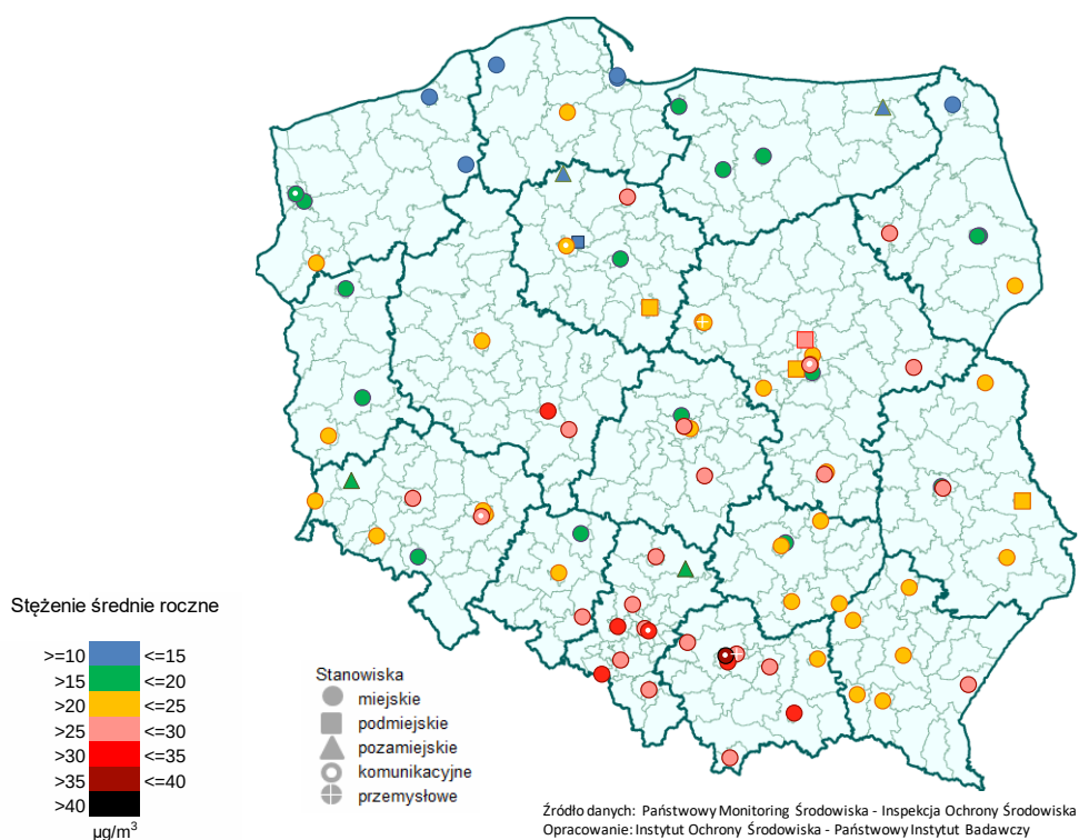
Rys. 6.2-1. Stężenia średnie roczne pyłu PM 2.5 w 2016 r.
