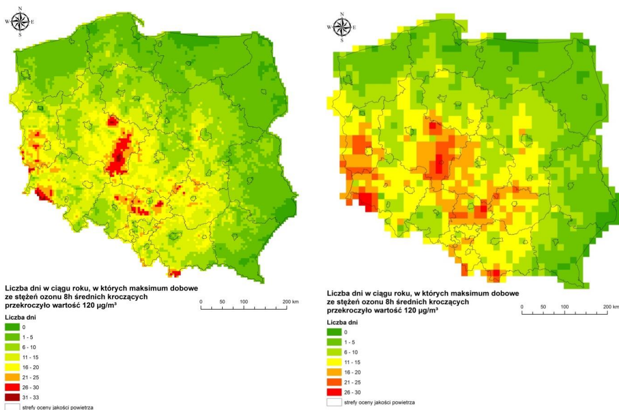
Rys. 4.2-2. Liczba dni z przekroczeniami wartości 120 µg/m³ przez stężenia 8-godz. ozonu w 2016 r. oszacowana na podstawie wyników modelowania (w węzłach siatki kwadratów o boku 5 km – lewy rysunek i 15 km – prawy rysunek) i pomiarów. Źródło: Wyniki modelowania stężeń ozonu troposferycznego na potrzeby rocznej oceny jakości powietrza dla roku 2016. Atmoterm 2017
