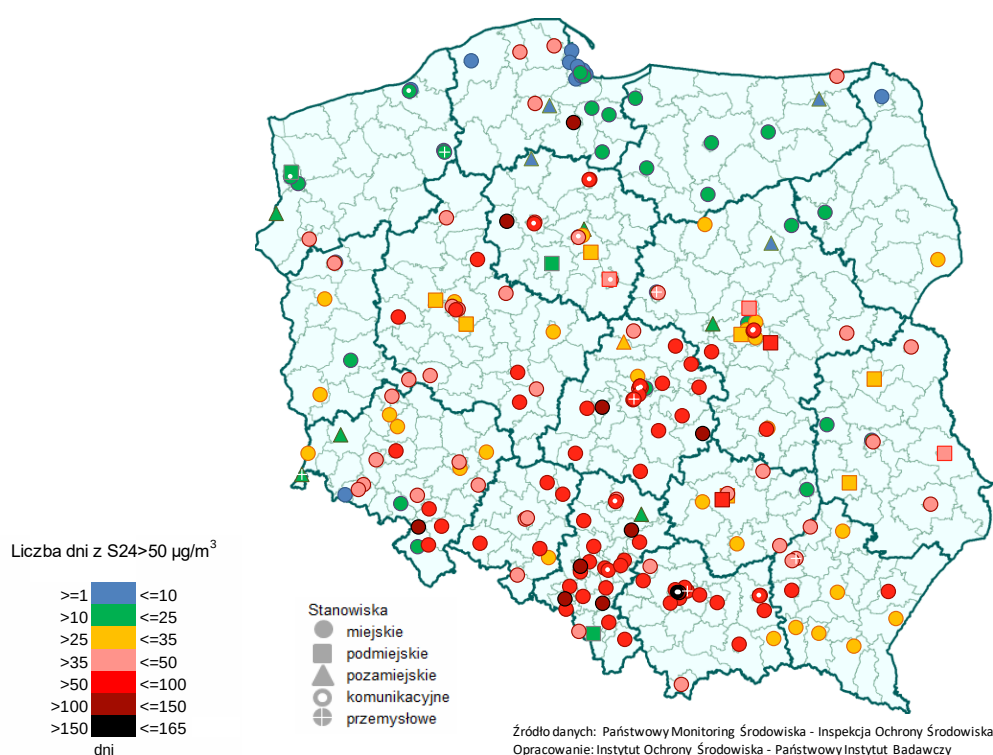
Rys. 5.2-5. Liczba dni z przekroczeniami poziomu 50 \mu\text{g}/\text{m}^3 przez stężenia 24-godz. PM10 w 2016 r.
