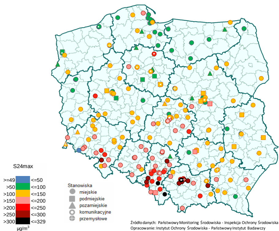
Rys. 5.2-6. Maksymalne stężenia 24-godz. PM10 (S24max) zarejestrowane w 2016 r.
