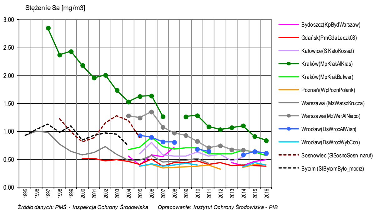
Rys. 3.3-2. Stężenie średnie roczne tlenku węgla w latach 1995-2016 na wybranych stanowiskach w aglomeracjach w Polsce (linie z kropkami oznaczają stanowiska „komunikacyjne”)
