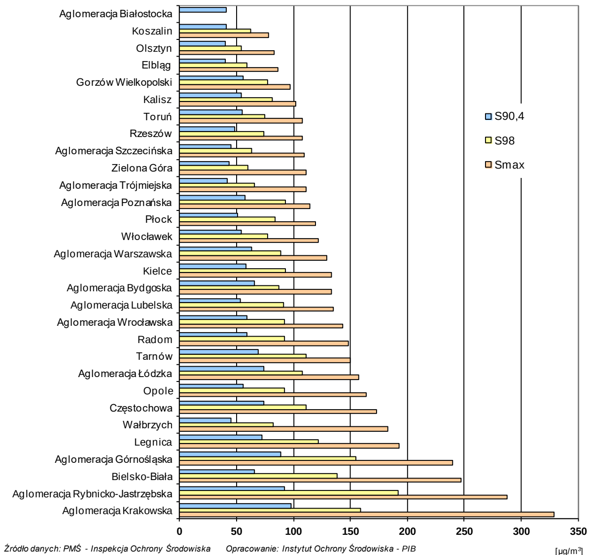
Rys. 3.6-3. Najwyższe wartości percentyli S90.4 i S98 oraz stężenia maksymalnego S24max dla 24-godzinnych stężeń pyłu PM10, uzyskane z pomiarów prowadzonych w 2016 r. na terenie aglomeracji i miast powyżej 100 tys. mieszkańców
