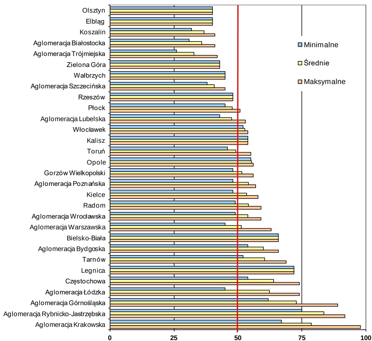
Rys. 3.6-2. Wartości percentyla S90.4 ze stężeń 24-godzinnych pyłu PM10 uzyskane z pomiarów prowadzonych w 2016 r. na terenie aglomeracji i miast powyżej 100 tys. mieszkańców
