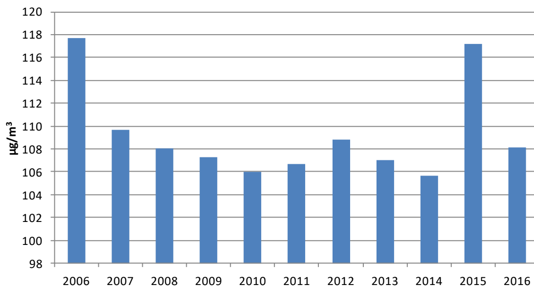
Rys. 3.5-5. Uśrednione dla wszystkich stanowisk uwzględnionych w analizach (zlokalizowanych na terenie aglomeracji i dużych miast) wartości percentyla S93.2 z rocznych serii maksimów dobowych stężeń 8-godz. kroczących ozonu w latach 2006-2016
