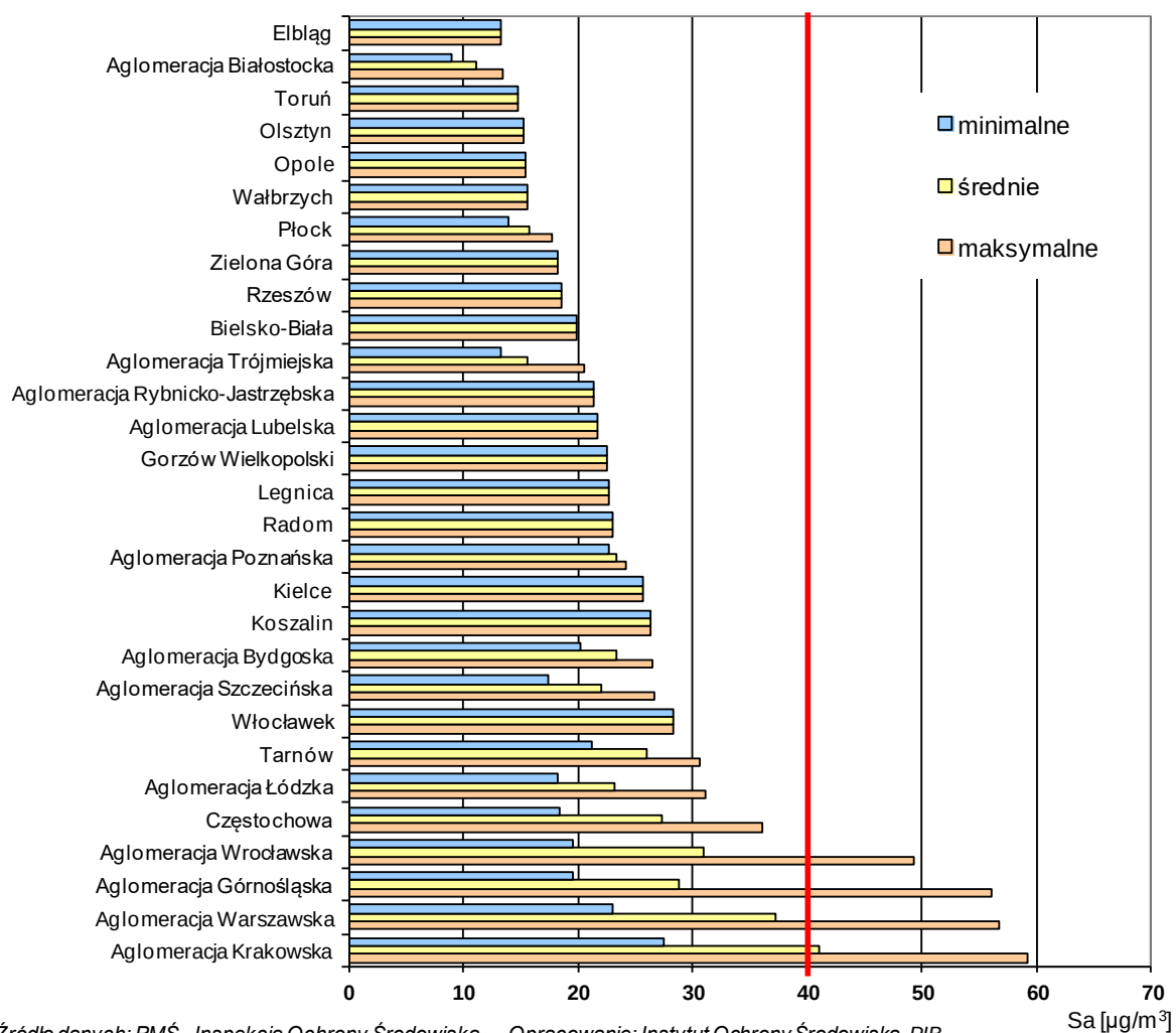
Rys. 3.2-1. Średnie roczne stężenia NO 2 uzyskane z pomiarów prowadzonych w 2016 r. na terenie aglomeracji i miast powyżej 100 tys. mieszkańców
