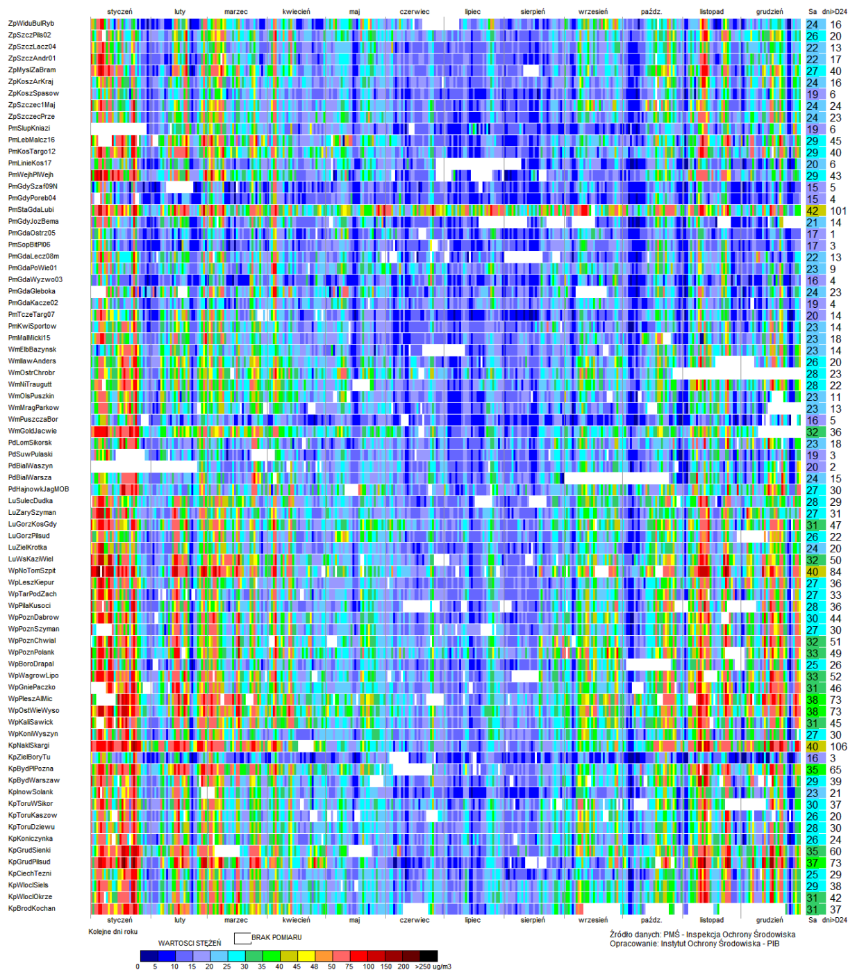
Rys. 5.2-7-A. Przebieg stężeń 24-godz. pyłu PM10 w 2016 r. na stanowiskach, z których wyniki wykorzystano w ocenie (dwie pierwsze litery w kodzie stanowisk to skrót nazwy województwa, na obszarze którego zlokalizowane jest stanowisko, np. Pd - podlaskie, Lu - lubuskie itd.)
