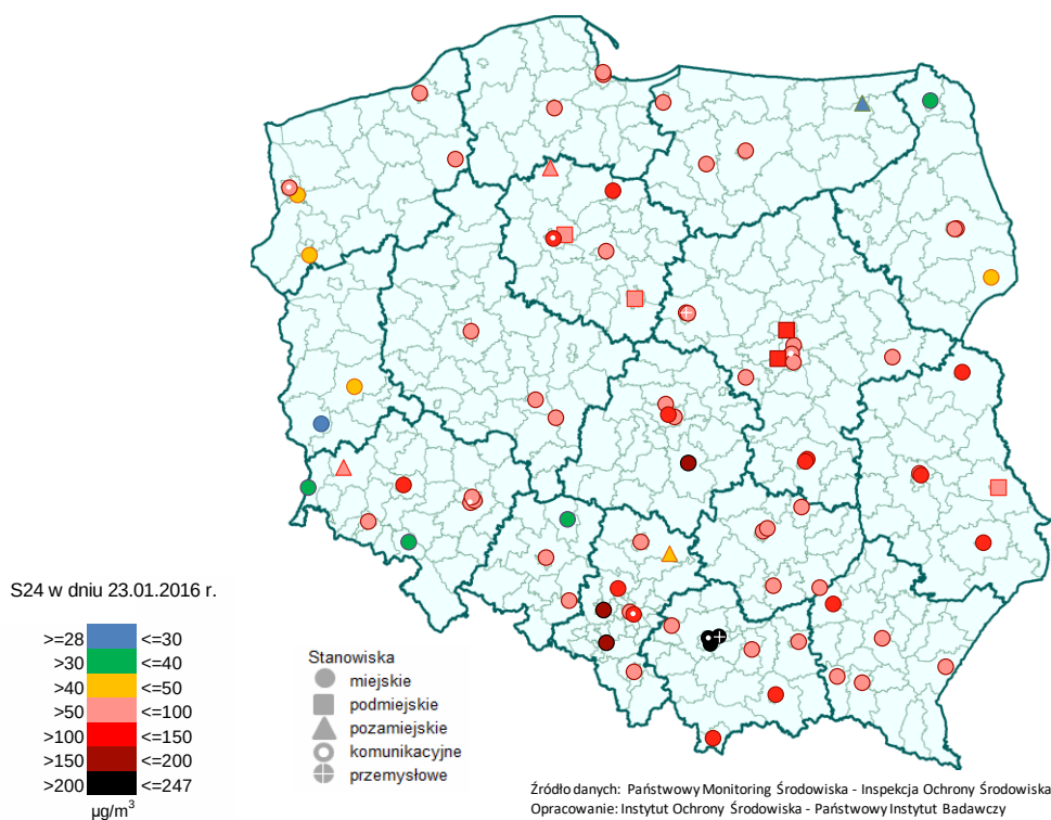
Rys. 6.2-5. Stężenia 24-godz. pyłu PM 2.5 w dniu 23.01.2016 r.
