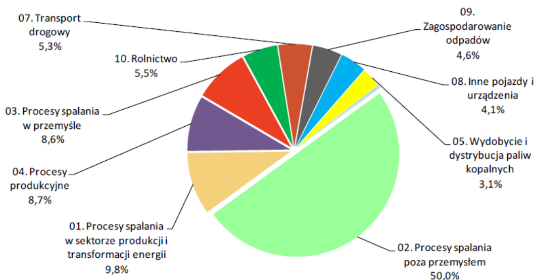
Rys. 5.5-1. Udział poszczególnych sektorów w emisji pyłu PM10 w Polsce w roku 2015. Źródło: IOŚ-PIB KOBIZE 2017
