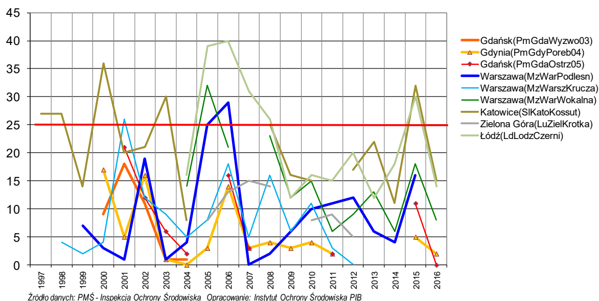
Rys. 3.5-4. Liczba dni ze stężeniami 8-godz. ozonu przewyższającymi 120 \mu\text{g}/\text{m}^3 w latach 1997-2016 na wybranych stanowiskach w aglomeracjach w Polsce
