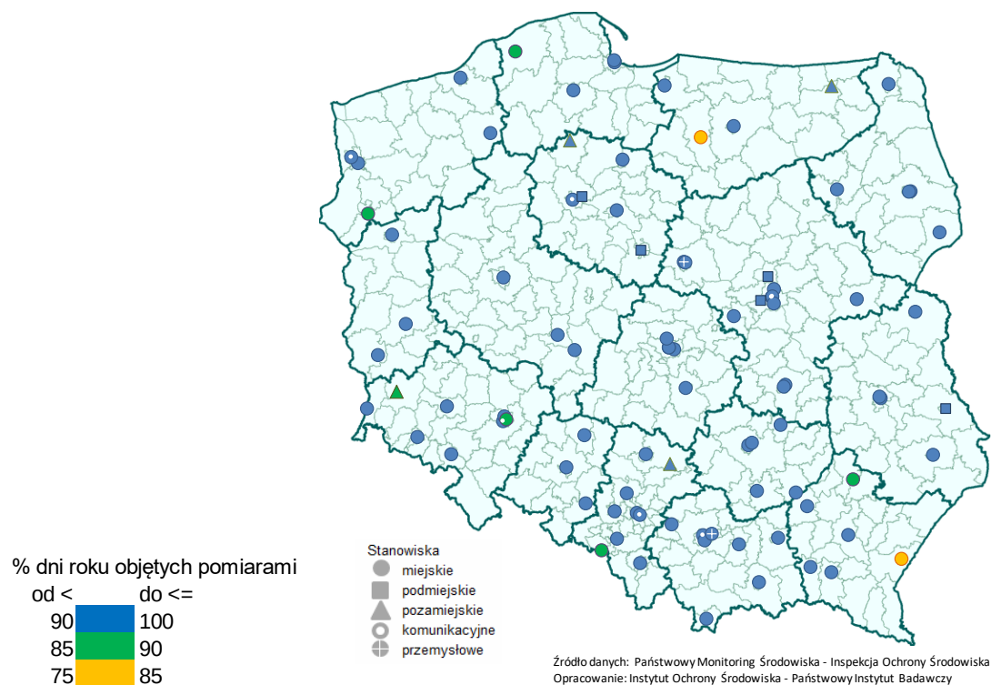
Rys. 6.1-1. Lokalizacja stanowisk pomiarów stężeń pyłu PM 2.5 , z których dane wykorzystano w raporcie za 2016 rok, z uwzględnieniem typu stanowiska, rodzaju obszaru lokalizacji i kompletności serii pomiarowej
