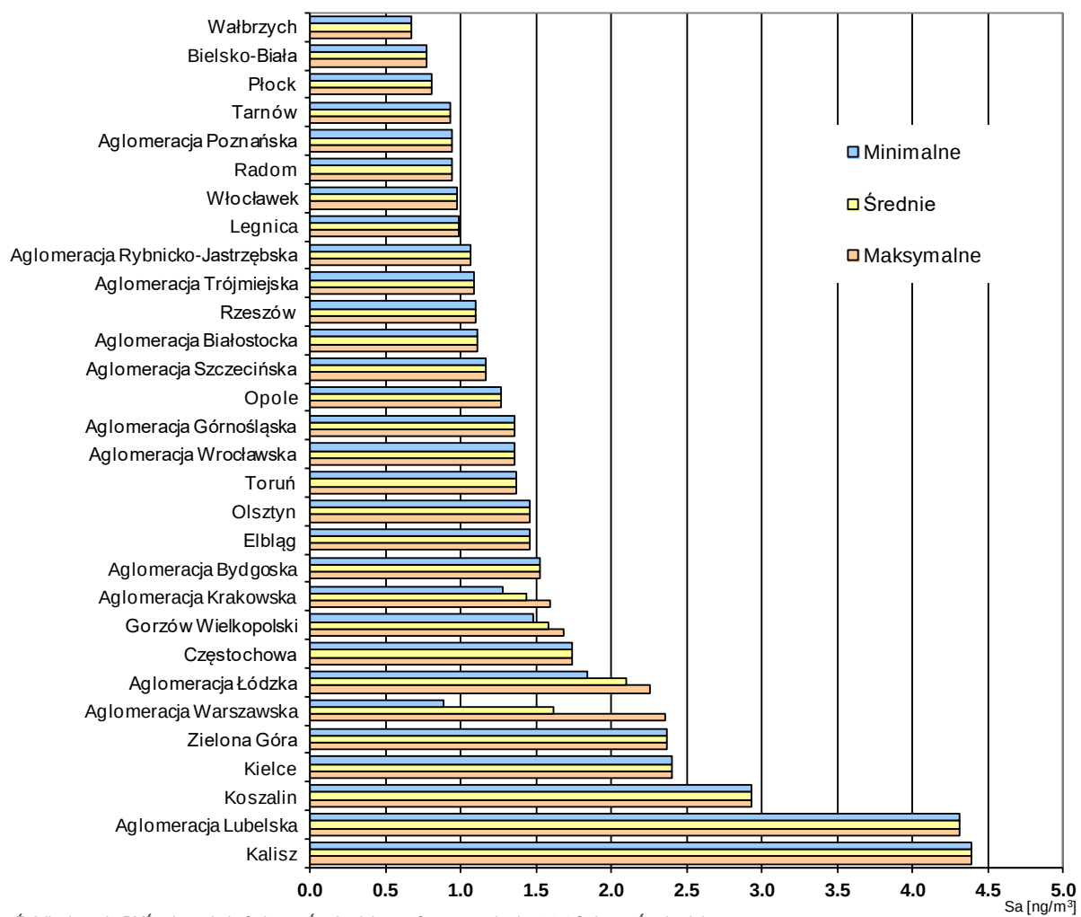
Rys. 3.10-1. Wartości średnich rocznych stężeń niklu (Ni) uzyskane w 2016 r. z pomiarów na terenie aglomeracji i miast powyżej 100 tys. mieszkańców.
