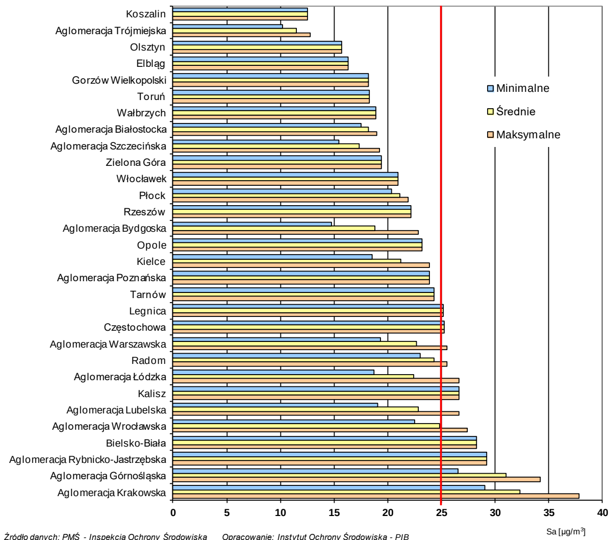
Rys. 3.12-1. Średnie roczne stężenia pyłu PM 2.5 uzyskane z pomiarów prowadzonych w 2016 r. na terenie aglomeracji i miast powyżej 100 tys. mieszkańców
