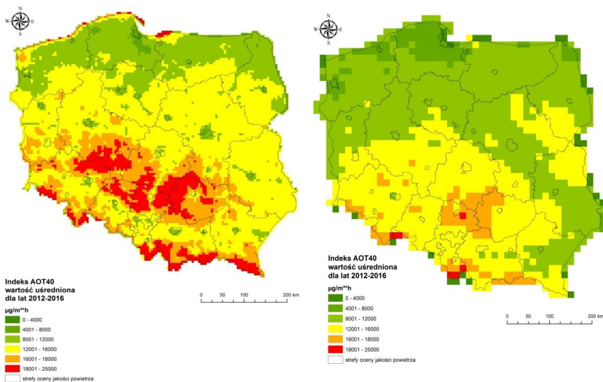
Rys. 4.5-2. Parametr AOT40 [ \mu\text{g}/\text{m}^3\cdot\text{h} ] obliczony dla okresu maj-lipiec, uśredniony dla 5 lat 2012-2016 r., oszacowany na podstawie wyników modelowania (w węzłach siatki kwadratów o boku 5 km – lewy rysunek i 15 km – prawy rysunek) i pomiarów. Źródło: Wyniki modelowania stężeń ozonu troposferycznego na potrzeby rocznej oceny jakości powietrza dla roku 2016. Atmoterm 2017
