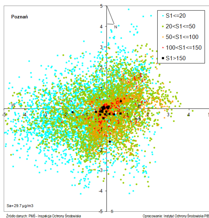
Rys. 5.2-12. Stężenia 1-godz. pyłu PM10 w 2016 r. w zależności od prędkości i kierunku wiatru na stacji w Poznaniu (WpPoznDabrow)
