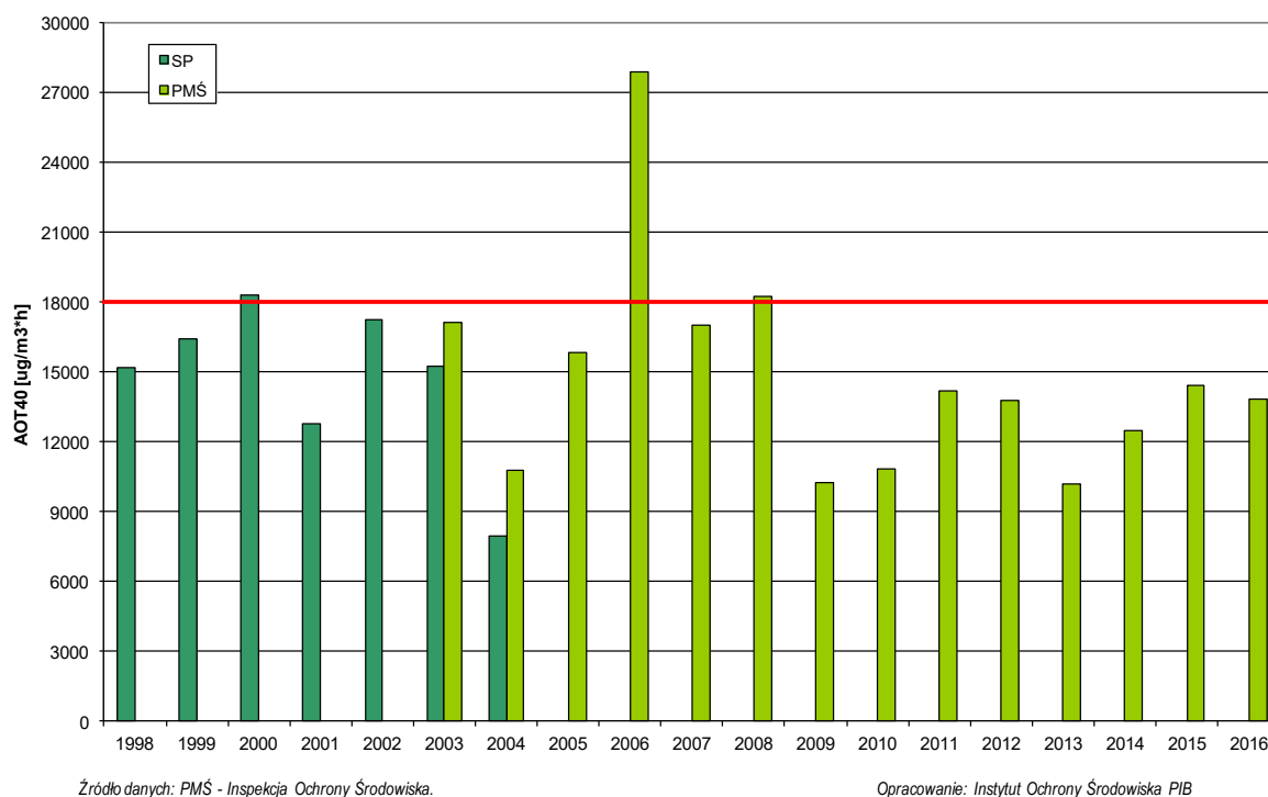
Rys. 4.3-3. Wartości parametru AOT40 obliczone dla pojedynczych lat z okresu maj-lipiec; dla lat 1998-2004 uśrednione dla wszystkich pozamiejskich stanowisk pomiarowych stężeń ozonu należących uprzednio do sieci podstawowej (SP) oraz dla lat 2003-2016 r. dla wszystkich podmiejskich i pozamiejskich stanowisk włączonych do Państwowego Monitoringu Środowiska (PMŚ) uwzględnionych w analizach (PMŚ)
