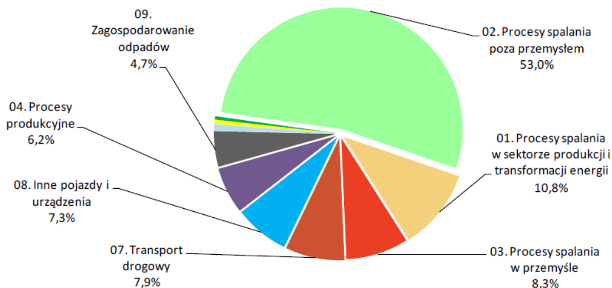
Rys. 6.5-1. Udział poszczególnych sektorów w emisji pyłu PM2.5 w Polsce w roku 2015
