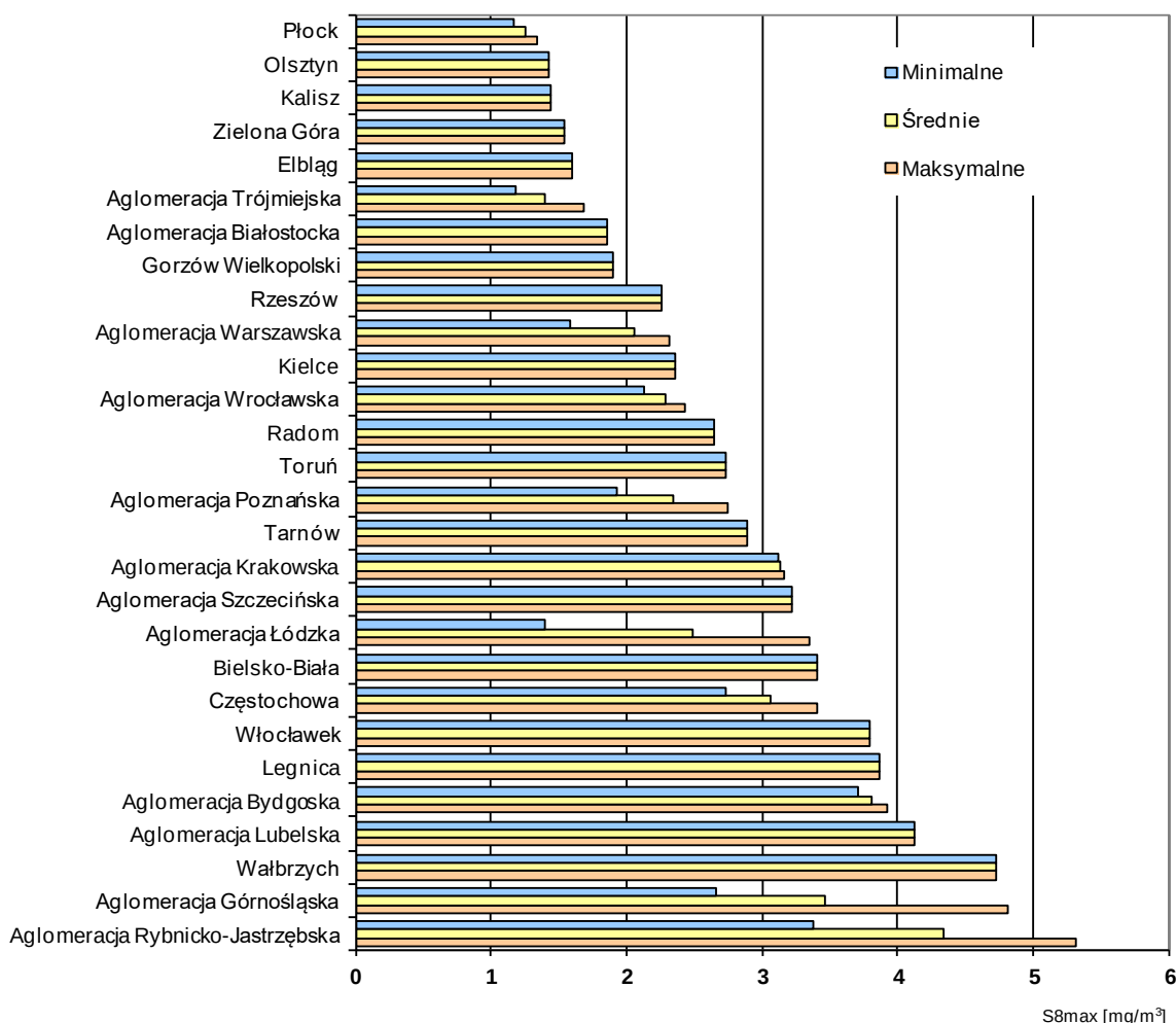
Rys. 3.3-1. Stężenia maksymalne 8-godz. tlenu węgla uzyskane z pomiarów prowadzonych w 2016 r. na terenie aglomeracji i miast powyżej 100 tys. mieszkańców (poziom dopuszczalny – 10 mg/m 3 )
