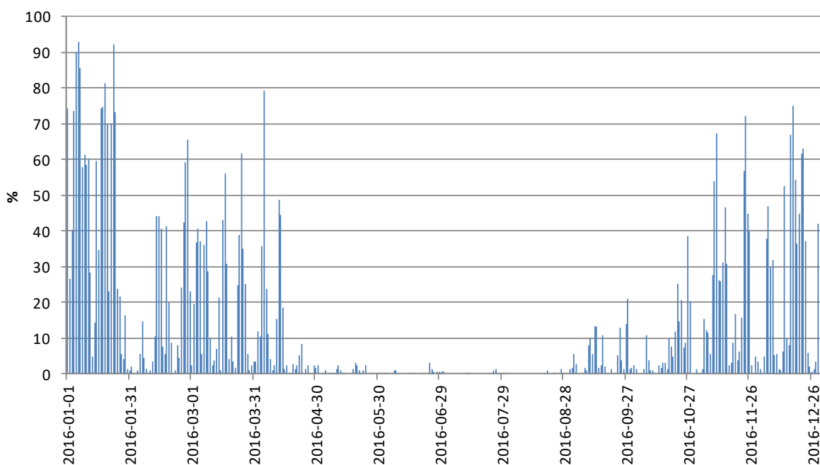
Rys. 5.2-9. Procent stanowisk pomiarowych stężeń pyłu PM10, na których stężenie 24-godz. w 2016 r. przekraczało wartość 50 \mu\text{g}/\text{m}^3 (spośród wszystkich stanowisk, na których w danym dniu pomiary były prowadzone)
