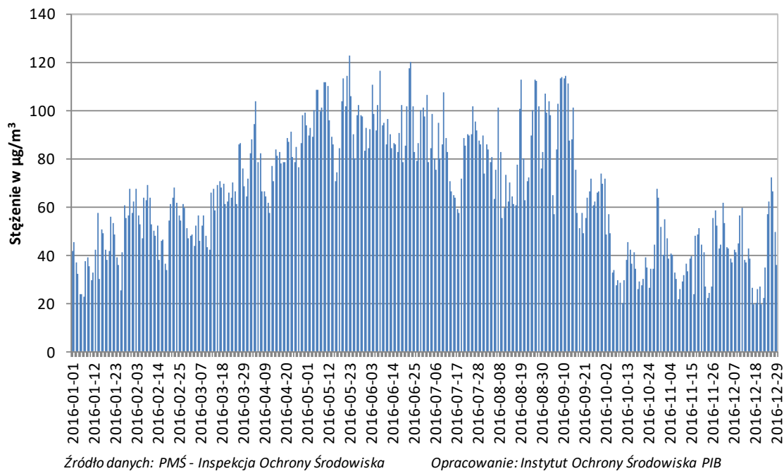
Rys. 4.2-6. Uśrednione dla wszystkich stanowisk w kraju maksima dobowe ze stężeń 8-godz. ozonu w 2016 r.
