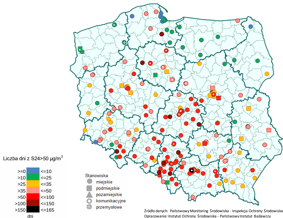
Rys. 5.4-3. Liczba dni w 2016 r. ze stężeniem 24-godz. pyłu \text{PM}_{10} wyższym od 50 \mu\text{g}/\text{m}^3 określona na podstawie pomiarów na stanowiskach miejskich i podmiejskich
