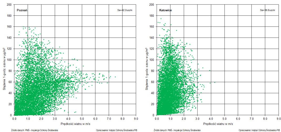
Rys. 4.2-13. Stężenia 1-godz. ozonu w 2016 r. w zależności od prędkości wiatru na stacjach w Poznaniu i Katowicach
