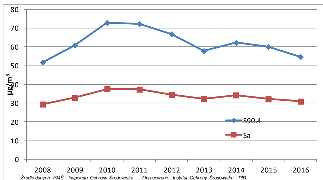
Rys. 3.6-5. Stężenie średnie roczne i percentyl 90.4 ze stężeń 24-godz. pyłu PM10 w latach 2008-2016, uśrednione dla wszystkich stanowisk uwzględnionych w analizach (zlokalizowanych na terenie aglomeracji i dużych miast)
