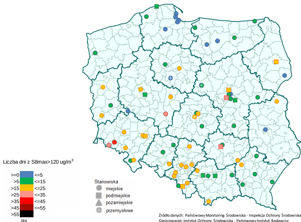
Rys. 4.4-1. Liczba dni z przekroczeniami wartości 120 \mu\text{g}/\text{m}^3 przez stężenia 8-godz. ozonu uśredniona dla 1-3 lat na stanowiskach miejskich i podmiejskich (dopuszczalna liczba dni z przekroczeniami: 25)
