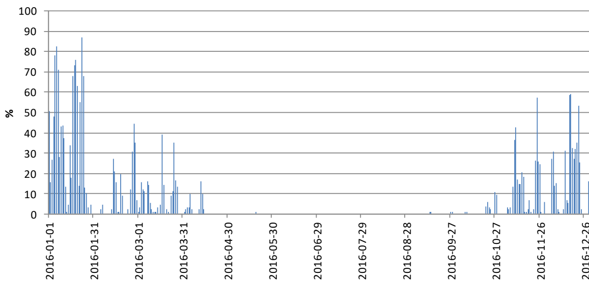
Rys. 6.2-4. Procent stanowisk pomiarowych pyłu PM 2.5 , na których stężenie 24-godz. pyłu PM 2.5 przekraczało wartość 50 µg/m 3 w poszczególnych dniach 2016 r. (spośród wszystkich stanowisk, na których w danym dniu pomiary były prowadzone)
