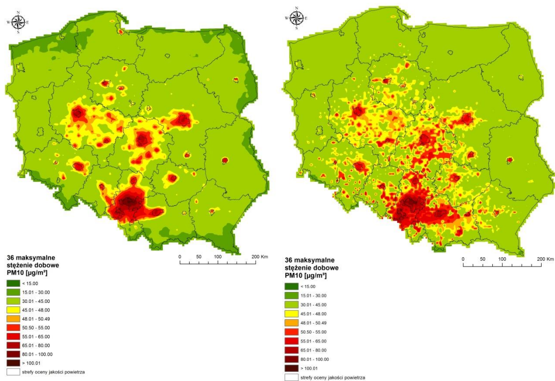
Rys. 5.2-4. Rozkład stężeń 24-godzinnych pyłu PM10 w skali kraju - wynik modelowania CAMx w wariancie I (modelowanie) i II (połączenie modelowania i wyników pomiarów stężeń)
