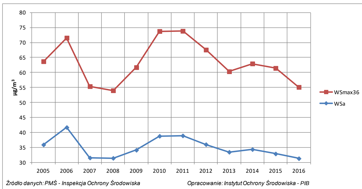
Rys. 5.3-1. Zmiany stężeń średnich rocznych PM10 (wskaźnika WSa) oraz stężeń 24-godz. PM10 (wskaźnika WSmax36) na stanowiskach tła miejskiego i podmiejskiego w Polsce w latach 2005-2016
