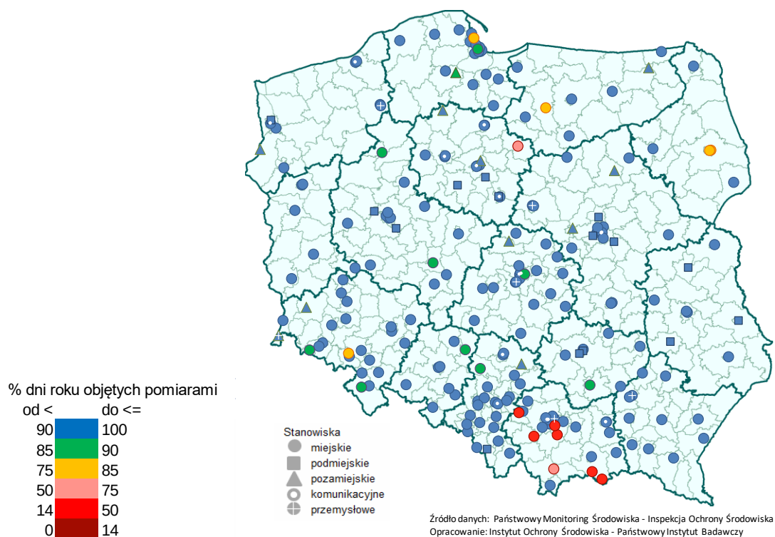
Rys. 5.1-1. Lokalizacja stanowisk pomiarów stężeń pyłu PM10, z których dane wykorzystano w raporcie za 2016 rok, z uwzględnieniem typu stanowiska i obszaru oraz liczebności serii pomiarowej. Na 6 stanowiskach w woj. małopolskim prowadzone były pomiary cykliczne (8 dwutygodniowych okresów pomiarowych rozłożonych równomiernie w ciągu roku).
