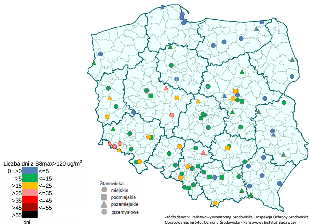
Rys. 4.2-1. Liczba dni z przekroczeniami poziomu 120 \mu\text{g}/\text{m}^3 przez stężenia 8-godz. ozonu w 2016 r.
