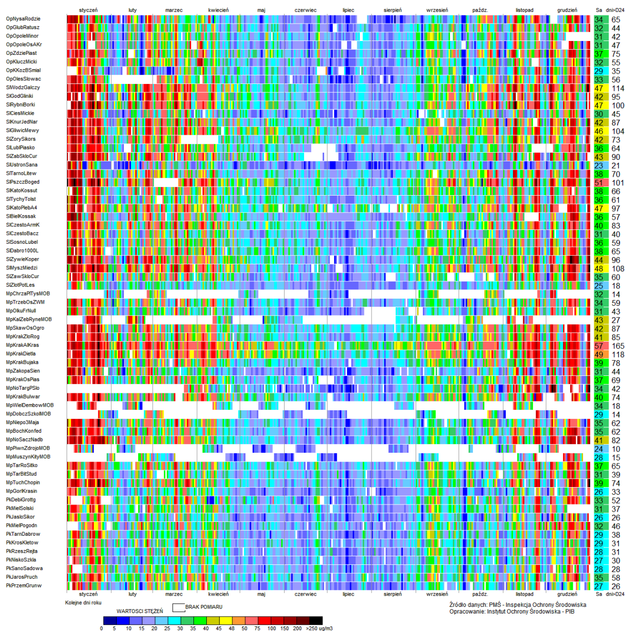
Rys. 5.2-7-C. Przebieg stężeń 24-godz. pyłu PM10 w 2016 r. na stanowiskach, z których wyniki wykorzystano w ocenie (dwie pierwsze litery w kodzie stanowisk to skrót nazwy województwa, na obszarze którego zlokalizowane jest stanowisko, np. Sl - śląskie, Mp - małopolskie itd.)
