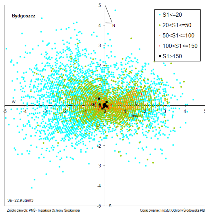
Rys. 6.2-7. Stężenia 1-godz. PM 2.5 w 2016 r. w zależności od prędkości i kierunku wiatru na stacji w Bydgoszczy (kod stacji: KpBydPlPozna)
