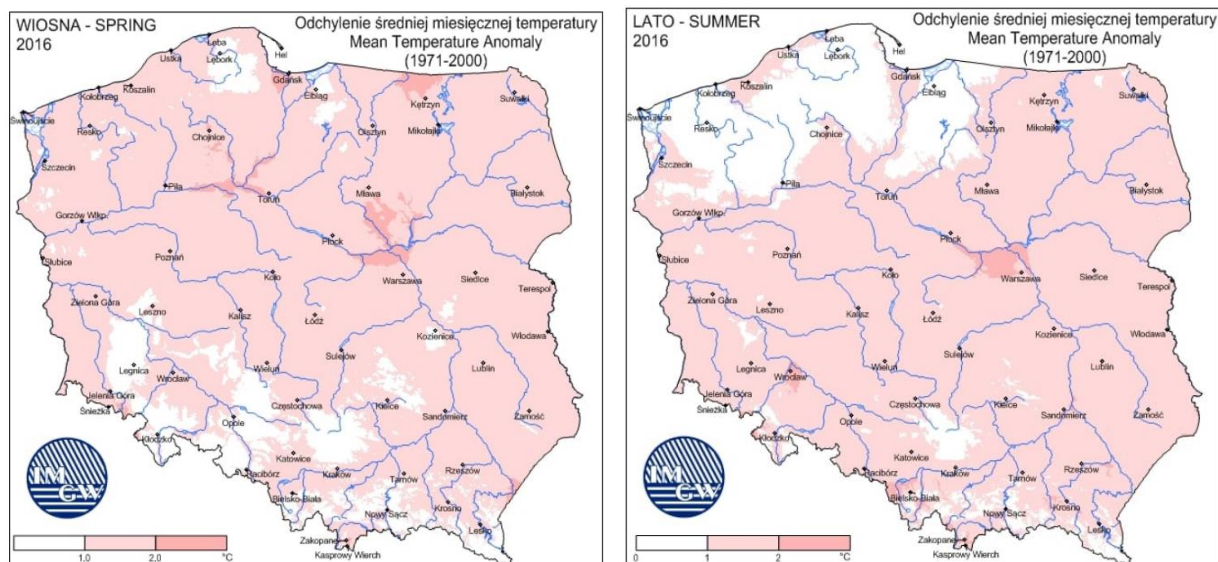
Rys. 4.2-3. Odchylenie średniej temperatury powietrza wiosną i latem 2016 r. od średnich dla wielolecia 1971-2000. Źródło: IMGW-PIB, http://klimat.pogodynka.pl/pl/climate-maps/#Mean_Temperature/Seasonal/2016/1/Spring
