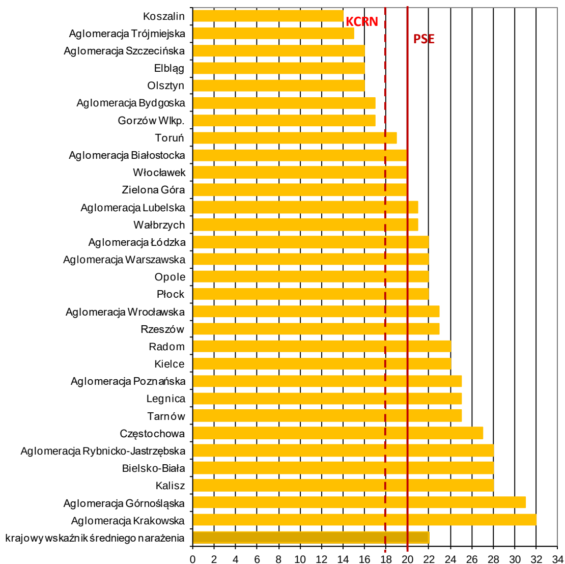
Rys. 3.12-2. Wskaźniki średniego narażenia WM i krajowy wskaźnik średniego narażenia WK dla 2016 r. oraz wartości pułapu stężenia ekspozycji (PSE) (pionowa czerwona linia) i krajowego celu redukcji narażenia (KCRN) (pionowa czerwona przerywana linia)
