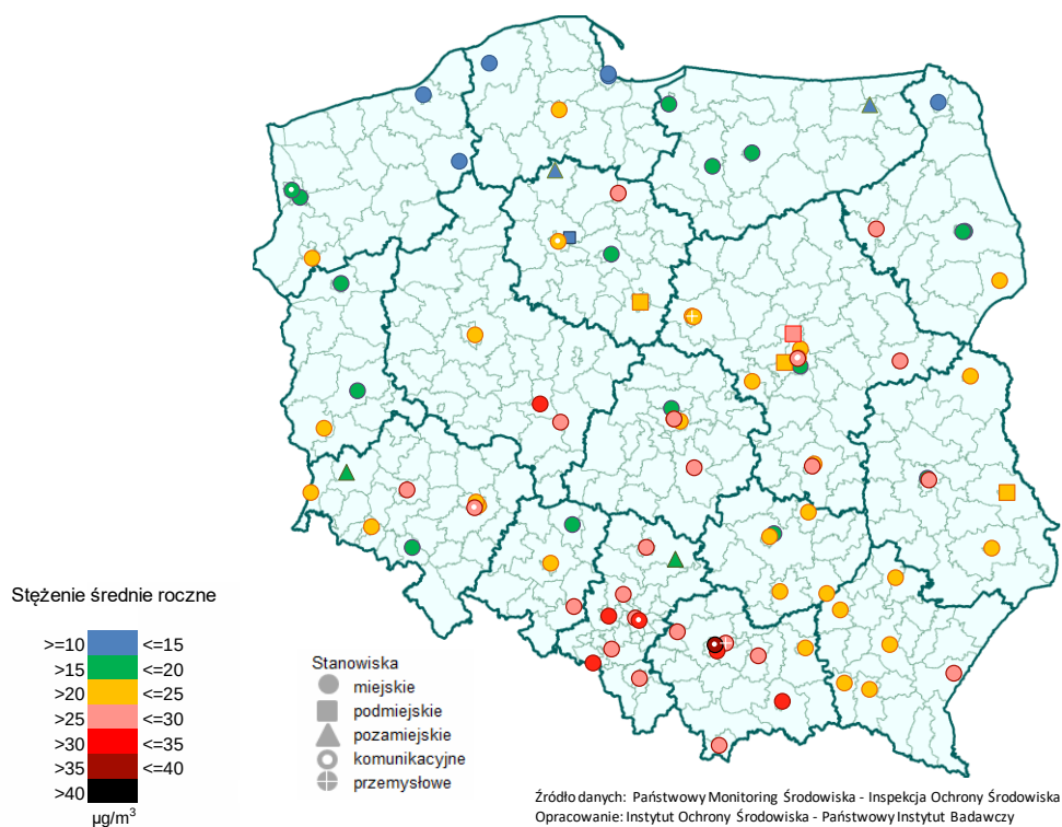
Rys. 6.4-1. Stężenia średnie roczne pyłu PM 2.5 w 2016 r.
