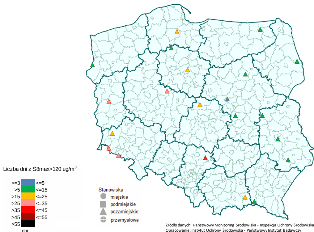
Rys. 4.4-3. Liczba dni z przekroczeniami wartości 120 \mu\text{g}/\text{m}^3 przez stężenia 8-godz. ozonu, uśredniona dla 1-3 lat, na stanowiskach pozamiejskich (dopuszczalna l. dni z przekroczeniami: 25)
