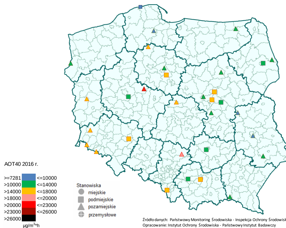
Rys. 4.5-3. Parametr AOT40 [ \mu\text{g}/\text{m}^3\cdot\text{h} ] obliczony dla okresu maj-lipiec 2016 r. dla stanowisk pozamiejskich i podmiejskich
