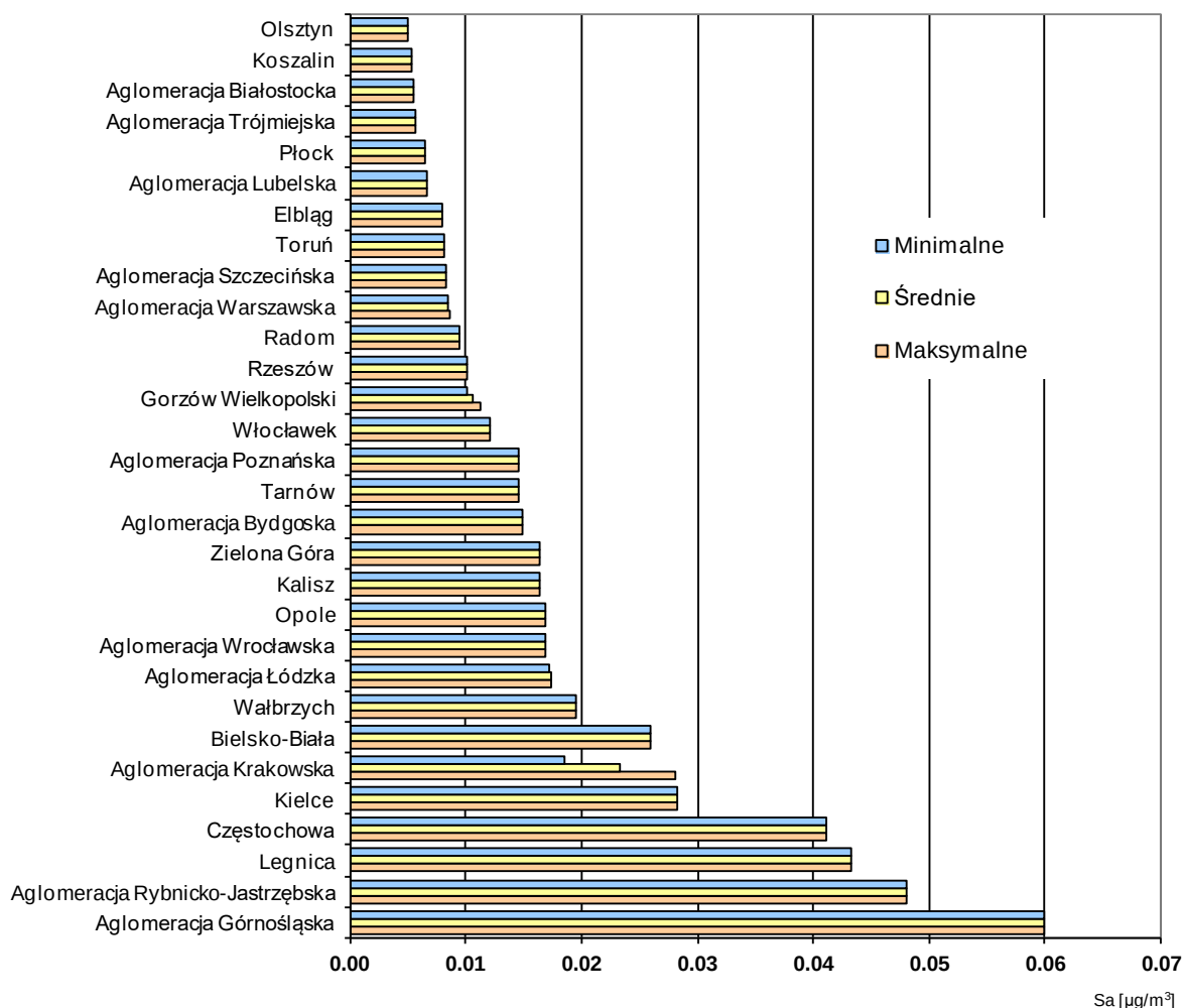
Rys. 3.7-1. Wartości średnich rocznych stężeń ołowiu (Pb) uzyskane w 2016 r. z pomiarów na terenie aglomeracji i miast powyżej 100 tys. mieszkańców
