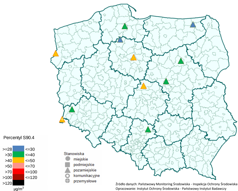
Rys. 5.4-5. Percentyl S90.4 z serii pomiarów 24-godz. stężeń pyłu PM10 w 2016 r. na stanowiskach pozamiejskich
