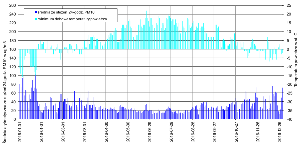
Rys. 5.2-8. Przebieg stężenia dobowego pyłu PM10 uśrednionego dla wszystkich stanowisk w Polsce w 2016 r. oraz minimum dobowe temperatury powietrza w Warszawie
