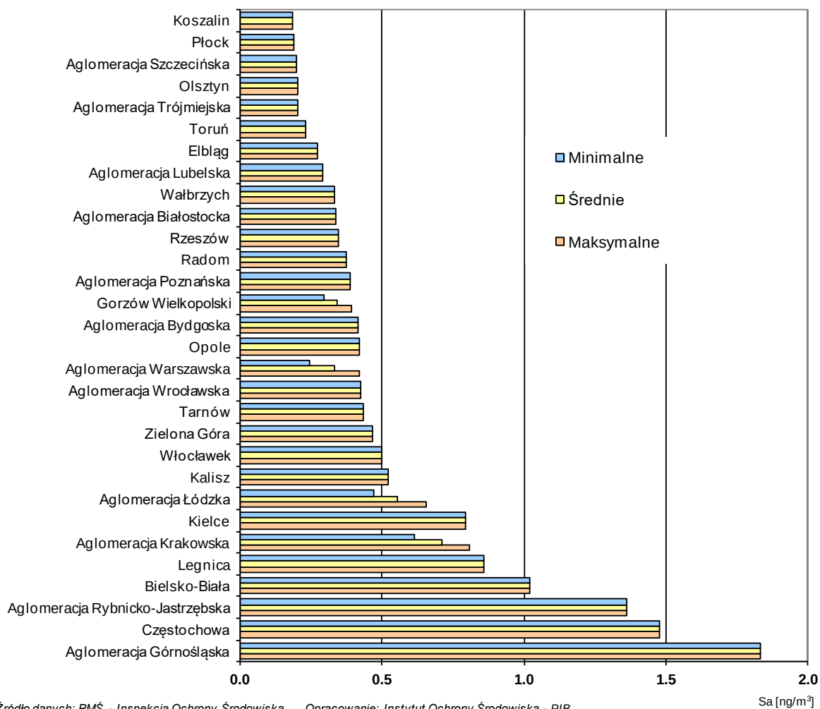
Rys. 3.9-1. Wartości średnich rocznych stężeń kadmu (Cd) uzyskane w 2016 r. z pomiarów na terenie aglomeracji i miast powyżej 100 tys. mieszkańców
