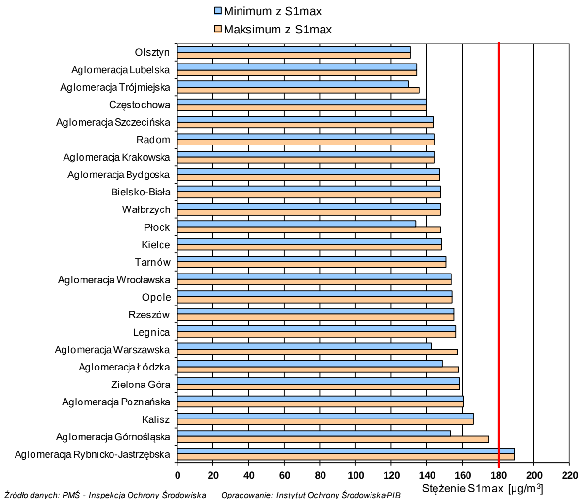
Rys. 3.5-3. Stężenia maksymalne 1-godz. ozonu uzyskane z pomiarów prowadzonych w 2016 r. na terenie aglomeracji i miast powyżej 100 tys. mieszkańców
