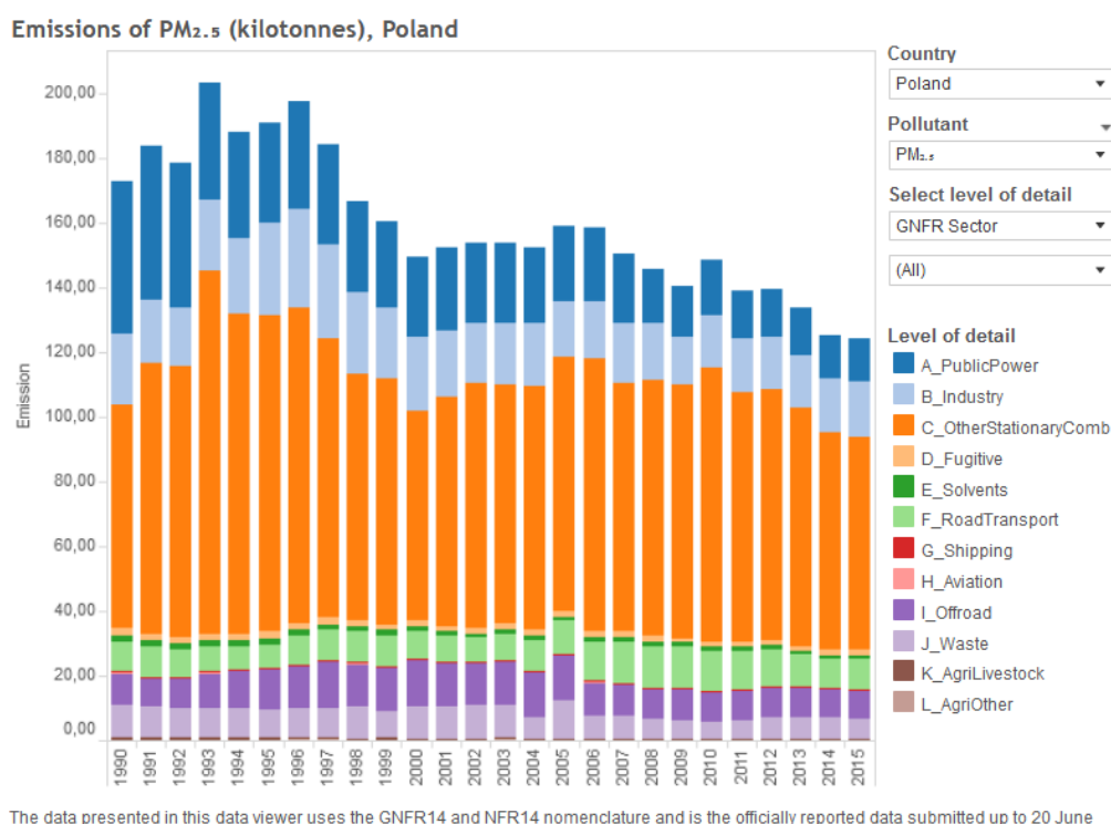
Rys. 6.5-2. Emisja pyłu PM 2.5 w Polsce w latach 1990-2015 r.
