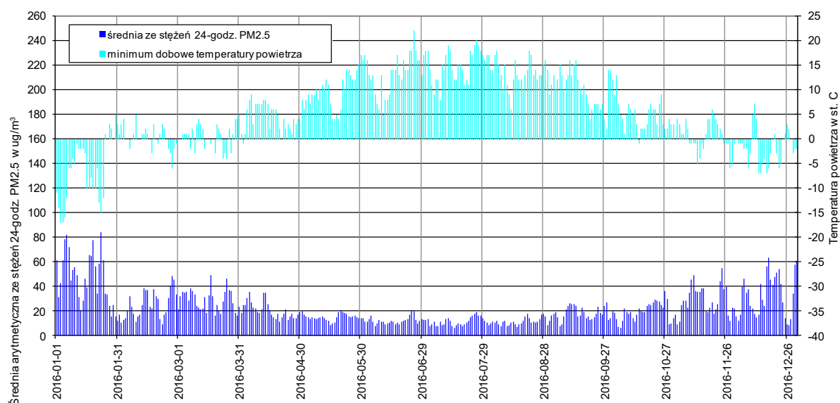
Rys. 6.2-3. Przebieg stężenia dobowego pyłu \text{PM}_{2.5} uśrednionego dla wszystkich stanowisk w Polsce w 2016 r. oraz minimum dobowe 1-godz. temperatury powietrza na stacji w Warszawie
