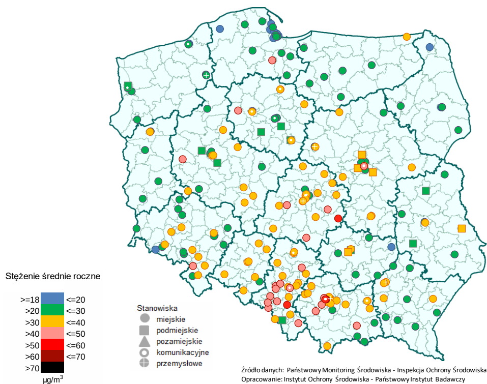
Rys. 5.4-1. Stężenia średnie roczne pyłu PM10 w 2016 r. na stanowiskach miejskich i podmiejskich
