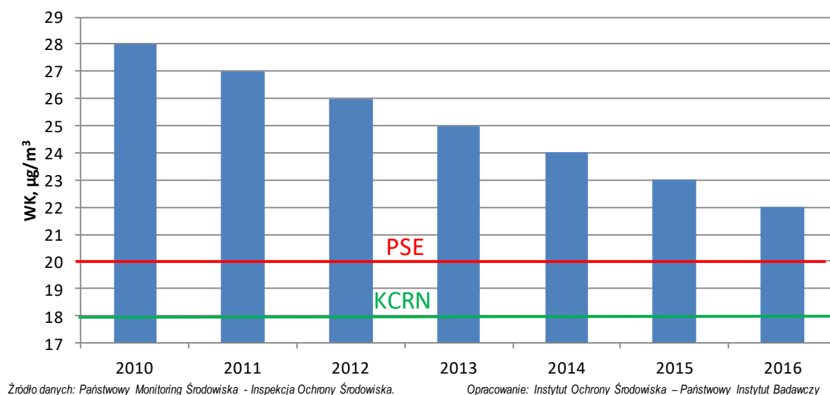
Rys. 3.12-4. Zmiany krajowego wskaźnika średniego narażenia PM 2.5 w latach 2010-2016 w odniesieniu do wartości pułapu stężenia ekspozycji (PSE=20 \mu\text{g}/\text{m}^3 ) oraz krajowego celu redukcji narażenia (KCRN=18 \mu\text{g}/\text{m}^3 )
