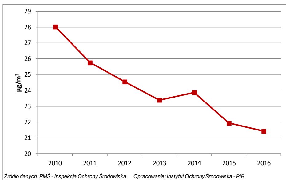
Rys. 3.12-3. Stężenie średnie roczne PM2.5 w latach 2010-2016, uśrednione dla zbioru 32 stanowisk znajdujących się na terenie aglomeracji i dużych miast, uwzględnianych przy obliczaniu wskaźnika średniego narażenia
