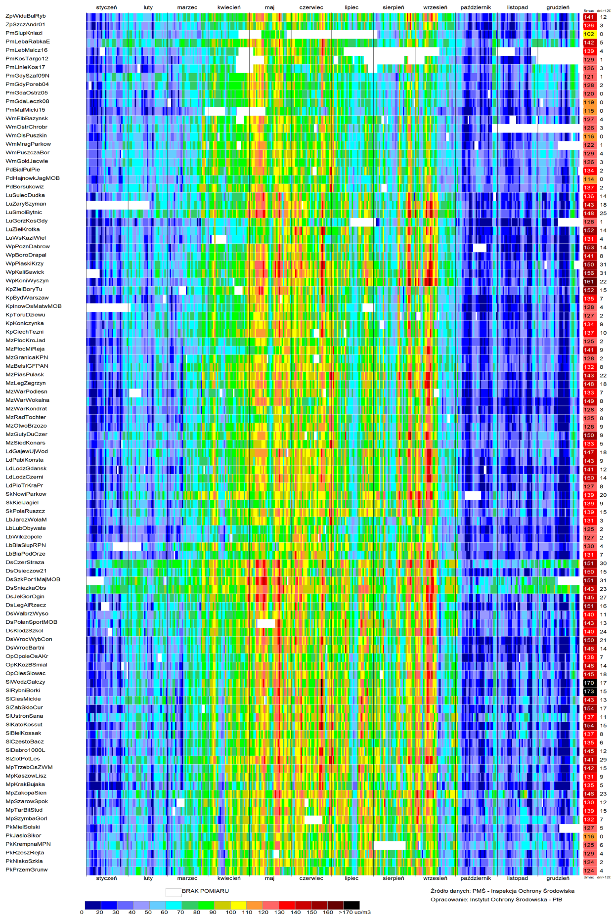
Rys. 4.2-5. Przebieg maksimów dziennych ze stężeń 8-godz. ozonu w 2016 na stanowiskach, z których wyniki wykorzystano w ocenie (dwie pierwsze litery w kodzie stanowisk to skrót nazwy województwa, np. Mz -mazowieckie, Mp - małopolskie itd.)
