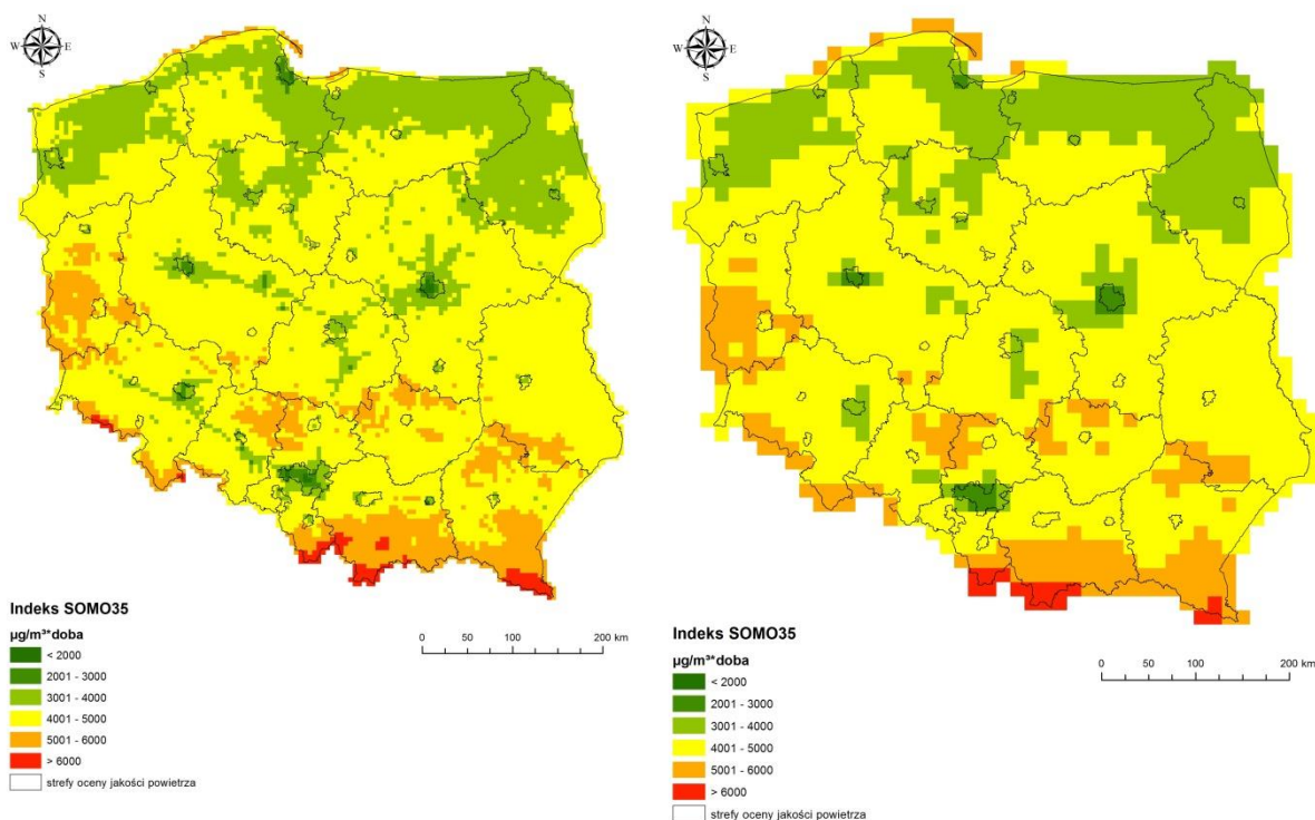
Rys. 4.2-16. Wartości parametru SOMO35 w 2016 r. oszacowana na podstawie wyników modelowania i pomiarów (w węzłach siatki kwadratów o boku 5 km – lewy rysunek i 15 km – prawy rysunek). Źródło: Wyniki modelowania stężeń ozonu troposferycznego na potrzeby rocznej oceny jakości powietrza dla roku 2016. Atmoterm 2017
