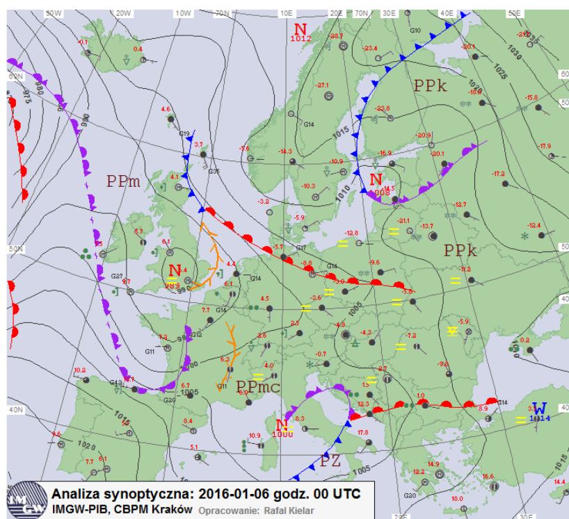
Rys. 5.2-11. Mapa synoptyczna na dzień 6.01.2016 g. 00 UTC. Źródło: IMGW-PIB
