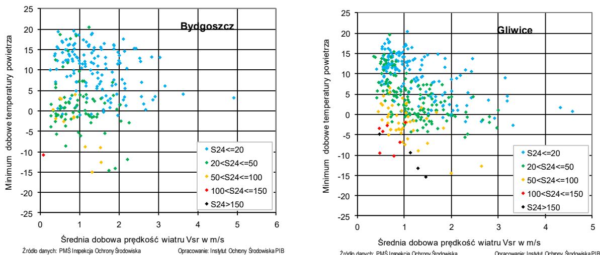
Rys. 6.2-8. Stężenia 24-godz. pyłu PM 2.5 w 2016 r. w zależności od średniej dobowej prędkości wiatru i minimum dobowego temperatury powietrza na stacjach w Bydgoszczy i Gliwicach
