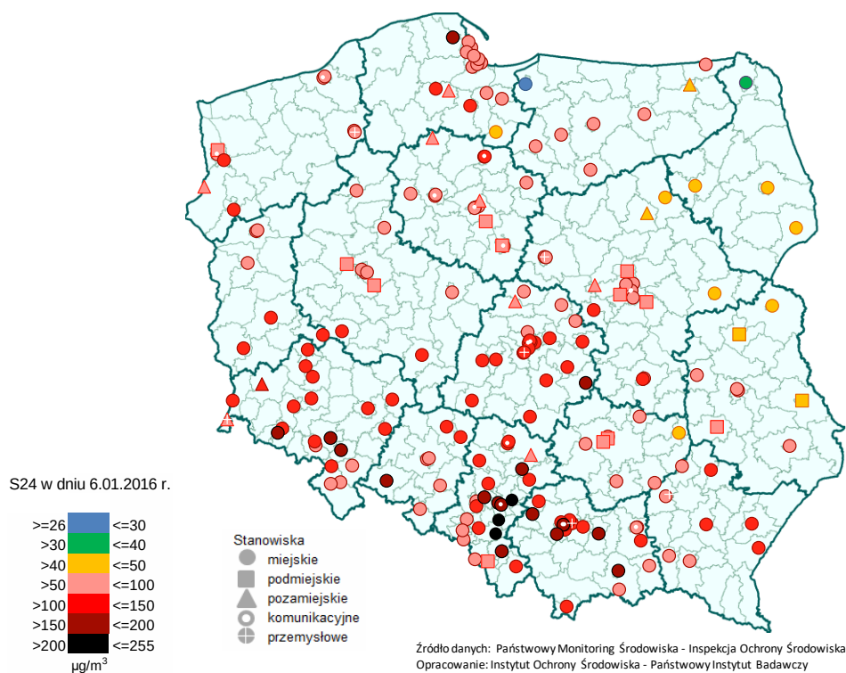
Rys. 5.2-10. Stężenia 24-godz. PM10 w dniu 6.01.2016 r.
