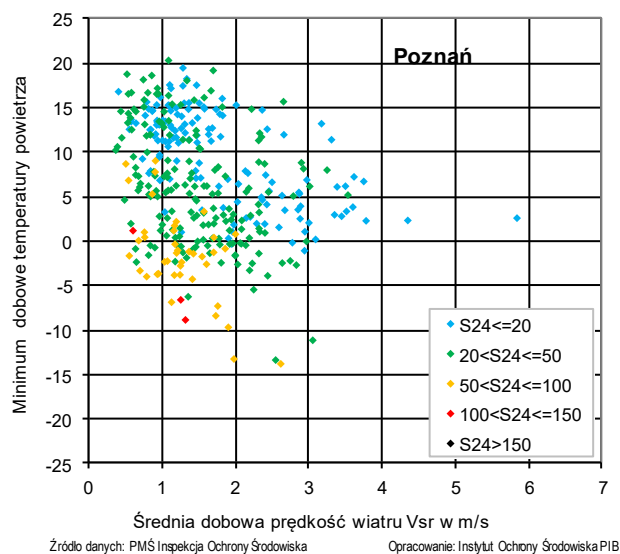
Rys. 5.2-13. Stężenia 24-godz. pyłu PM10 w 2016 r. w zależności od średniej dobowej prędkości wiatru i minimum dobowego temperatury powietrza na stacji Poznaniu (WpPoznDabrow)
