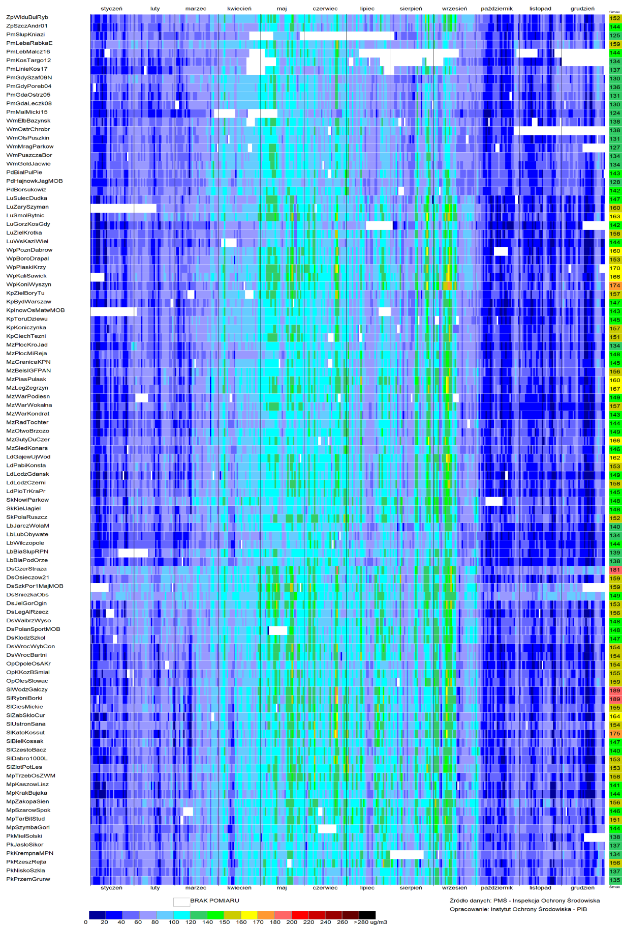
Rys. 4.2-11. Przebieg maksimów dziennych ze stężeń 1-godz. ozonu w 2016 na stanowiskach, z których wyniki wykorzystano w ocenie (dwie pierwsze litery w kodzie stanowisk to skrót nazwy województwa, np. Mz - mazowieckie, Mp - małopolskie itd.)
