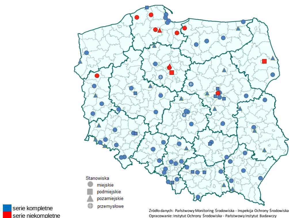
Rys. 4.1-1. Stanowiska pomiarowe stężeń ozonu, z których wyniki z 2016 r. wykorzystano w opracowaniu
