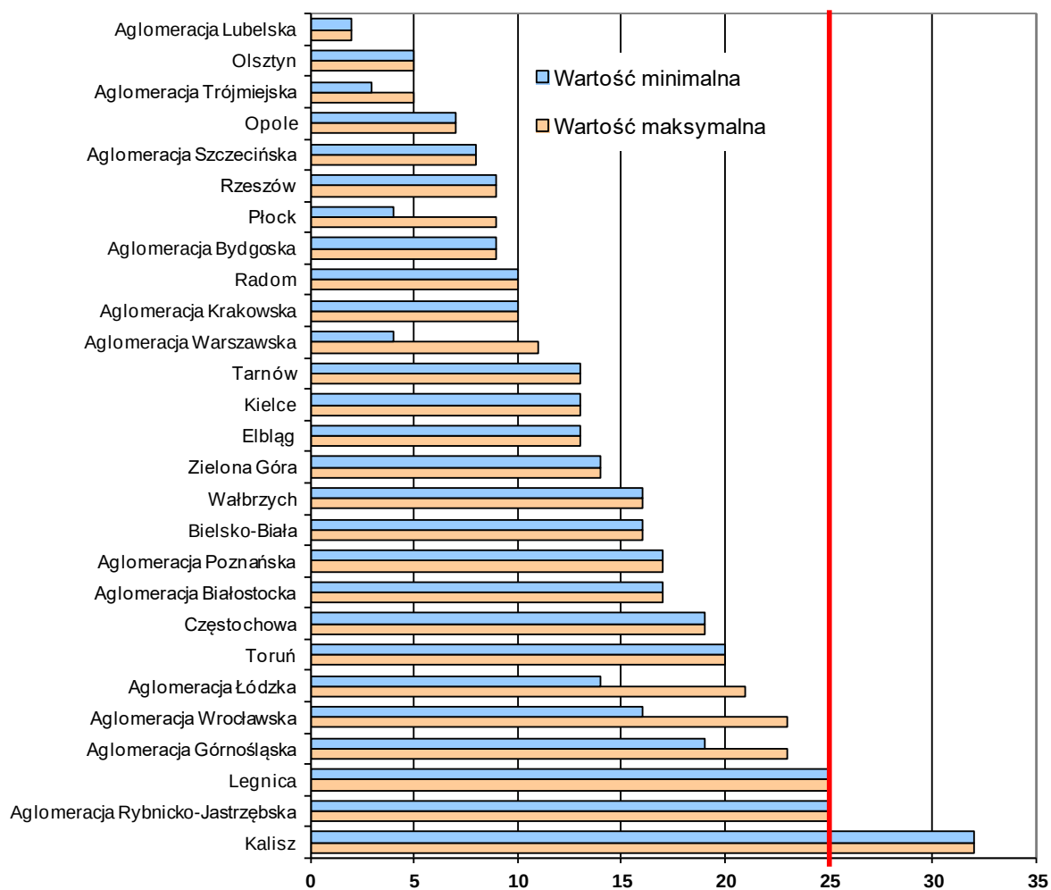
Rys. 3.5-2. Liczba dni w roku z przekroczeniami poziomu docelowego 120 \mu\text{g}/\text{m}^3 przez stężenia 8-godz. krocząco ozonu uśredniona dla 1-3 lat (z okresu 2014-2016), określona na podstawie pomiarów na terenie aglomeracji i miast powyżej 100 tys. mieszkańców
