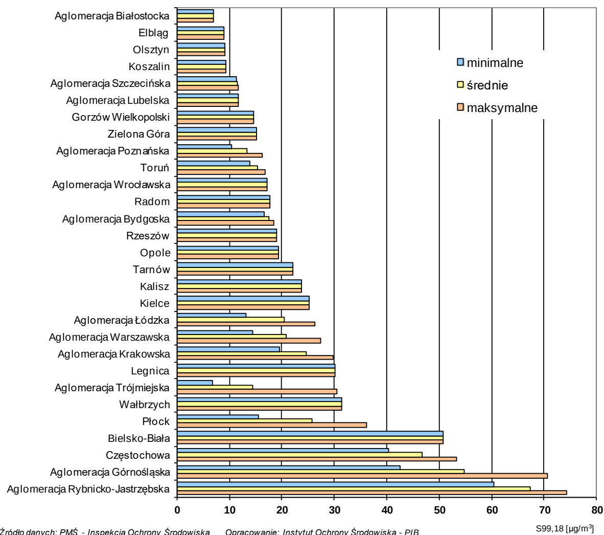
Rys. 3.1-1. Wartości percentyla S99.18 ze stężeń 24-godzinnych SO 2 uzyskane z pomiarów prowadzonych w 2016 r. na terenie aglomeracji i miast powyżej 100 tys. mieszkańców
