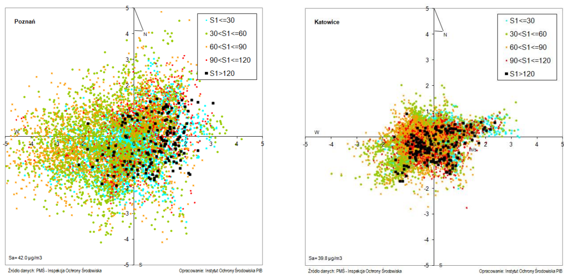
Rys. 4.2-12. Stężenia 1-godz. ozonu w 2016 r. w zależności od prędkości i kierunku wiatru na stacjach w Poznaniu i Katowicach
