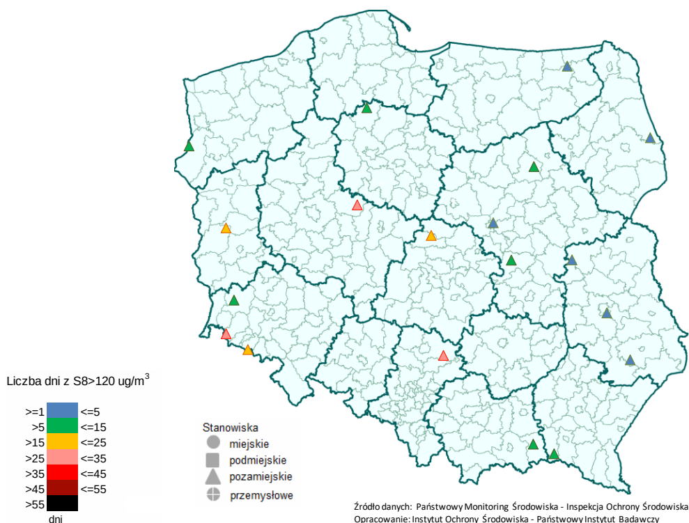
Rys. 4.4-5. Liczba dni z przekroczeniami wartości 120 \mu\text{g}/\text{m}^3 przez stężenia 8-godz. ozonu w 2016 r. na stanowiskach pozamiejskich
