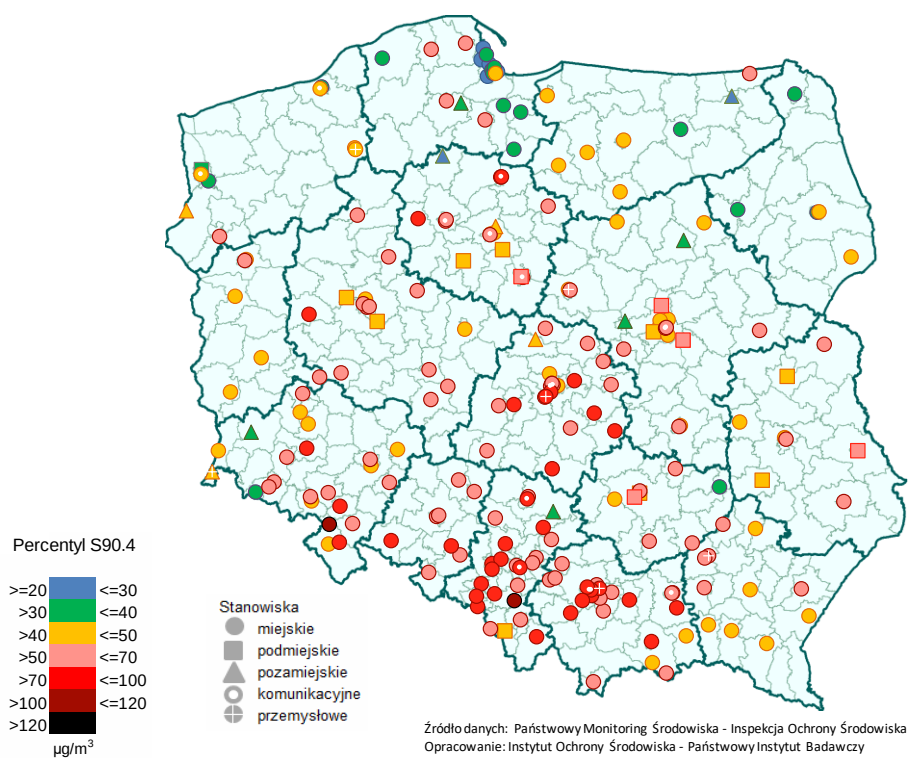
Rys. 5.2-3. Percentyl S90.4 z serii stężeń 24-godz. pyłu PM10 w 2016 r.
