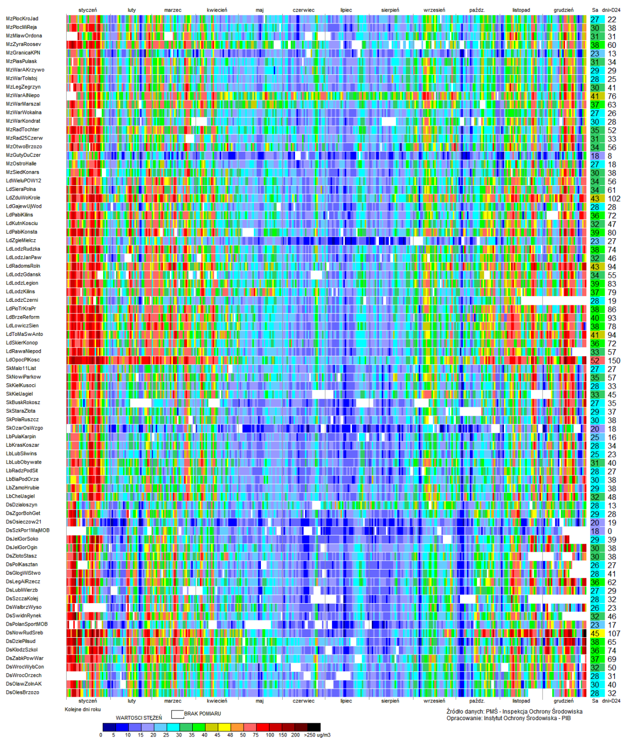
Rys. 5.2-7-B. Przebieg stężeń 24-godz. pyłu PM10 w 2016 r. na stanowiskach, z których wyniki wykorzystano w ocenie (dwie pierwsze litery w kodzie stanowisk to skrót nazwy województwa, na obszarze którego zlokalizowane jest stanowisko, np. Mz - mazowieckie, Ds - dolnośląskie itd.)
