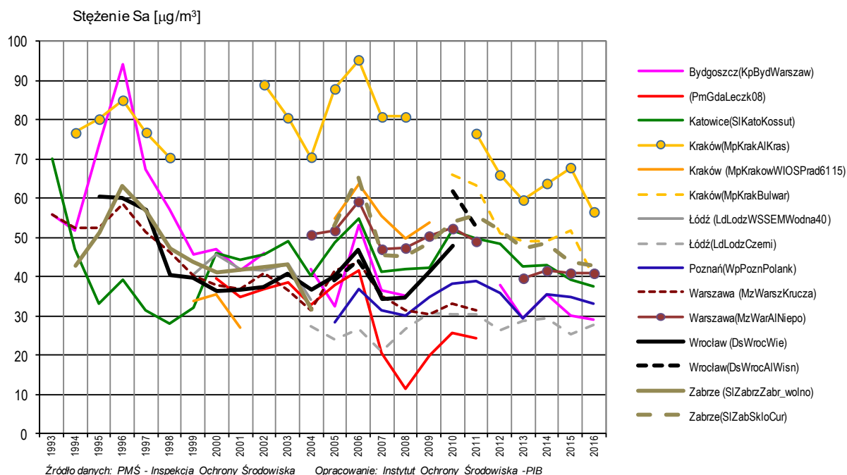
Rys. 3.6-4. Stężenie średnie roczne pyłu PM10 w latach 1993-2016 na wybranych stanowiskach w aglomeracjach w Polsce (linie z kropkami oznaczają stanowiska „komunikacyjne”)
