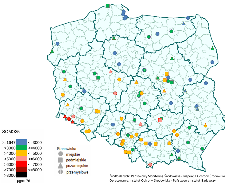
Rys. 4.2-15. Wartości parametru SOMO35 w 2016 r. na stanowiskach pomiarowych
