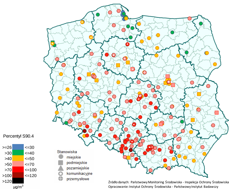
Rys. 5.4-2. Percentyl S90.4 z serii pomiarów 24-godz. stężeń pyłu PM10 w 2016 r. na stanowiskach miejskich i podmiejskich
