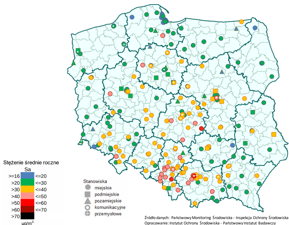
Rys. 5.2-1. Stężenia średnie roczne pyłu PM 10 w 2016 r.
