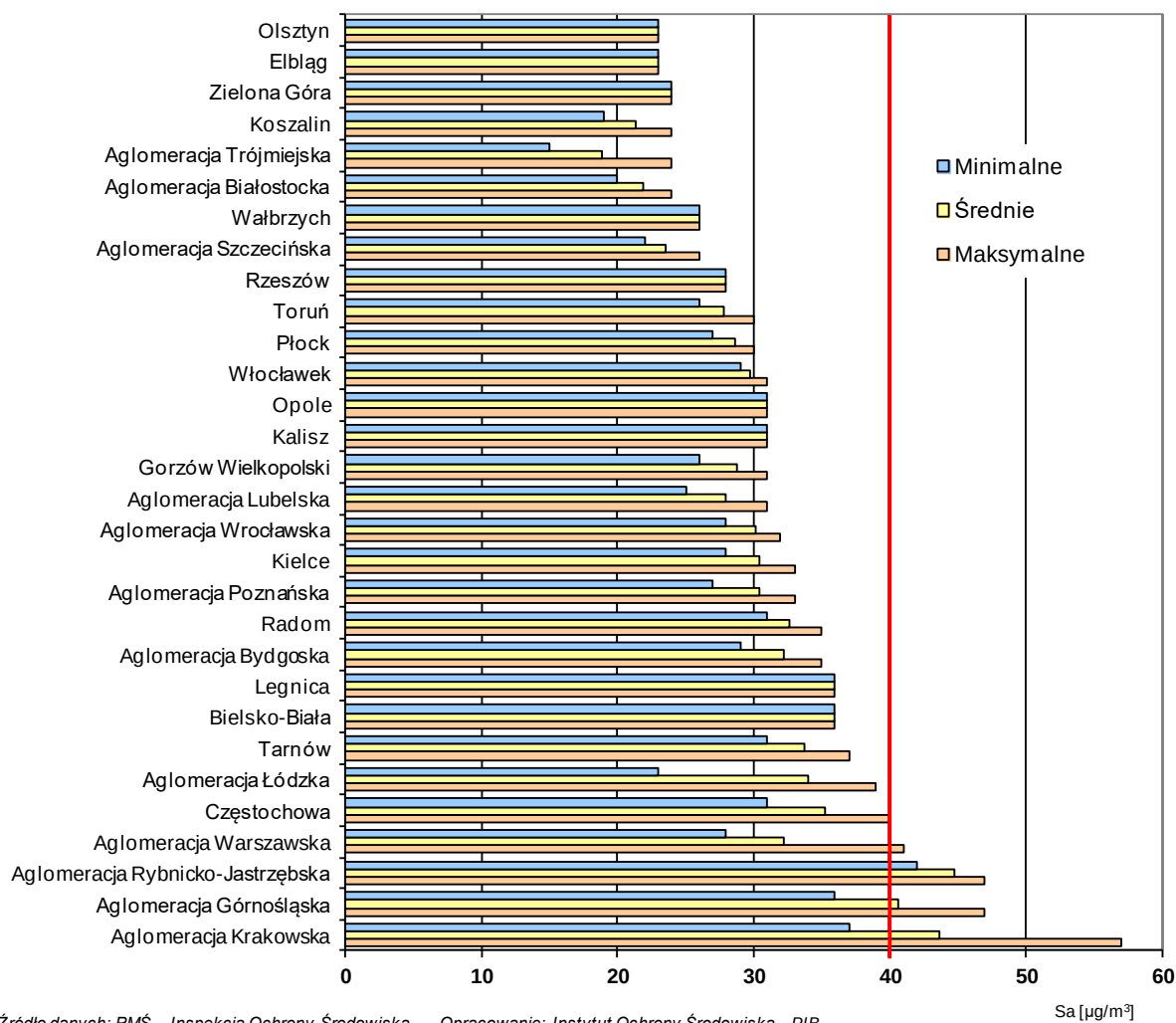
Rys. 3.6-1. Średnie roczne stężenia pyłu PM10 uzyskane z pomiarów prowadzonych w 2016 r. na terenie aglomeracji i miast powyżej 100 tys. mieszkańców
