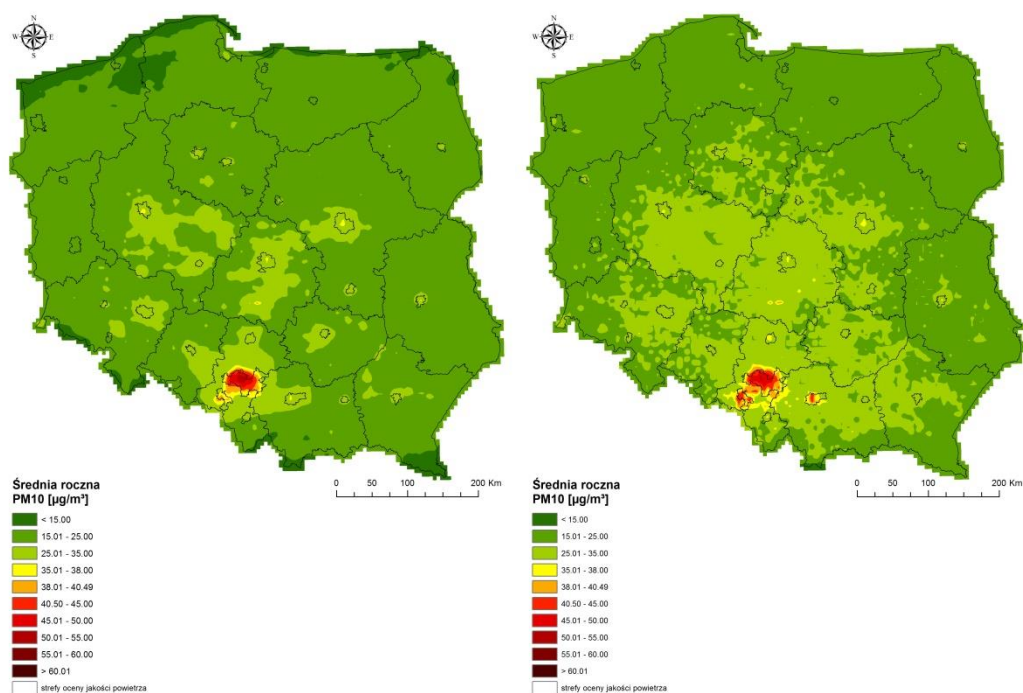
Rys. 5.2-2. Rozkład stężeń średniorocznych pyłu PM 10 w skali kraju - wynik modelowania CAMx w wariancie I (modelowanie) i II (połączenie modelowania i wyników pomiarów stężeń)
