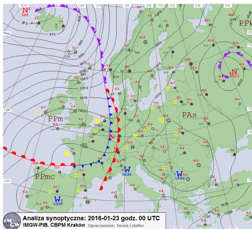
Rys. 6.2-6. Mapa synoptyczna na dzień 23.01.2016 g. 00 UTC. Źródło: IMGW-PIB
