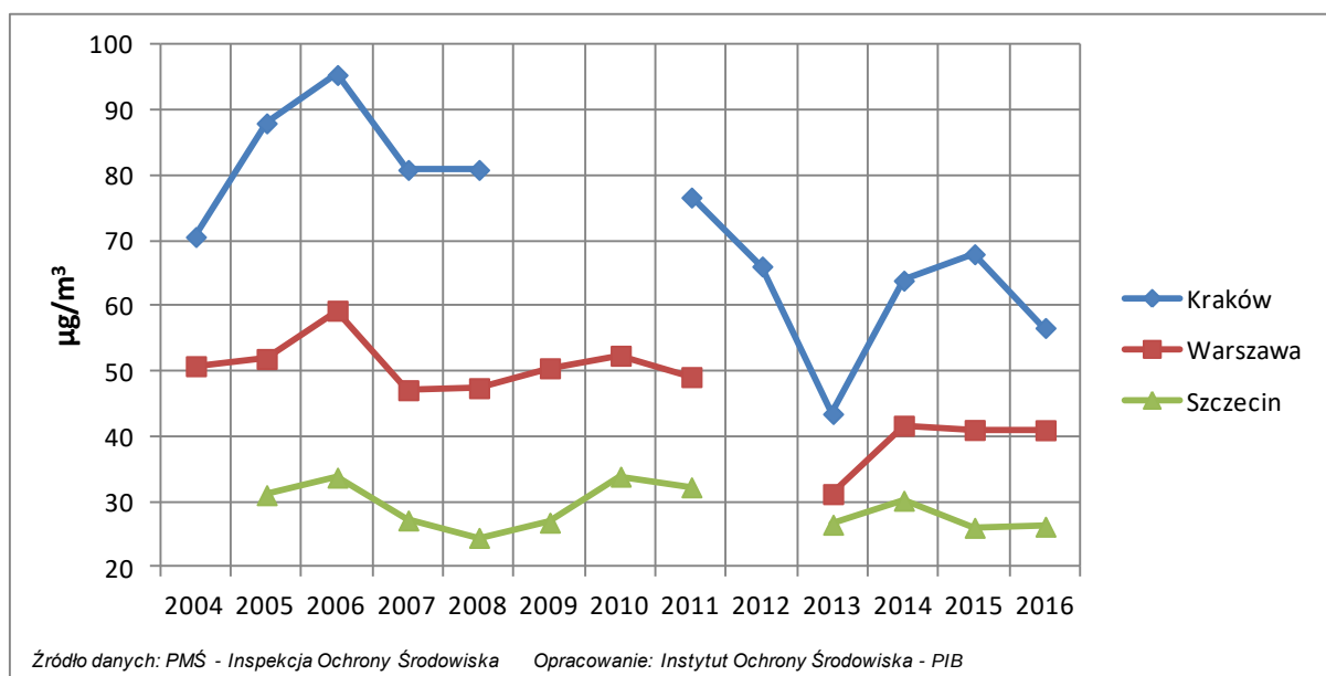
Rys. 5.3-2. Stężenia średnie roczne PM10 w latach 2004-2016 na stanowiskach komunikacyjnych w Krakowie, w Warszawie i w Szczecinie
