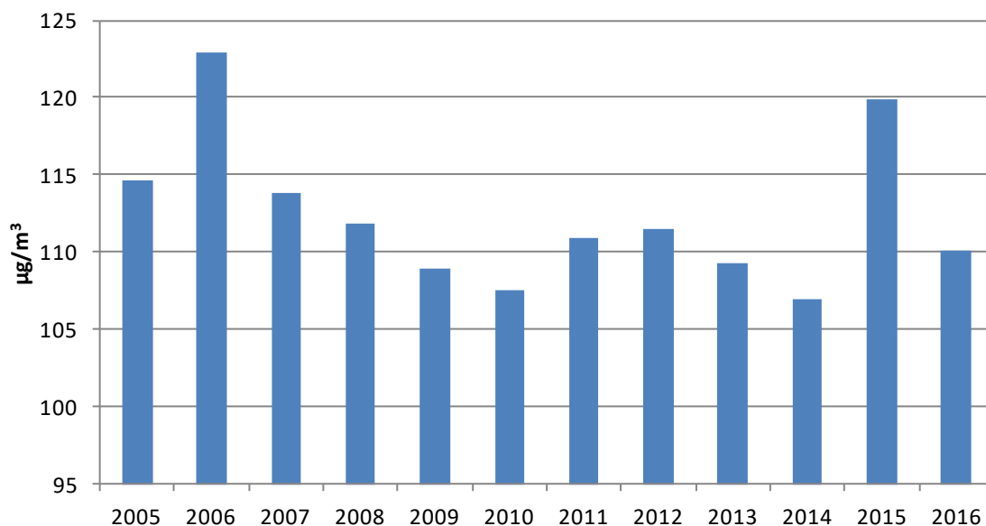
Rys. 4.3-2. Uśredniona dla wszystkich stanowisk uwzględnionych w analizach (z kompletnymi seriami pomiarowymi) wartości percentyla S93.2 z rocznych serii maksimów dobowych stężeń 8-godz. kroczących ozonu w latach 2005-2016
