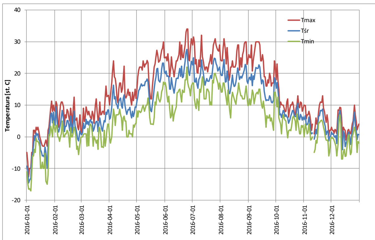
Rys. 4.2-4. Temperatura średnia dobową, maksymalna i minimalna na stacji IMGW-PIB Warszawa Okęcie. Źródło: http://www7.ncdc.noaa.gov/CDO/cdoselect.cmd?datasetabbv=GSOD&countryabbv=&georegionabbv=&resolution=40
