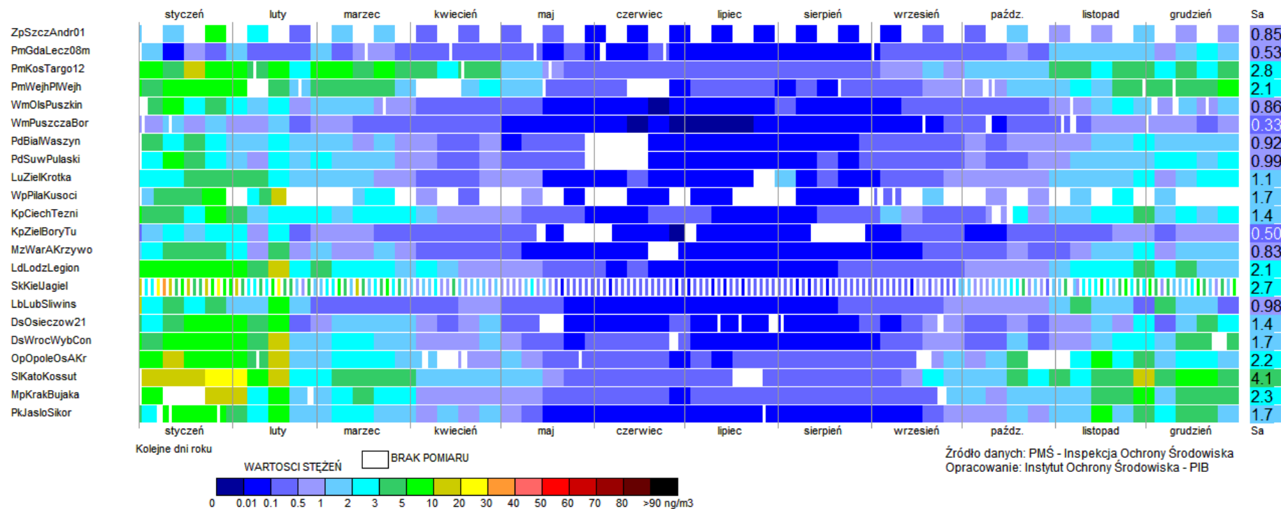
Rys. 4.5-2. Przebieg stężeń benzo(k)fluorantenu (B(k)F) w 2017 r. oraz stężenie średnie roczne Sa na stanowiskach, z których wyniki wykorzystano w ocenie (dwie pierwsze litery w kodzie stanowisk to skrót nazwy województwa, na obszarze którego zlokalizowane jest stanowisko, np. Pm - pomorskie, Kp – kujawsko-pomorskie itd.)
