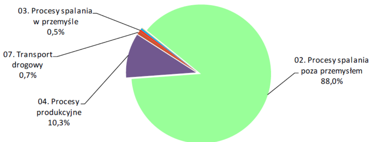
Rys. 2-1. Udział największych sektorów w emisji WWA w Polsce w roku 2016
