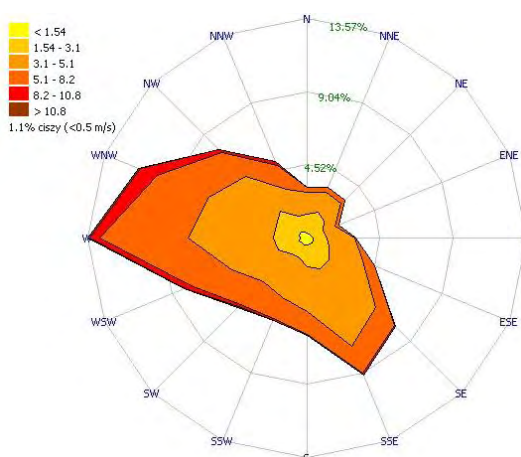
Mapa Z5.2. Róża wiatrów w oczku siatki odpowiadającym położeniu stacji Warszawa-Targówek
