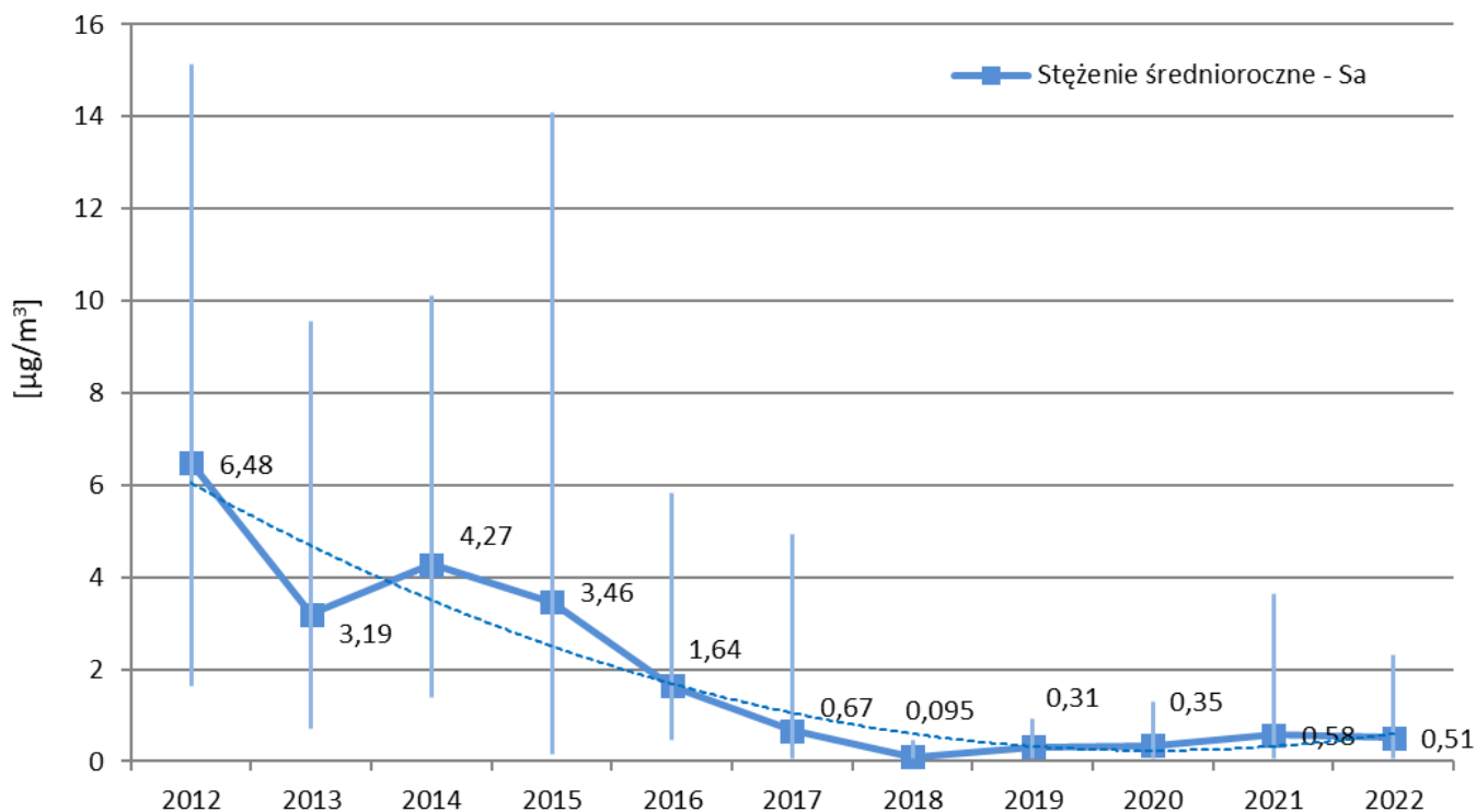
Rys. 1. Stężenia średnioroczne formaldehydu pomierzone w latach 2012-2022 na stacji w Żarach, przy ul. Szymanowskiego, wraz ze stężeniami dobowymi minimalnymi i maksymalnymi w danym roku
