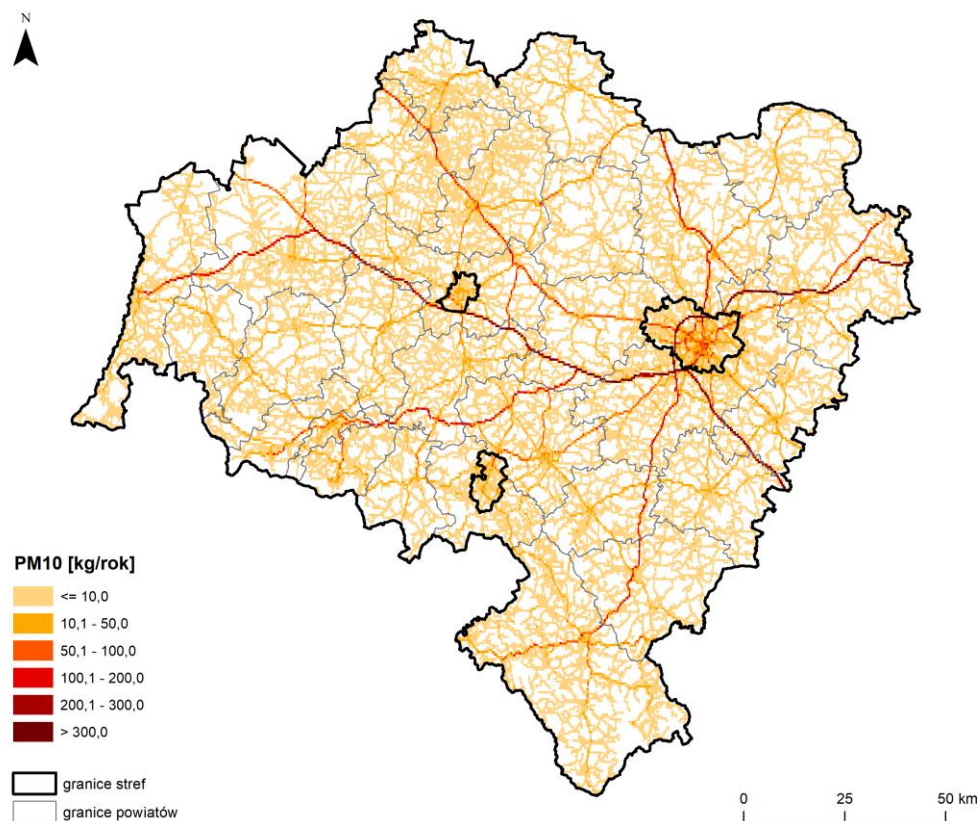
Rysunek 6.6. Lokalizacja liniowych źródeł emisji pyłu PM10 na obszarze województwa dolnośląskiego [opracowanie własne, źródło danych: KOBIZE / IOŚ-PIB]
