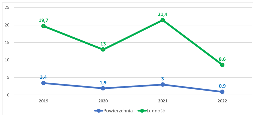
Rys. 3.6.12. Procentowy udział obszaru przekroczenia oszacowanego dla poziomu dopuszczalnego dotyczącego wartości średnich 24-godzinnych stężenia pyłu zawieszonego PM10 w skali Polski w latach 2019 - 2022
