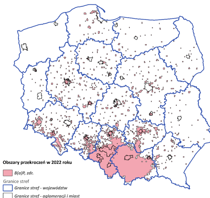
Rys. 3.11.8. Zasięg obszaru przekroczenia oszacowanego dla średniego rocznego stężenia benzo(a)pirenu w pyłe zawieszonym PM10 na obszarze Polski w 2022 roku
