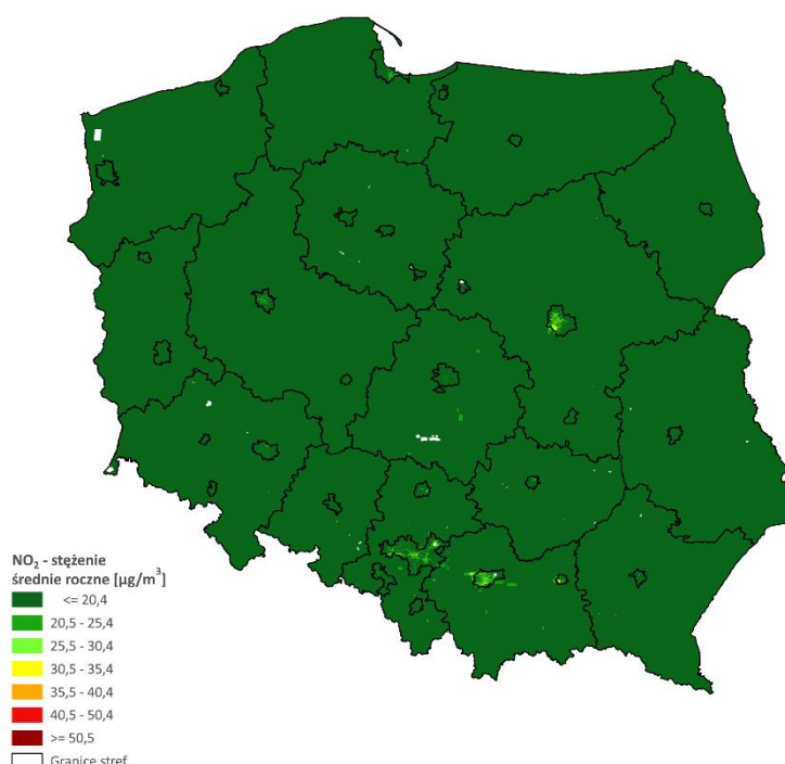
Rys. 3.2.10. Rozkład przestrzenny średniego rocznego stężenia \text{NO}_2 na obszarze Polski w 2022 roku, określony na podstawie modelowania matematycznego oraz obiektywnego szacowania
