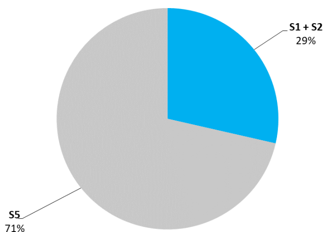
Rys. 3.6.13. Przyczyny wystąpienia sytuacji przekroczeń dopuszczalnego poziomu 24-godz. stężeń pyłu zawieszonego PM 10 w strefach zaliczonych do klasy C w 2022 roku, wskazane jako główne dla poszczególnych przypadków przekroczeń – udział procentowy w skali kraju
