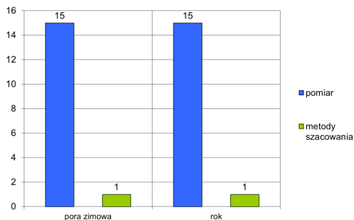
Rys. 4.1.2. Liczba stref, w których jako podstawę rocznej oceny dla SO 2 (określenie klasy wg parametrów, ochrona roślin) w 2022 r. wskazano określone metody
