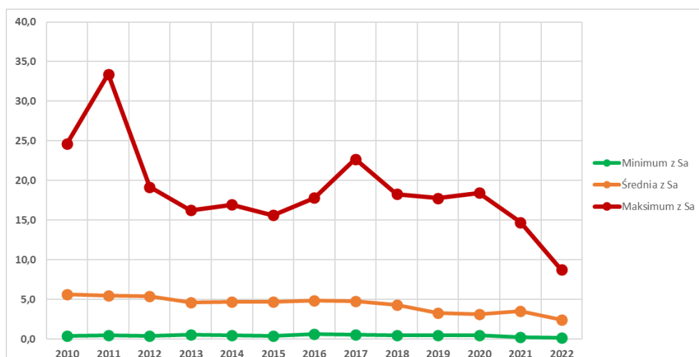
Rys. 3.13.5. Wartości maksymalne, średnie i minimalne z mierzonych w Polsce średnich rocznych stężeń benzo(a)pirenu w latach 2010 – 2022 [ \text{ng/m}^3 ]
