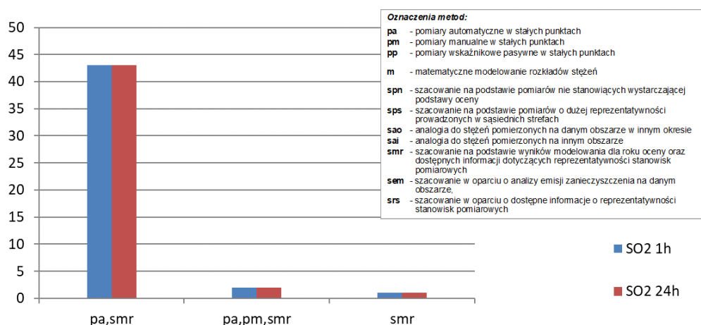
Rys. 3.1.6. Liczba stref, w których na potrzeby rocznej oceny dotyczącej SO 2 (stężenia 1-godz. i 24-godz., ochrona zdrowia) w 2022 r. wykorzystano określone połączenie metod szczegółowych
