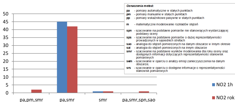
Rys. 3.2.8. Liczba stref, w których na potrzeby oceny dotyczącej NO 2 , (stężenia 1-godz. i średnie roczne, ochrona zdrowia) za 2022 rok wykorzystano wskazane szczegółowe metody oceny
