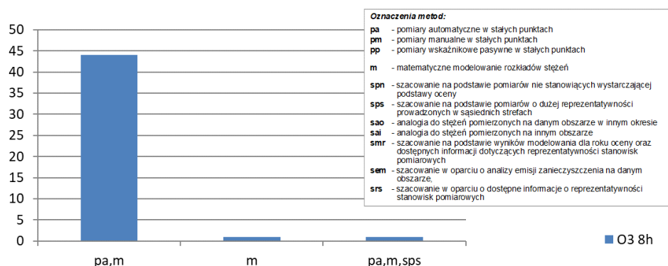
Rys. 3.5.5. Liczba stref, w których na potrzeby oceny dotyczącej O 3 (ochrona zdrowia) za 2022 rok wykorzystano wskazane szczegółowe metody oceny
