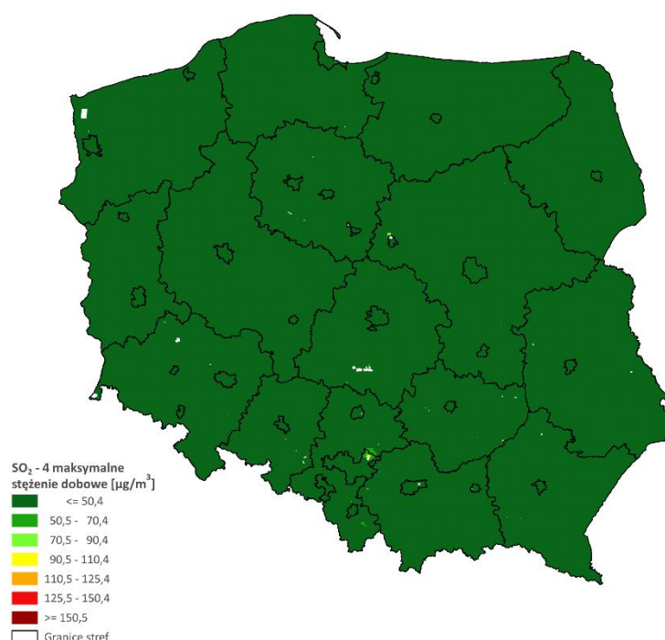
Rys. 3.1.8. Rozkład przestrzenny stężenia \text{SO}_2 na obszarze Polski w 2022 roku, wyrażony jako 4-te maksymalne stężenie średnie dobowe, określony na podstawie modelowania matematycznego oraz obiektywnego szacowania
