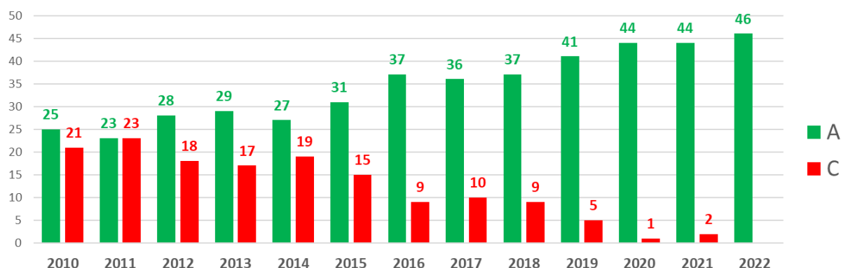
Rys. 3.6.4. Liczba stref z klasą A oraz C, określona na podstawie średnich rocznych stężeń pyłu zawieszonego PM10 w wyniku ocen jakości powietrza za lata 2010 - 2022 (ochrona zdrowia)
