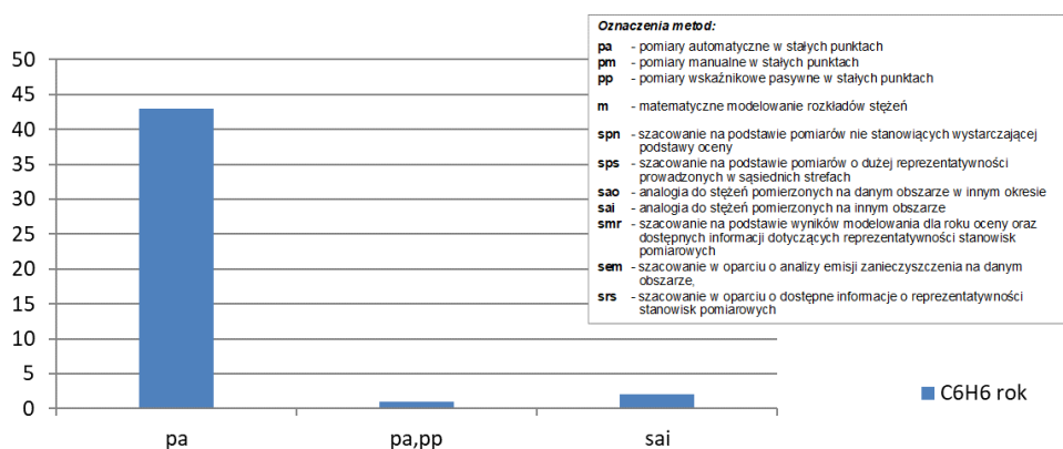
Rys. 3.4.4. Liczba stref, w których na potrzeby oceny dotyczącej C 6 H 6 (ochrona zdrowia) za 2022 rok wykorzystano wskazane szczegółowe metody oceny
