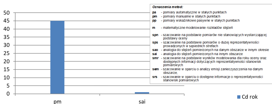
Rys. 3.9.4. Liczba stref, w których na potrzeby oceny dotyczącej Cd w pyłe zawieszonym PM10 (ochrona zdrowia) za 2022 rok wykorzystano wskazane szczegółowe metody oceny
