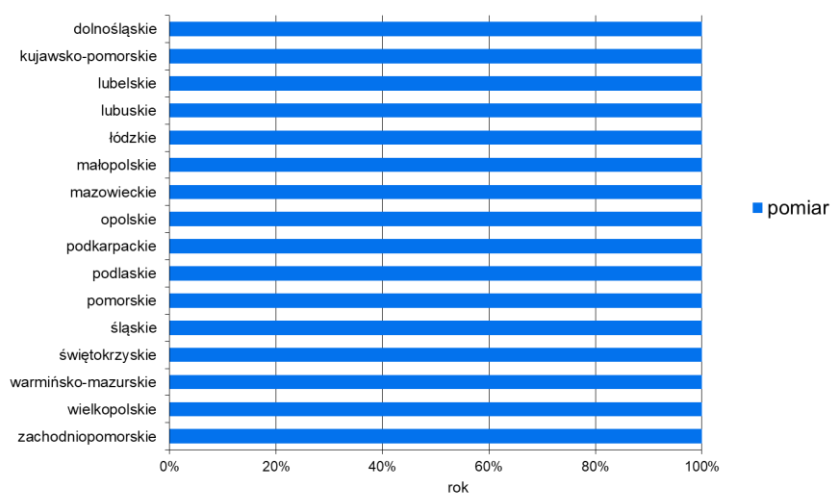
Rys. 3.12.7. Procent stref, w poszczególnych województwach, w których jako podstawę rocznej oceny dla pyłu zawieszonego PM 2,5 (ochrona zdrowia) w 2022 r. wskazano określone metody
