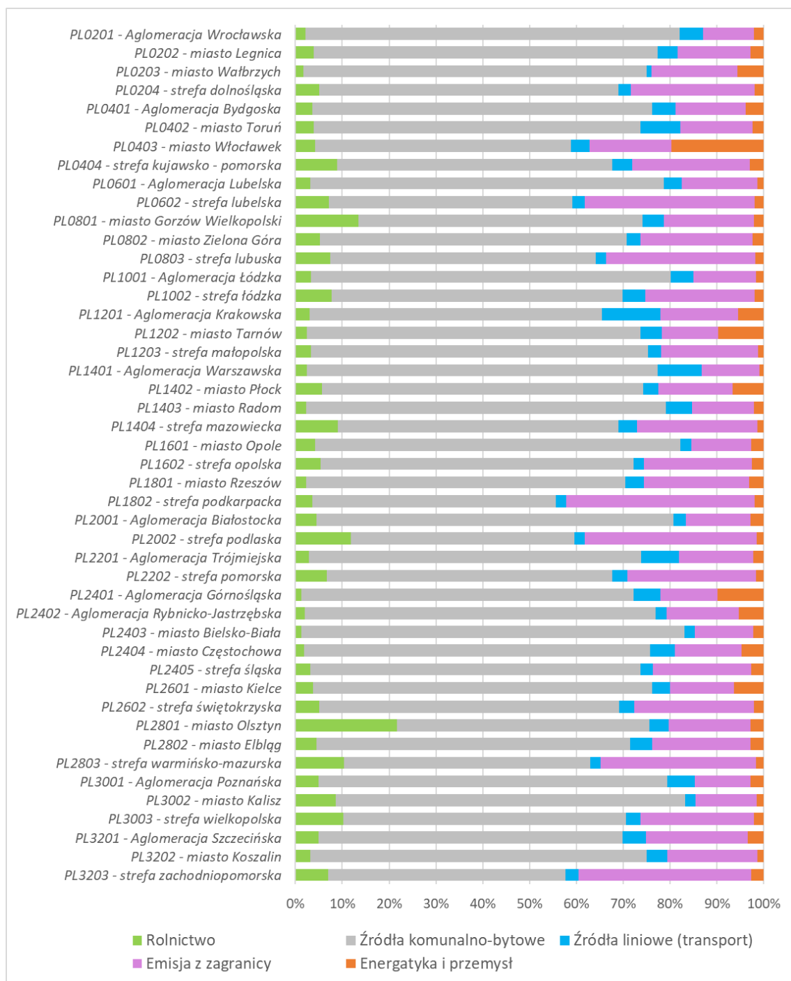
Rys. 3.6.15. Uśredniony udział źródeł emisji w stężeniu pyłu zawieszonego PM10 w poszczególnych strefach w Polsce w 2022 roku (dla ocenianego parametru związanego ze stężeniami średnimi 24-godzinnymi) oszacowany na podstawie modelowania
