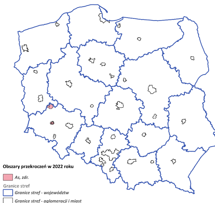
Rys. 3.8.6. Zasięg obszaru przekroczenia oszacowanego dla średniego rocznego stężenia arsenu w pyłe zawieszonym PM10 na obszarze Polski w 2022 roku
