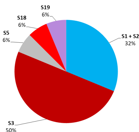
Rys. 3.12.13. Przyczyny przekroczeń II fazy dopuszczalnego poziomu pyłu zawieszonego PM 2,5 w powietrzu (stężenia średniego rocznego) w strefach zaliczonych do klasy C w 2022 roku, wskazane jako dodatkowe – udział procentowy w skali kraju
