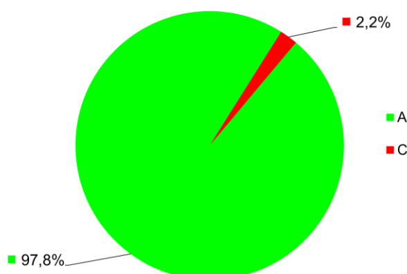
Rys. 3.12.6. Procent stref zaliczonych do określonych klas dla pyłu zawieszonego PM 2,5 (klasa strefy, ochrona zdrowia) w Polsce w 2022 r.
