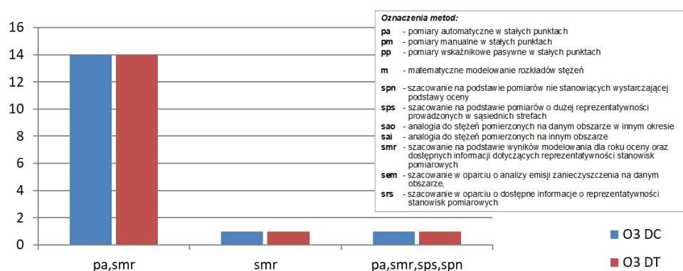
Rys. 4.3.4. Liczba stref, w których na potrzeby oceny dotyczącej O 3 (ochrona roślin, DC - poziom docelowy; DT - poziom celu długoterminowego) za 2022 rok wykorzystano wskazane szczegółowe metody oceny
