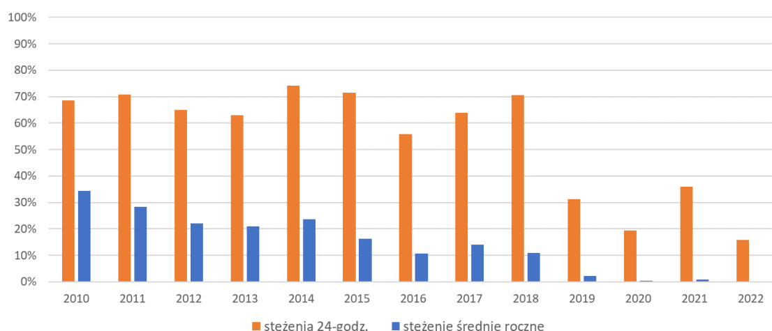
Rys. 3.13.3. Udział stanowisk pomiarowych na których wystąpiło przekroczenie poziomu dopuszczalnego pyłu zawieszonego PM 10 w ogólnej liczbie stanowisk uwzględnionych w ocenie w latach 2010-2022
