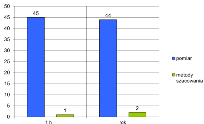
Rys. 3.2.5. Liczba stref, w których jako podstawę rocznej oceny dla NO 2 (stężenia 1-godz. i średnie roczne, ochrona zdrowia) w 2022 r. wskazano określone metody
