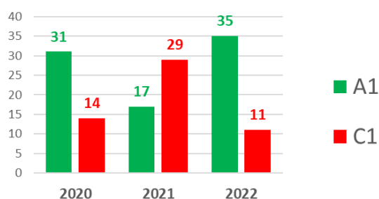
Rys. 3.12.2. Liczba stref z klasą A1 oraz C1, określona na podstawie średnich rocznych stężeń pyłu zawieszonego PM 2,5 w wyniku ocen jakości powietrza za lata 2020 - 2022 (poziom dopuszczalny II faza, ochrona zdrowia)
