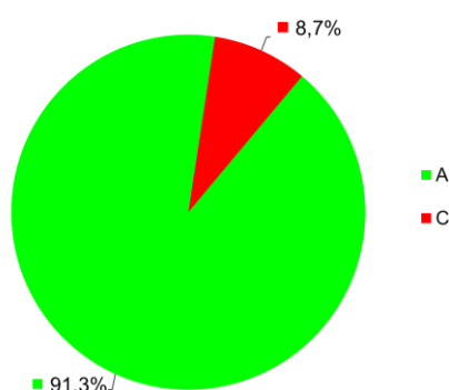
Rys. 3.2.4. Procent stref zaliczonych do określonych klas dla NO 2 (klasa strefy, ochrona zdrowia) w Polsce w 2022 r.
