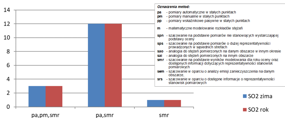
Rys. 4.1.3. Liczba stref, w których na potrzeby oceny dotyczącej SO 2 (określenie klasy wg parametrów, ochrona roślin) za 2022 rok wykorzystano wskazane szczegółowe metody oceny
