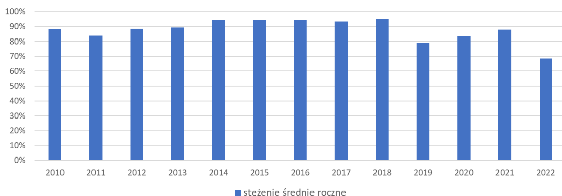
Rys. 3.13.4. Udział stanowisk pomiarowych na których wystąpiło przekroczenie poziomu docelowego stężenia benzo(a)pirenu zawartego w pyłe zawieszonym PM 10 w ogólnej liczbie stanowisk uwzględnionych w ocenie w latach 2010-2022
