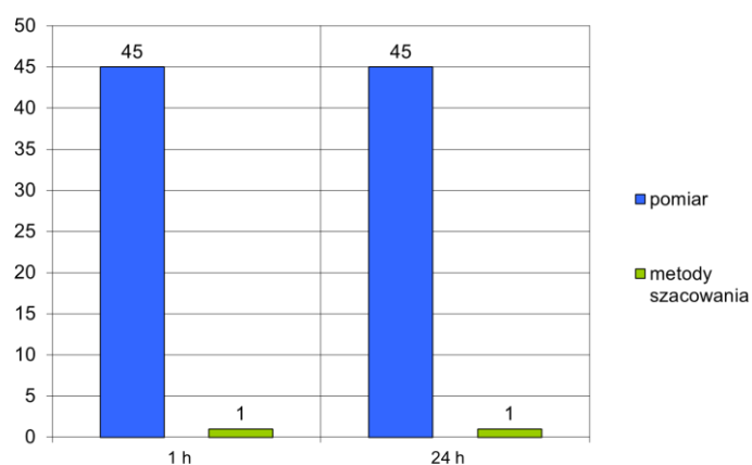
Rys. 3.1.4. Liczba stref, w których jako podstawę rocznej oceny dla SO 2 (stężenia 1-godz. i 24-godz., ochrona zdrowia) w 2022 r. wskazano określone metody
