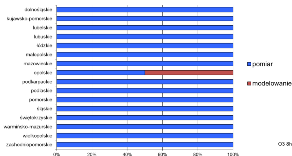
Rys. 3.5.4. Udział określonych metod przyjętych w poszczególnych województwach jako podstawa oceny za 2022 r. dla O 3 (ochrona zdrowia)
