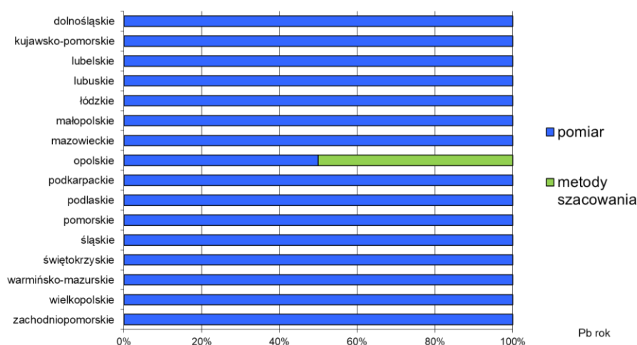
Rys. 3.7.3. Procent stref, w poszczególnych województwach, w których jako podstawę rocznej oceny dla Pb w pyłe zawieszonym PM10 (stężenia średnie roczne, ochrona zdrowia) w 2022 r. wskazano określone metody
