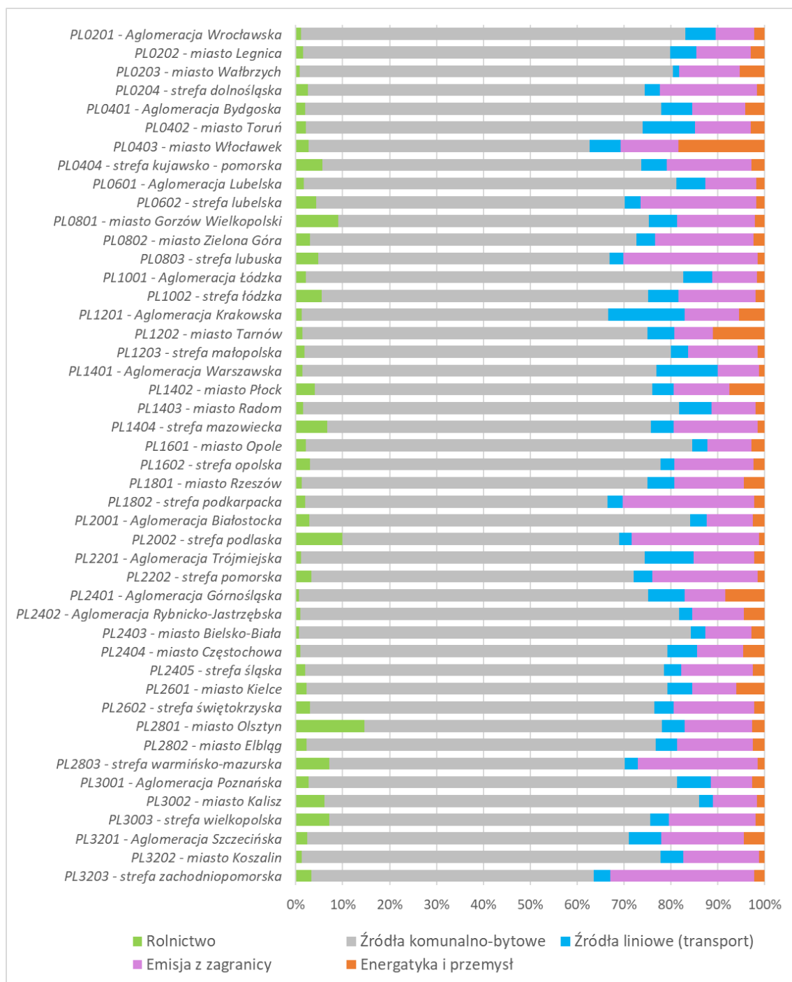
Rys. 3.12.14. Uśredniony udział źródeł emisji w stężeniu pyłu zawieszonego PM 2,5 w poszczególnych strefach w Polsce w 2022 roku (dla ocenianego parametru związanego ze stężeniem średnim rocznym) oszacowany na podstawie modelowania
