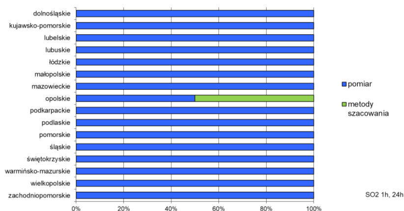
Rys. 3.1.5. Procent stref, w poszczególnych województwach, w których jako podstawę rocznej oceny dla SO 2 (stężenia 1-godz. i 24-godz., ochrona zdrowia) w 2022 r. wskazano określone metody
