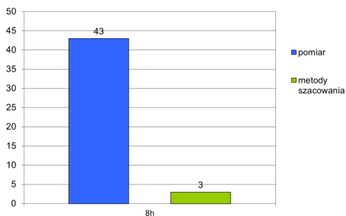
Rys. 3.3.2. Liczba stref, w których jako podstawę rocznej oceny dla CO (ochrona zdrowia) w 2022 r. wskazano określone metody
