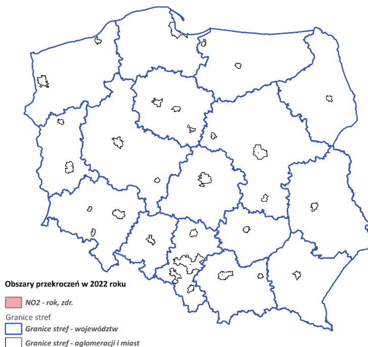
Rys. 3.2.11. Zasięg obszarów przekroczeń oszacowanych dla średniego rocznego stężenia NO 2 na obszarze Polski w 2022 roku
