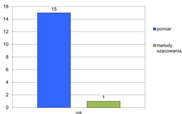
Rys. 4.2.2. Liczba stref, w których jako podstawę rocznej oceny dla NO x (ochrona roślin) w 2022 r. wskazano określone metody
