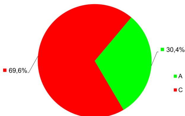
Rys. 3.11.3. Procent stref zaliczonych do określonych klas dla benzo(a)pirenu B(a)P w pyłe zawieszonym PM10 (ochrona zdrowia) w Polsce w 2022 r.
