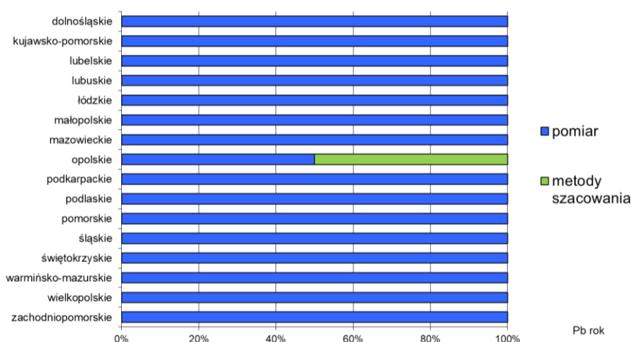
Rys. 3.8.3. Procent stref, w poszczególnych województwach, w których jako podstawę rocznej oceny dla Ni w pyłe zawieszonym PM10 (ochrona zdrowia) w 2022 r. wskazano określone metody
