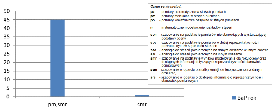
Rys. 3.11.6. Liczba stref, w których na potrzeby oceny dotyczącej B(a)P w pyłe zawieszonym PM10 (ochrona zdrowia) za 2022 rok wykorzystano wskazane szczegółowe metody oceny
