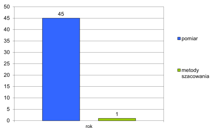
Rys. 3.8.3. Liczba stref, w których jako podstawę rocznej oceny dla As w pyłe zawieszonym PM10 (ochrona zdrowia) w 2022 r. wskazano określone metody
