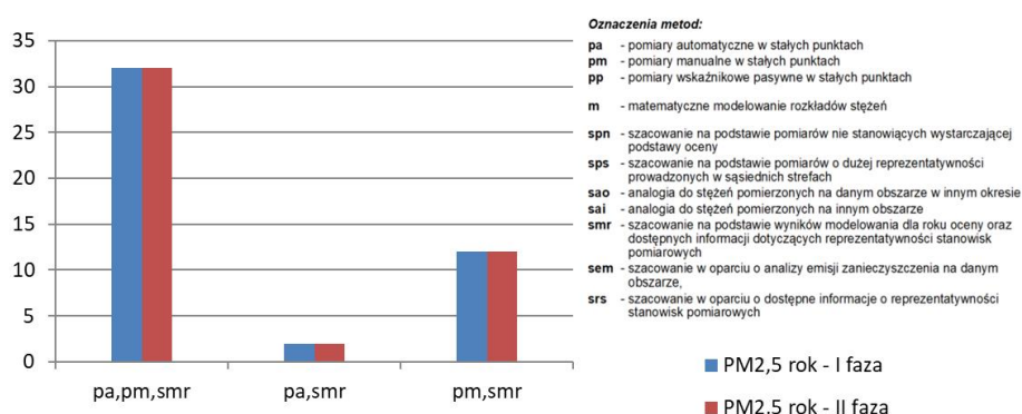
Rys. 3.12.8. Liczba stref, w których na potrzeby oceny dotyczącej pyłu zawieszonego PM2,5 (ochrona zdrowia) za 2022 rok wykorzystano wskazane szczegółowe metody oceny
