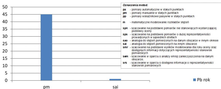
Rys. 3.7.4. Liczba stref, w których na potrzeby oceny dotyczącej Pb w pyłe zawieszonym PM10 (ochrona zdrowia) za 2022 rok wykorzystano wskazane szczegółowe metody oceny
