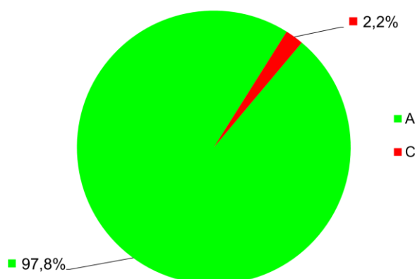
Rys. 3.12.4. Procent stref zaliczonych do określonych klas dla ozonu O 3 (poziom docelowy, ochrona roślin) w Polsce w 2022 r.
