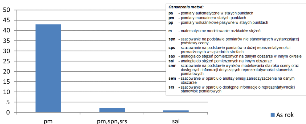
Rys. 3.8.5. Liczba stref, w których na potrzeby oceny dotyczącej As w pyłe zawieszonym PM10 (ochrona zdrowia) za 2022 rok wykorzystano wskazane szczegółowe metody oceny
