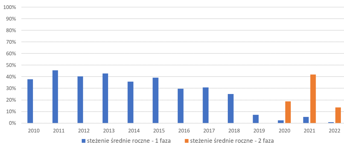
Rys. 3.13.2. Udział stanowisk pomiarowych na których wystąpiło przekroczenie poziomu dopuszczalnego pyłu zawieszonego PM 2,5 w ogólnej liczbie stanowisk uwzględnionych w ocenie w latach 2010-2022
