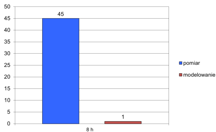
Rys. 3.5.3. Liczba stref, w których jako podstawę rocznej oceny dla ozonu O 3 (ochrona zdrowia) w 2022 r. wskazano określone metody
