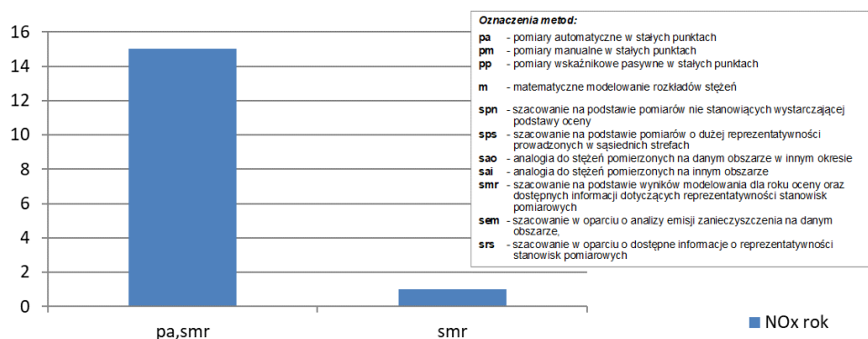
Rys. 4.2.3. Liczba stref, w których na potrzeby oceny dotyczącej NO x (ochrona roślin) za 2022 rok wykorzystano wskazane szczegółowe metody oceny
