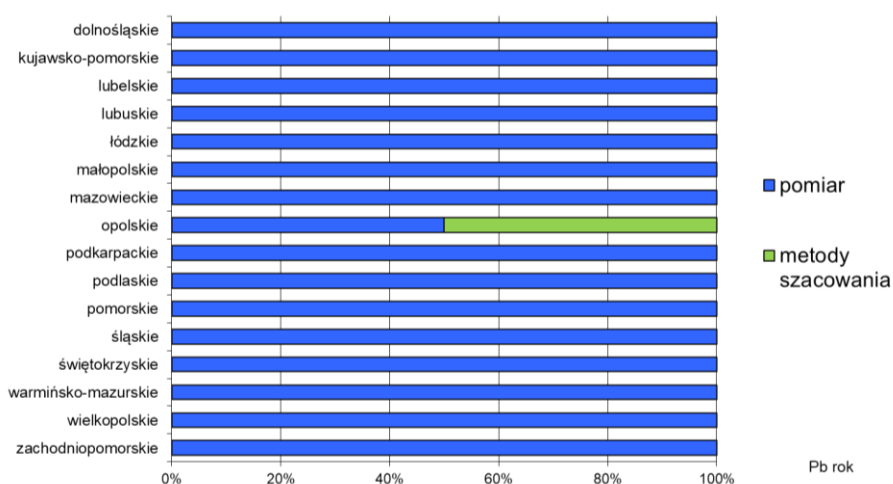
Rys. 3.9.3. Procent stref, w poszczególnych województwach, w których jako podstawę rocznej oceny dla Cd w pyłe zawieszonym PM10 (ochrona zdrowia) w 2022 r. wskazano określone metody
