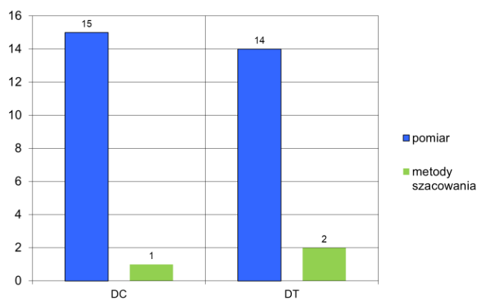
Rys. 4.3.3. Liczba stref, w których jako podstawę rocznej oceny dla ozonu (ochrona roślin, DC- poziom docelowy; DT- poziom celu długoterminowego) w 2022 r. wskazano określone metody
