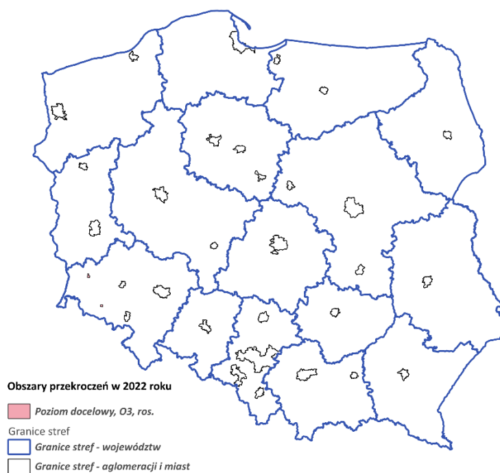
Rys. 4.3.8. Zasięg oszacowanych obszarów przekroczeń poziomu docelowego O 3 , w 2022 r. (ochrona roślin) Źródło danych: Główny Inspektorat Ochrony Środowiska, Opracowanie: INFAIR, IOŚ-PIB
