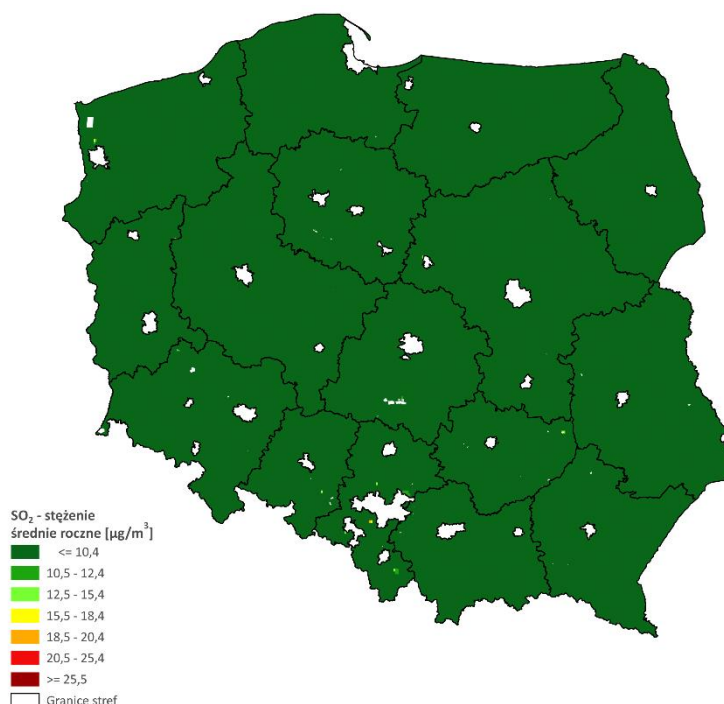
Rys. 4.1.4. Rozkład przestrzenny średniego rocznego stężenia SO 2 na obszarze Polski w 2022 roku, określony na podstawie modelowania matematycznego oraz obiektywnego szacowania
