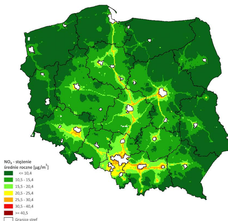
Rys. 4.2.4. Rozkład przestrzenny stężenia NO x na obszarze Polski w 2022 roku, wyrażony jako stężenie średnie roczne, określony na podstawie modelowania matematycznego oraz obiektywnego szacowania
