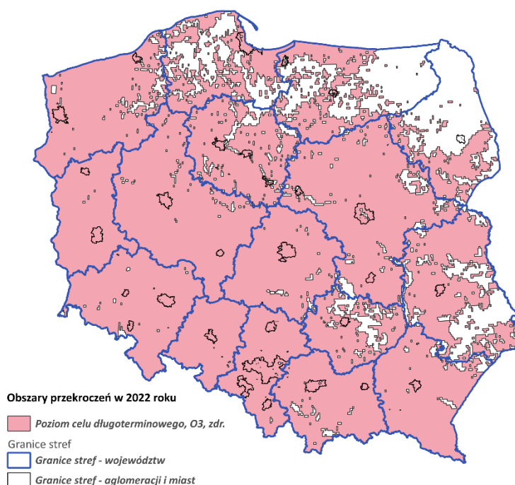
Rys. 3.5.8. Zasięg obszarów oszacowanych dla przekroczeń poziomu celu długoterminowego O 3 w 2022 r.
