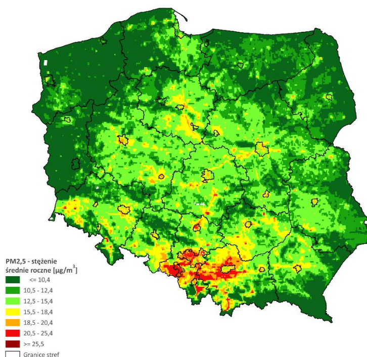
Rys. 3.12.9. Rozkład przestrzenny średniego rocznego stężenia pyłu zawieszonego PM 2,5 na obszarze Polski w 2022 roku, określony na podstawie modelowania matematycznego oraz obiektywnego szacowania
