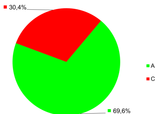
Rys. 3.6.6. Procent stref zaliczonych do określonych klas dla pyłu zawieszonego PM10 (klasa strefy, ochrona zdrowia) w Polsce w 2022 r.
