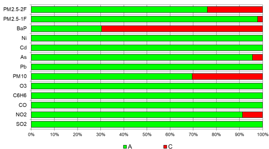
Rys. 3.13.1. Udział stref zaliczonych do określonych klas w łącznej liczbie stref w Polsce w 2022 r. dla poszczególnych zanieczyszczeń (klasy stref, ochrona zdrowia)
