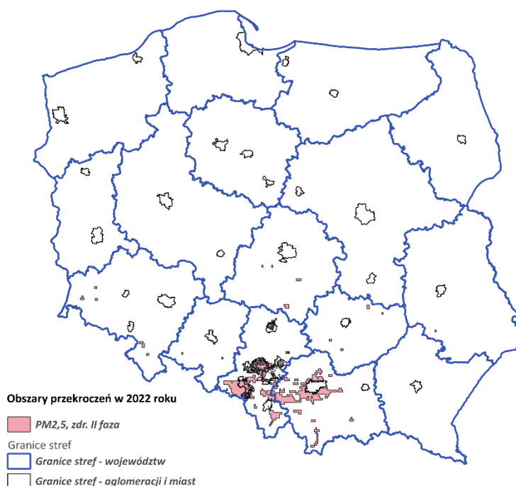
Rys. 3.12.10. Zasięg obszaru przekroczenia oszacowanego dla średniego rocznego stężenia pyłu zawieszonego PM2,5 na obszarze Polski w 2022 roku (II faza poziomu dopuszczalnego)
