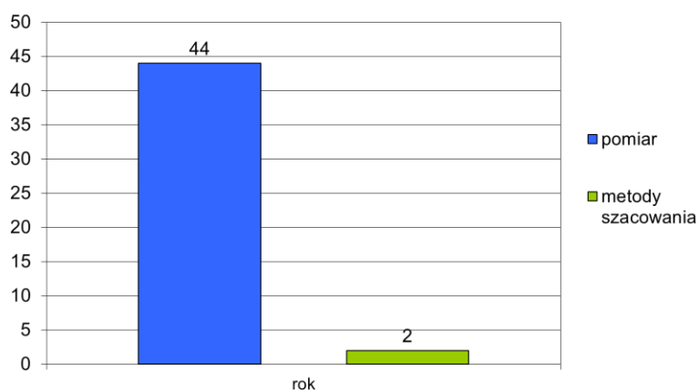
Rys. 3.4.2. Liczba stref, w których jako podstawę rocznej oceny dla benzenu C_6H_6 (ochrona zdrowia) w 2022 r. wskazano określone metody
