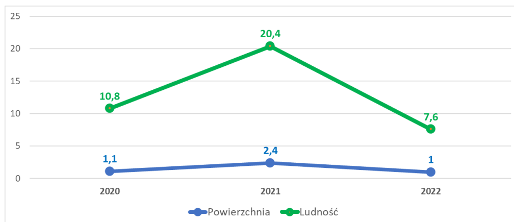
Rys. 3.12.11. Procentowy udział obszaru przekroczenia oszacowanego dla poziomu dopuszczalnego (II faza) dotyczącego wartości średnich rocznych stężenia pyłu zawieszonego PM2,5 w skali Polski w latach 2020 - 2022
