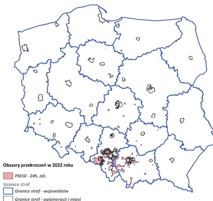
Rys. 3.6.11. Zasięg obszaru przekroczenia oszacowanego dla poziomu dopuszczalnego dotyczącego wartości średnich 24-godzinnych stężenia pyłu zawieszonego PM10 na obszarze Polski w 2022 roku
