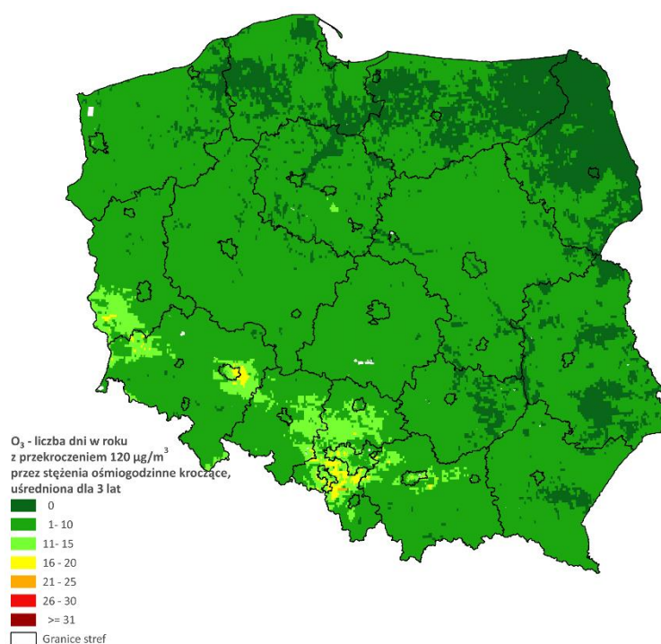
Rys. 3.5.6. Rozkład przestrzenny stężenia O 3 na obszarze Polski w 2022 roku, wyrażony jako liczba dni w roku z przekroczeniem poziomu 120 µg/m 3 przez wartości średnie 8-godzinne kroczące, uśredniona dla 3 lat, określony na podstawie modelowania matematycznego
