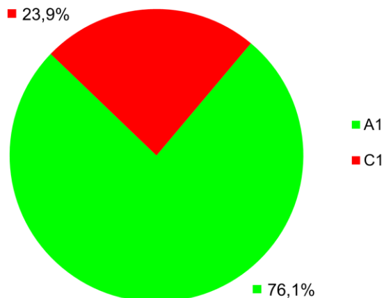
Rys. 3.12.3. Procent stref zaliczonych do określonych klas dla pyłu zawieszonego PM 2,5 (klasa strefy, ochrona zdrowia) w Polsce w 2022 r.
