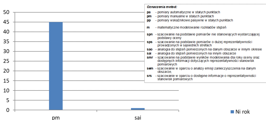
Rys. 3.10.3. Liczba stref, w których na potrzeby oceny dotyczącej Ni w pyłe zawieszonym PM10 (ochrona zdrowia) za 2022 rok wykorzystano wskazane szczegółowe metody oceny
