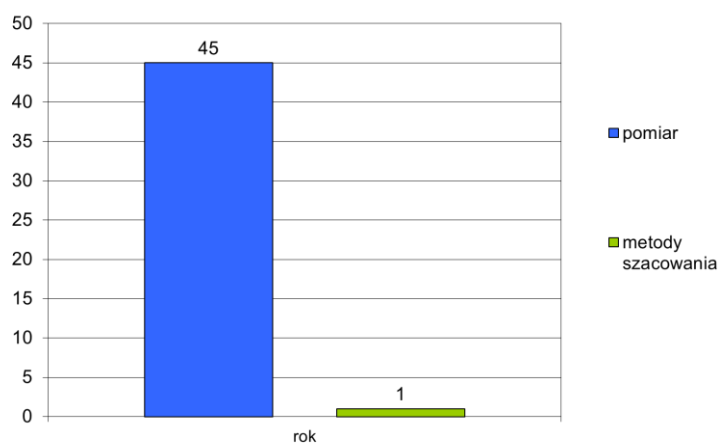
Rys. 3.7.2. Liczba stref, w których jako podstawę rocznej oceny dla Pb w pyłe zawieszonym PM10 (ochrona zdrowia) w 2022 r. wskazano określone metody
