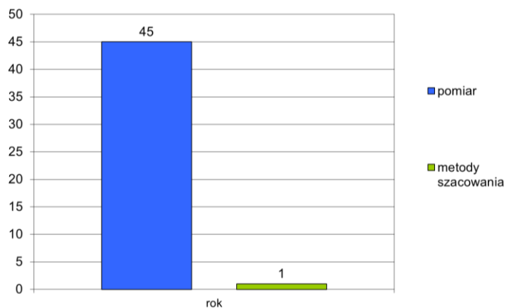
Rys. 3.8.3. Liczba stref, w których jako podstawę rocznej oceny dla Ni w pyłe zawieszonym PM10 (ochrona zdrowia) w 2022 r. wskazano określone metody
