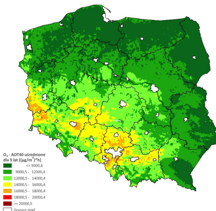
Rys. 4.3.6. Rozkład przestrzenny wartości wskaźnika AOT40 dla O 3 na obszarze Polski uśrednionej dla okresu 5 lat (2018 – 2022), określony na podstawie modelowania matematycznego oraz obiektywnego szacowania
