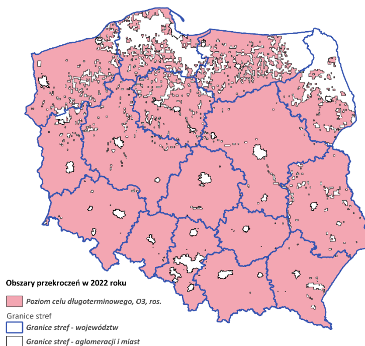
Rys. 4.3.9. Zasięg oszacowanych obszarów przekroczeń poziomu celu długoterminowego O 3 , w 2022 r. (ochrona roślin) Źródło danych: Główny Inspektorat Ochrony Środowiska, Opracowanie: INFAIR, IOŚ-PIB
