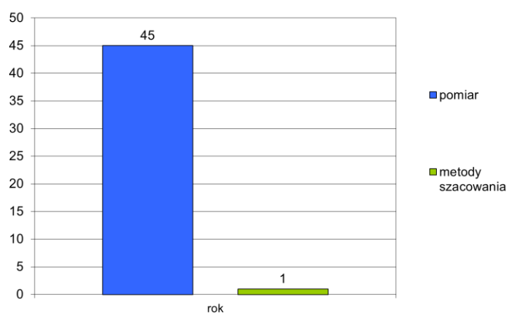
Rys. 3.11.4. Liczba stref, w których jako podstawę rocznej oceny dla B(a)P w pyłe zawieszonym PM10 (ochrona zdrowia) w 2022 r. wskazano określone metody
