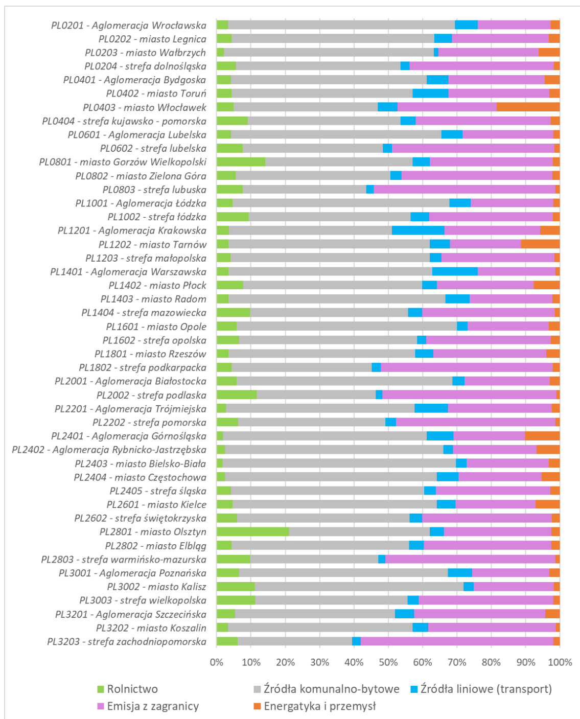
Rys. 3.6.16. Uśredniony udział źródeł emisji w stężeniu pyłu zawieszonego PM10 w poszczególnych strefach w Polsce w 2022 roku (dla ocenianego parametru związanego ze stężeniem średnim rocznym) oszacowany na podstawie modelowania
