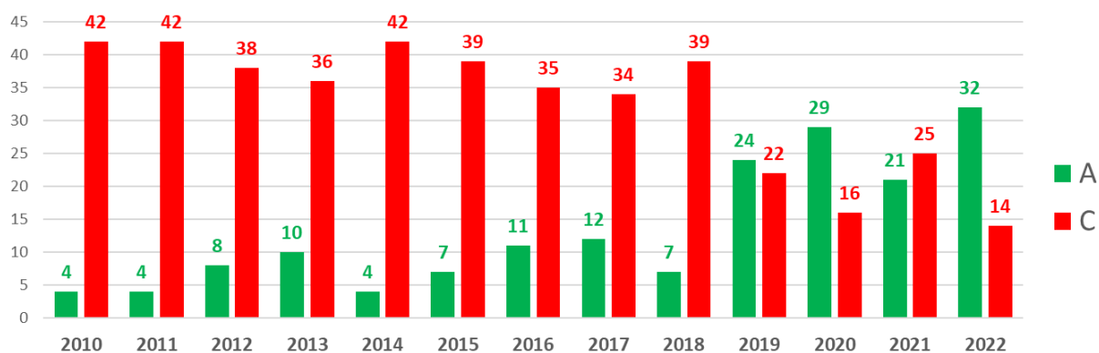
Rys. 3.6.2. Liczba stref z klasą A oraz C, określona na podstawie 24-godz. stężeń pyłu zawieszonego PM10 w wyniku ocen jakości powietrza za lata 2010 - 2022 (ochrona zdrowia)
