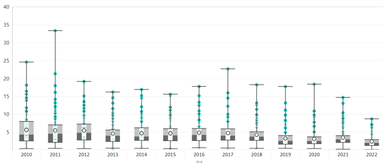
Rys. 3.13.6. Wykres pudełkowy - wartości parametrów statystycznych (minimum, maksimum, średnia, mediana, pierwszy i trzeci kwartyl) obliczone z mierzonych w Polsce średnich rocznych stężeń benzo(a)pirenu w latach 2010 – 2022 [ng/m 3 ]
