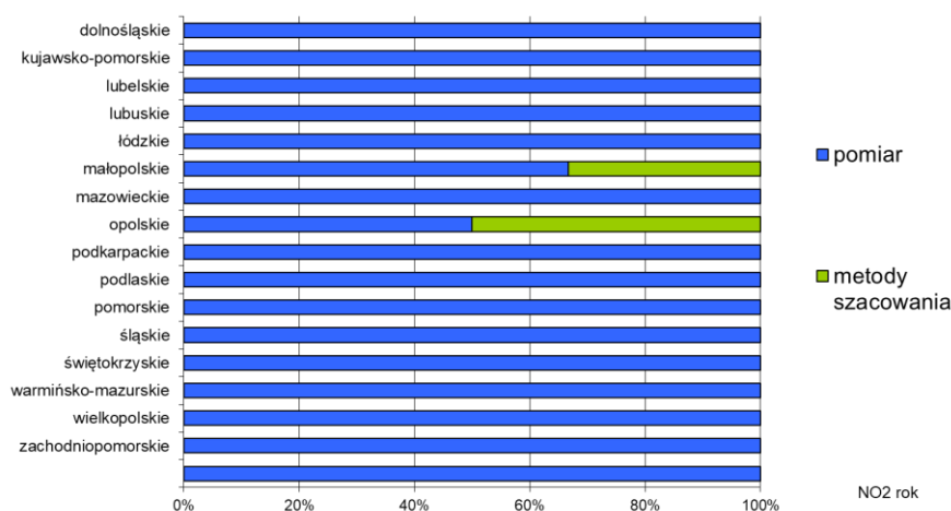
Rys. 3.2.7. Procent stref, w poszczególnych województwach, w których jako podstawę rocznej oceny dla NO 2 (stężenia średnie roczne, ochrona zdrowia) w 2022 r. wskazano określone metody
