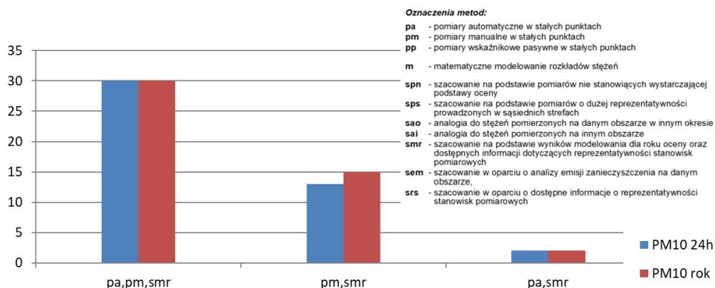
Rys. 3.6.8. Liczba stref, w których na potrzeby oceny dotyczącej pyłu zawieszonego PM10 (stężenia średnie 24-godz. i roczne, ochrona zdrowia) za 2022 rok wykorzystano wskazane szczegółowe metody oceny
