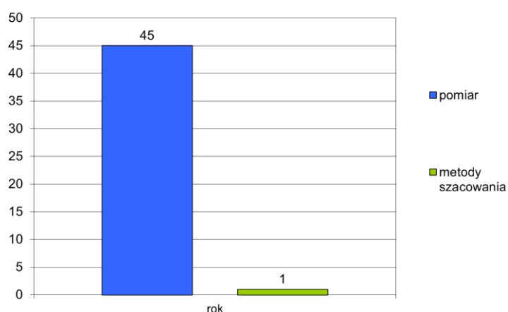
Rys. 3.9.2. Liczba stref, w których jako podstawę rocznej oceny dla Cd w pyłe zawieszonym PM10 (ochrona zdrowia) w 2022 r. wskazano określone metody
