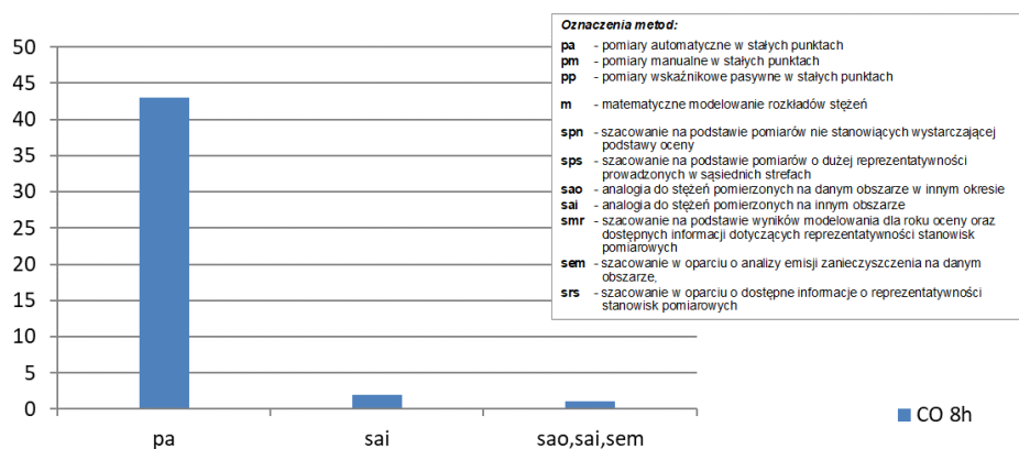
Rys. 3.3.4. Liczba stref, w których na potrzeby oceny dotyczącej CO (ochrona zdrowia) za 2022 rok wykorzystano wskazane szczegółowe metody oceny
