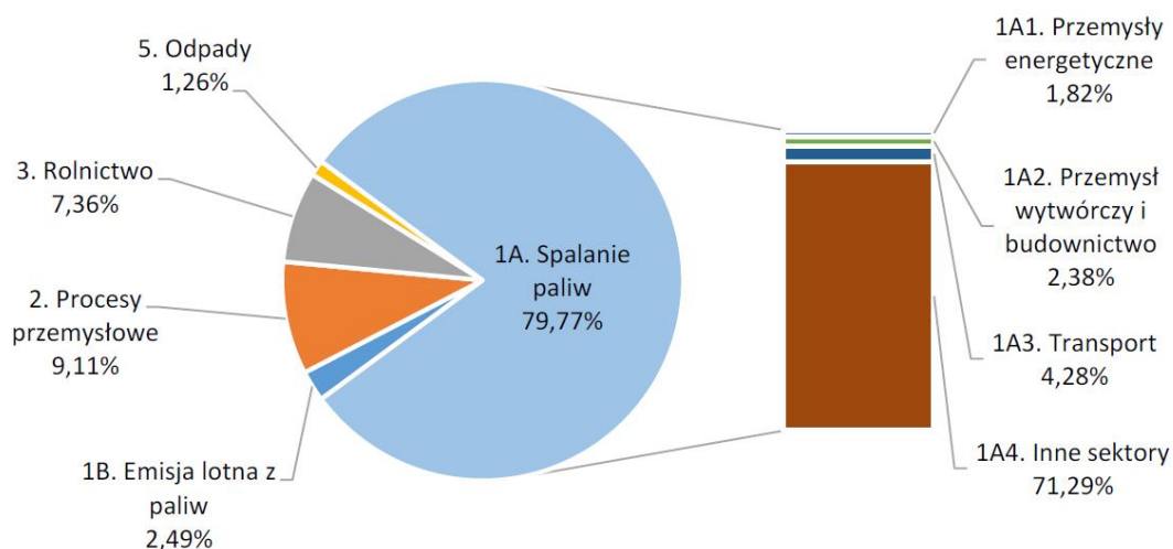
Rys. 3.6.18. Udział istotnych sektorów w emisji pyłu PM 10 w Polsce w roku 2021
