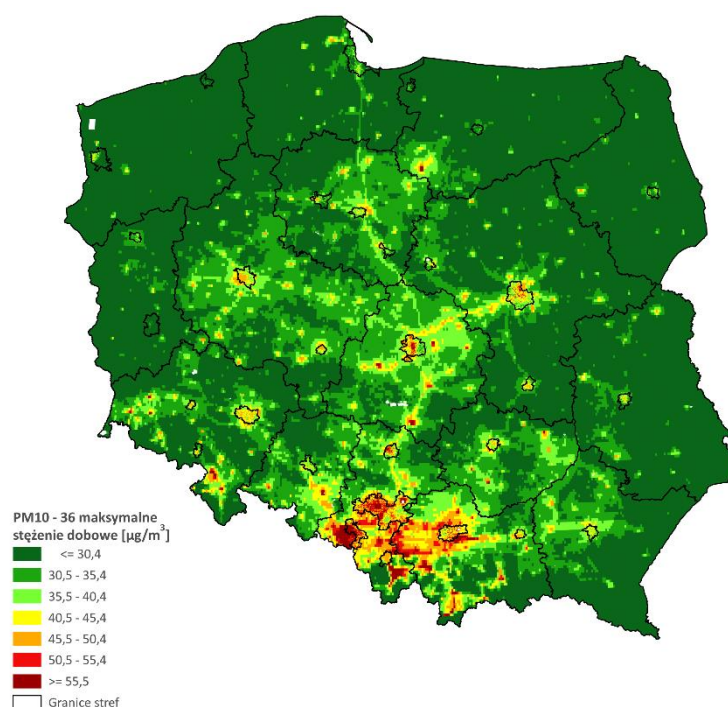
Rys. 3.6.9. Rozkład przestrzenny stężenia pyłu zawieszonego PM10 na obszarze Polski w 2022 roku, wyrażony jako 36-te maksymalne stężenie średnie dobowe, określony na podstawie modelowania matematycznego oraz obiektywnego szacowania
