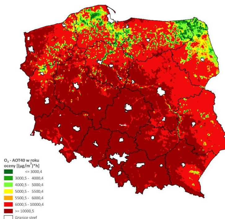
Rys. 4.3.7. Rozkład przestrzenny wartości wskaźnika AOT40 dla O 3 na obszarze Polski w roku 2022 określony na podstawie modelowania matematycznego oraz obiektywnego szacowania
