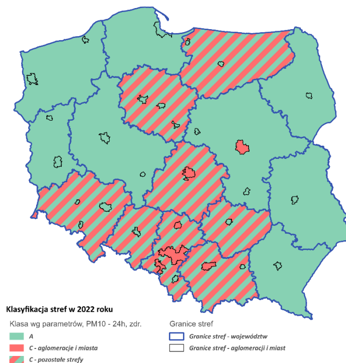
Rys. 3.6.1. Klasy stref określone na podstawie 24-godz. stężeń pyłu zawieszonego PM10 w wyniku oceny jakości powietrza za rok 2022 (ochrona zdrowia)
