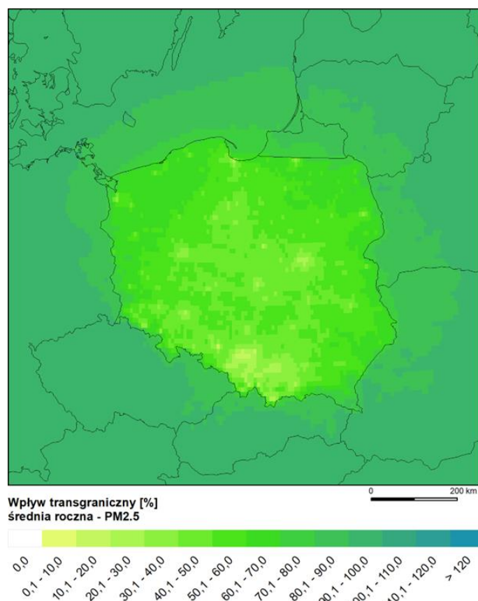
Rys. 3.12.15. Rozkład przestrzenny udziału procentowego źródeł zagranicznych w odniesieniu do stężenia średniego rocznego pyłu PM 2,5 na obszarze Polski w 2022 roku, na podstawie wyników modelowania modelem GEM-AQ
