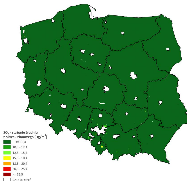
Rys. 4.1.5. Rozkład przestrzenny stężenia średniego SO 2 na obszarze Polski w okresie zimowym 2022 roku, określony na podstawie modelowania matematycznego oraz obiektywnego szacowania
