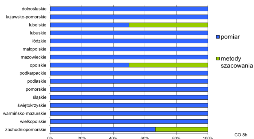
Rys. 3.3.3. Procent stref, w poszczególnych województwach, w których jako podstawę rocznej oceny dla CO (ochrona zdrowia) w 2022 r. wskazano określone metody
