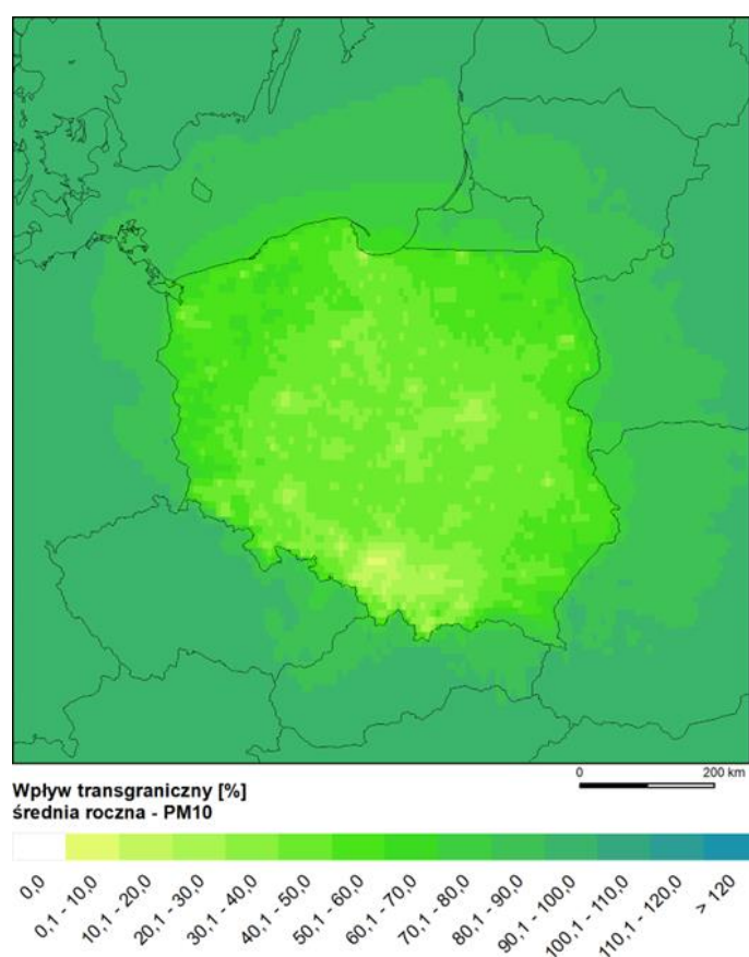
Rys. 3.6.17. Rozkład przestrzenny udziału procentowego źródeł zagranicznych w odniesieniu do stężenia średniego rocznego pyłu zawieszonego PM 10 na obszarze Polski w 2022 roku (model GEM-AQ)
