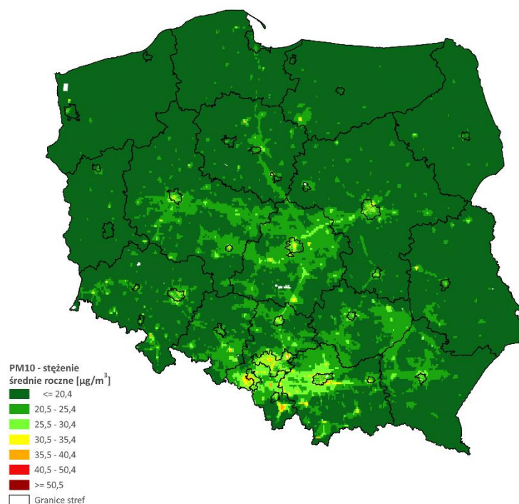
Rys. 3.6.10. Rozkład przestrzenny średniego rocznego stężenia pyłu zawieszonego PM10 na obszarze Polski w 2022 roku, określony na podstawie modelowania matematycznego oraz obiektywnego szacowania
