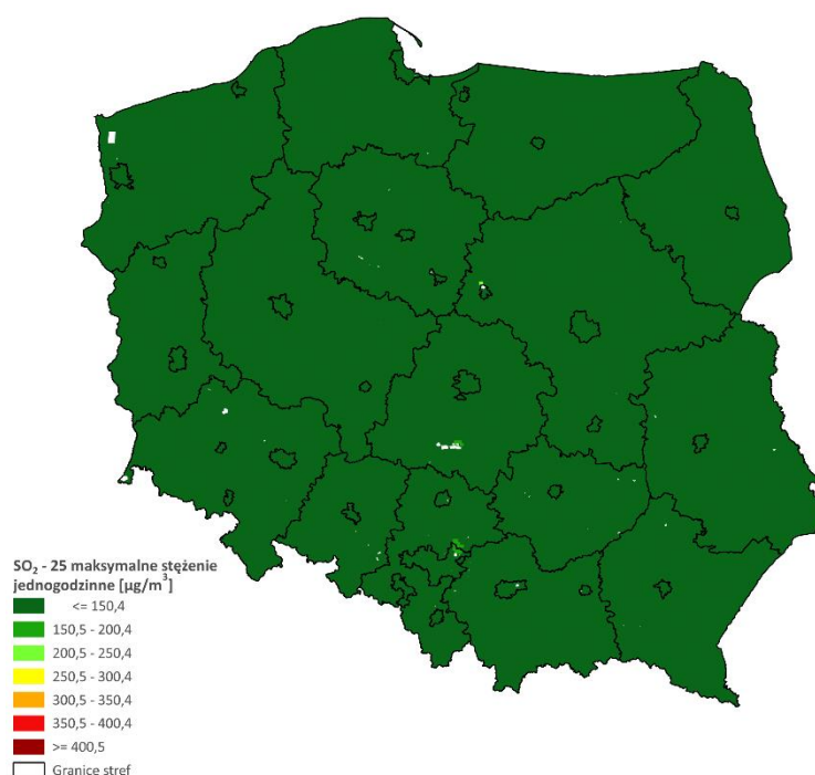
Rys. 3.1.7. Rozkład przestrzenny stężenia SO 2 na obszarze Polski w 2022 roku, wyrażony jako 25-te maksymalne stężenie średnie 1-godzinne, określony na podstawie modelowania matematycznego oraz obiektywnego szacowania
