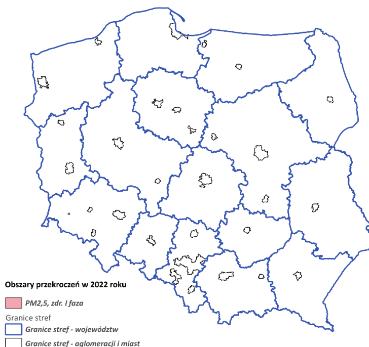
Rys. 3.12.12. Zasięg obszaru przekroczenia oszacowanego dla średniego rocznego stężenia pyłu zawieszonego PM2,5 na obszarze Polski w 2022 roku (I faza poziomu dopuszczalnego)
