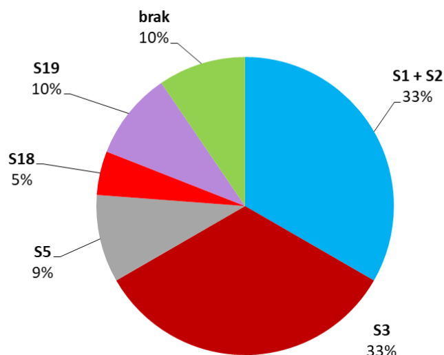
Rys. 3.6.14. Przyczyny wystąpienia sytuacji przekroczeń dopuszczalnego poziomu 24-godz. stężeń pyłu zawieszonego PM10 w strefach zaliczonych do klasy C w 2022 roku, wskazane jako dodatkowe dla poszczególnych przypadków przekroczeń – udział procentowy w skali kraju
