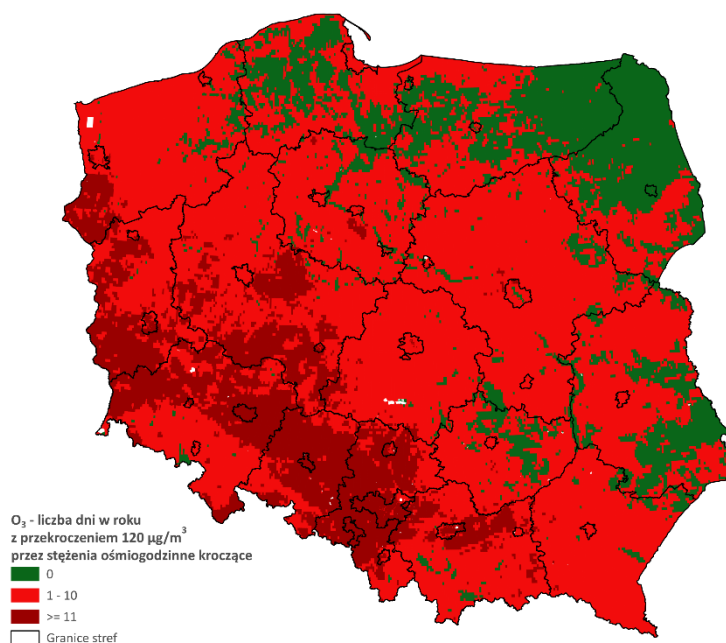
Rys. 3.5.7. Rozkład przestrzenny stężenia O 3 na obszarze Polski w 2022 roku, wyrażony jako liczba dni w roku z przekroczeniem poziomu 120 µg/m 3 przez wartości średnie 8-godzinne kroczące, określony na podstawie modelowania matematycznego oraz obiektywnego szacowania
