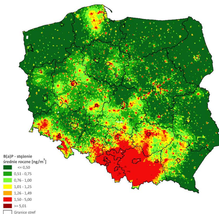
Rys. 3.11.7. Rozkład przestrzenny średniego rocznego stężenia B(a)P w pyłe zawieszonym PM 10 na obszarze Polski w 2022 roku, określony na podstawie modelowania matematycznego oraz obiektywnego szacowania
