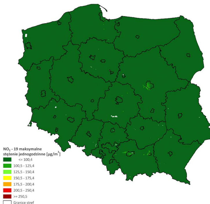
Rys. 3.2.9. Rozkład przestrzenny stężenia NO 2 na obszarze Polski w 2022 roku, wyrażony jako 19-te maksymalne stężenie 1-godzinne, określony na podstawie modelowania matematycznego oraz obiektywnego szacowania
