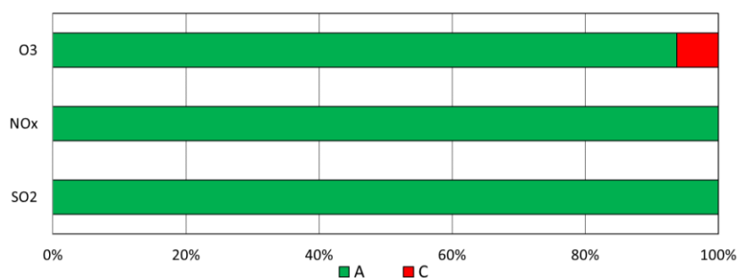
Rys. 4.4.1. Udział stref zaliczonych do klasy A lub C w łącznej liczbie stref w Polsce w 2022 r. dla poszczególnych zanieczyszczeń (ochrona roślin)
