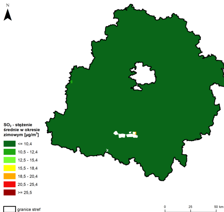
Rysunek 7.60. Rozkład przestrzenny wartości stężenia średniego dla pory zimowej SO 2 w województwie łódzkim w 2024 roku, opracowany z wykorzystaniem metody szacowania w oparciu o wyniki modelowania jakości powietrza dla roku 2024 wykonanego przez IOŚ-PIB [źródło: GIOŚ, IOŚ-PIB]
