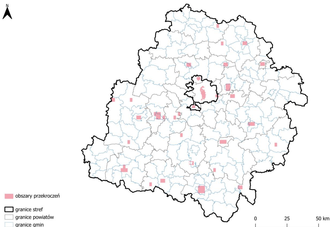
Rysunek 7.54. Zasięg obszarów przekroczeń poziomu docelowego B(a)P w pyłe zawieszonym PM 10 , określonego ze względu na ochronę zdrowia ludzi w województwie łódzkim w 2024 roku [źródło: GIOŚ]
