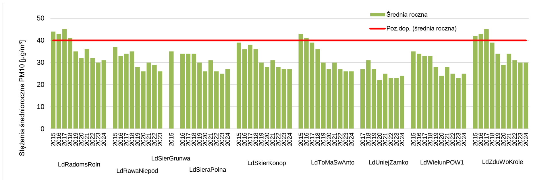
Rysunek 7.32. Przebieg wartości średniej rocznej stężenia pyłu zawieszonego PM10 na poszczególnych stanowiskach pomiarowych w województwie łódzkim, na tle poziomu dopuszczalnego w latach 2015 – 2024 (strefa oceny strefa łódzka – część II) [źródło: GIOŚ]
