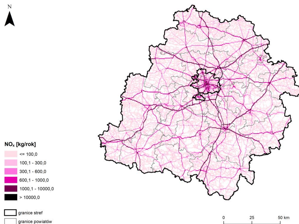
Rysunek 6.5. Zróżnicowanie wielkości emisji NO x ze źródeł liniowych na obszarze województwa łódzkiego [opracowanie GIOŚ, źródło: KOBiZE / IOŚ-PIB]
