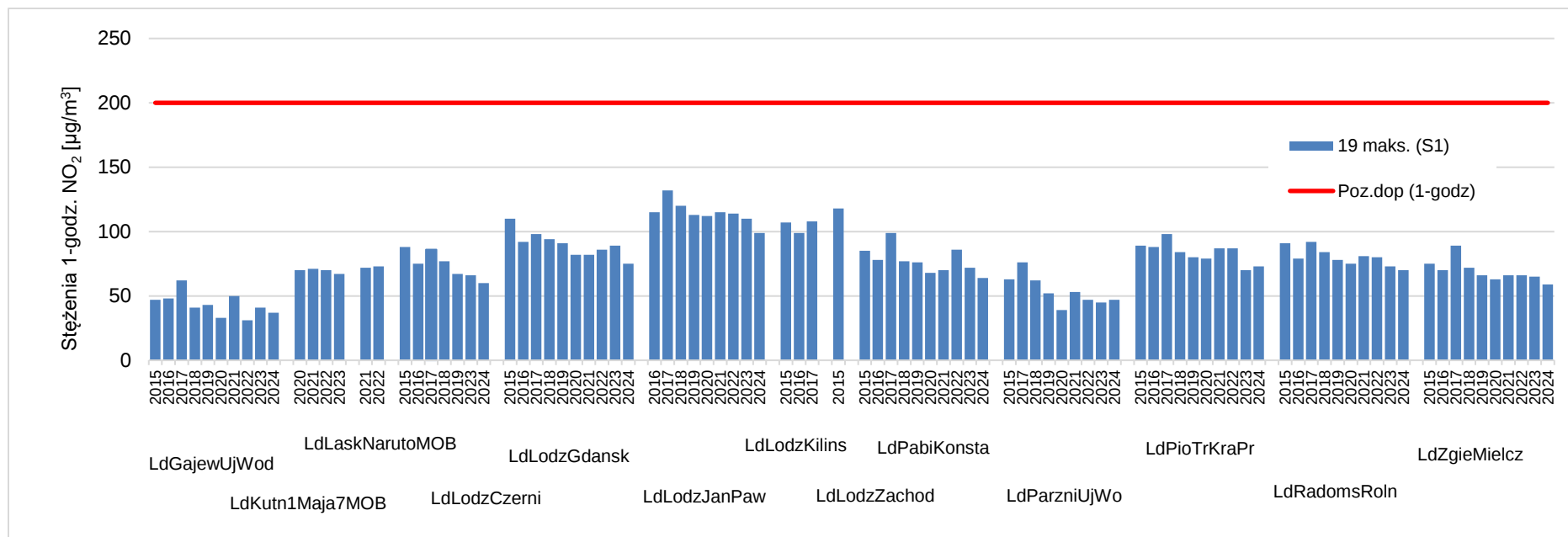
Rysunek 7.9. Przebieg 19 maksymalnej wartości 1-godzinowej stężenia NO 2 , na poszczególnych stanowiskach pomiarowych w województwie łódzkim, na tle poziomym dopuszczalnym w latach 2015 - 2024 [źródło: GIOŚ]
