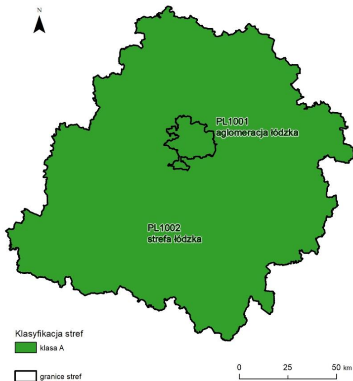
Rysunek 7.8. Klasyfikacja stref w województwie łódzkim za 2024 rok dla NO 2 dla czasu uśredniania - rok, z uwzględnieniem kryteriów określonych w celu ochrony zdrowia ludzi [źródło: GIOŚ]
