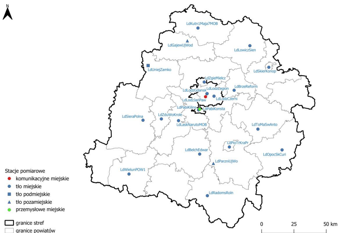
Rysunek 4.1. Lokalizacja stacji pomiarowych w województwie łódzkim, wykorzystanych w ocenie za rok 2024 [źródło: GIOŚ]
