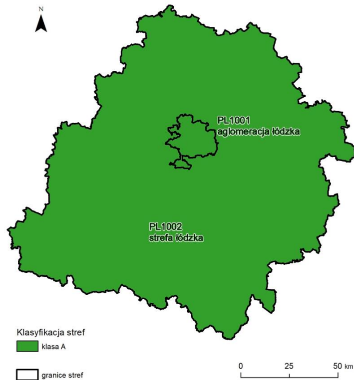
Rysunek 7.1. Klasyfikacja stref w województwie łódzkim za 2024 rok dla \text{SO}_2 dla czasu uśredniania - 1 godz., z uwzględnieniem kryteriów określonych w celu ochrony zdrowia ludzi [źródło: GIOŚ]
