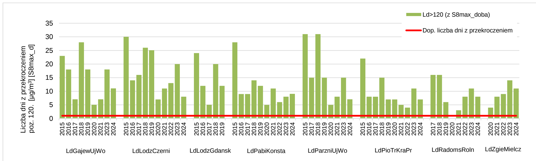
Rysunek 7.21. Przebieg liczby dni z przekroczeniami poziomu celu długoterminowego przez maksymalne dobowe stężenia 8-godzinne O 3 , na poszczególnych stanowiskach pomiarowych w województwie łódzkim, w latach 2015 - 2024 [źródło: GIOŚ]
