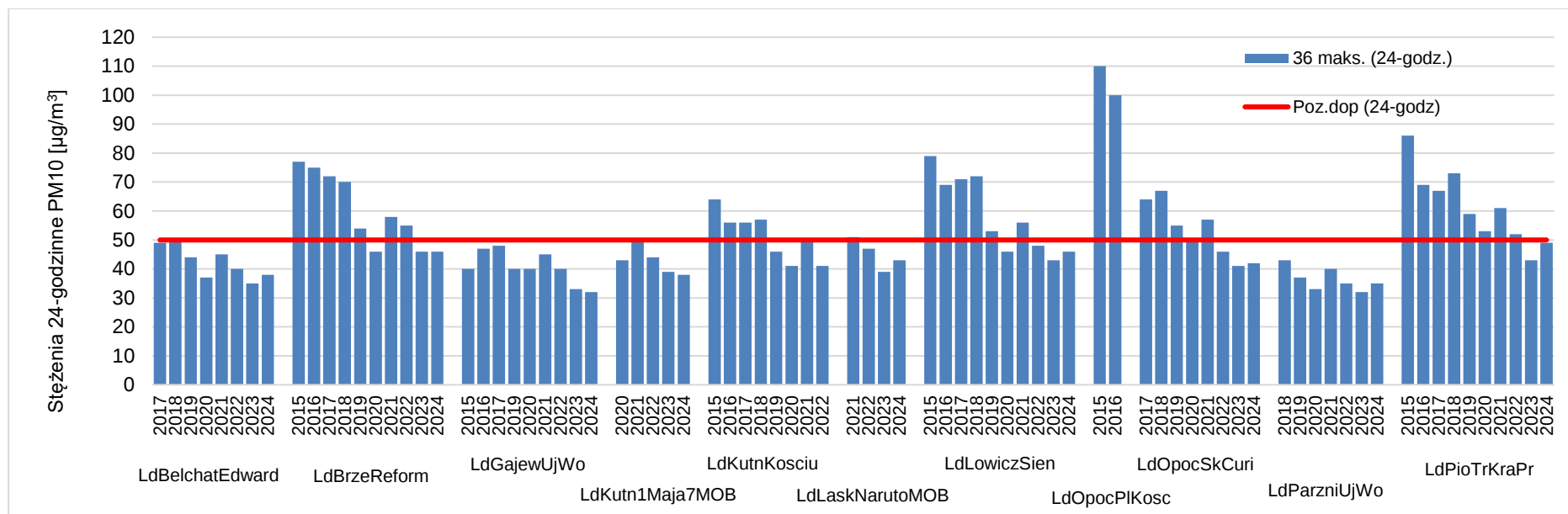
Rysunek 7.28. Przebieg 36 maksymalnej wartości 24-godzinowej stężenia pyłu zawieszonego PM10 na poszczególnych stanowiskach pomiarowych w województwie łódzkim, na tle poziomu dopuszczalnego w latach 2015 – 2024 (strefa oceny strefa łódzka - część I) [źródło: GIOŚ]
