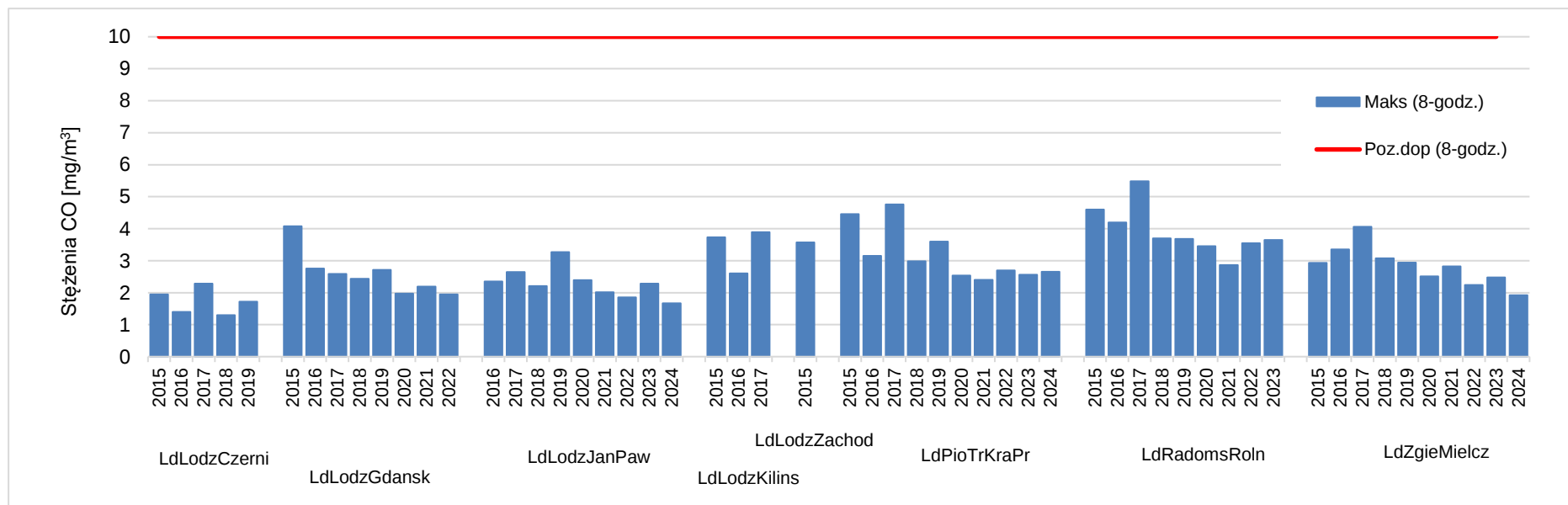
Rysunek 7.14. Przebieg maksymalnych wartości średnich 8-godzinnych stężenia CO na poszczególnych stanowiskach pomiarowych w województwie łódzkim na tle poziomu dopuszczalnego w latach 2015 - 2024 [źródło: GIOŚ]
