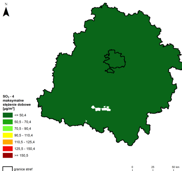
Rysunek 7.6. Rozkład przestrzenny 4 maksymalnej wartości stężenia 24-godzinne SO 2 w województwie łódzkim w 2024 roku, opracowany z wykorzystaniem metody szacowania w oparciu o wyniki modelowania jakości powietrza dla roku 2024 wykonanego przez IOŚ-PIB [źródło: GIOŚ, IOŚ-PIB]
