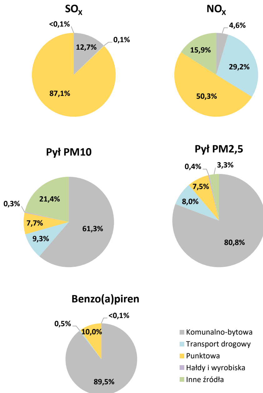
Rysunek 6.1. Udziały źródeł emisji w poszczególnych zanieczyszczeniach powietrza w województwie łódzkim [opracowanie GIOŚ, źródło: KOBiZE / IOŚ-PIB]
