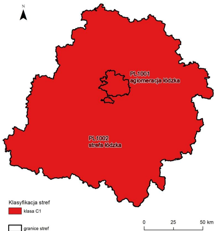
Rysunek 7.35. Klasyfikacja stref w województwie łódzkim za 2024 rok dla pyłu zawieszonego PM 2,5 , dla czasu uśredniania - rok, z uwzględnieniem kryteriów określonych w celu ochrony zdrowia ludzi – II faza [źródło: GIOŚ]
