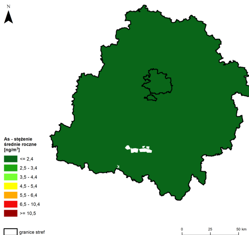
Rysunek 7.44. Rozkład przestrzenny wartości stężenia średniego rocznego As w pyłe zawieszonym PM10 w województwie łódzkim w 2024 roku, opracowany z wykorzystaniem metody szacowania w oparciu o wyniki modelowania jakości powietrza dla roku 2024 wykonanego przez IOŚ-PIB [źródło: GIOŚ, IOŚ-PIB]
