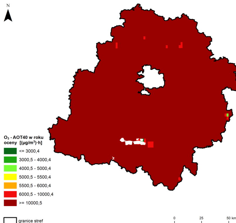
Rysunek 7.69. Rozkład przestrzenny wartości poziomu celu długoterminowego (wskaźnik AOT40) w województwie łódzkim w 2024 roku, opracowany z wykorzystaniem metody szacowania w oparciu o wyniki modelowania jakości powietrza dla roku 2024 wykonanego przez IOŚ-PIB [źródło: GIOŚ, IOŚ-PIB]
