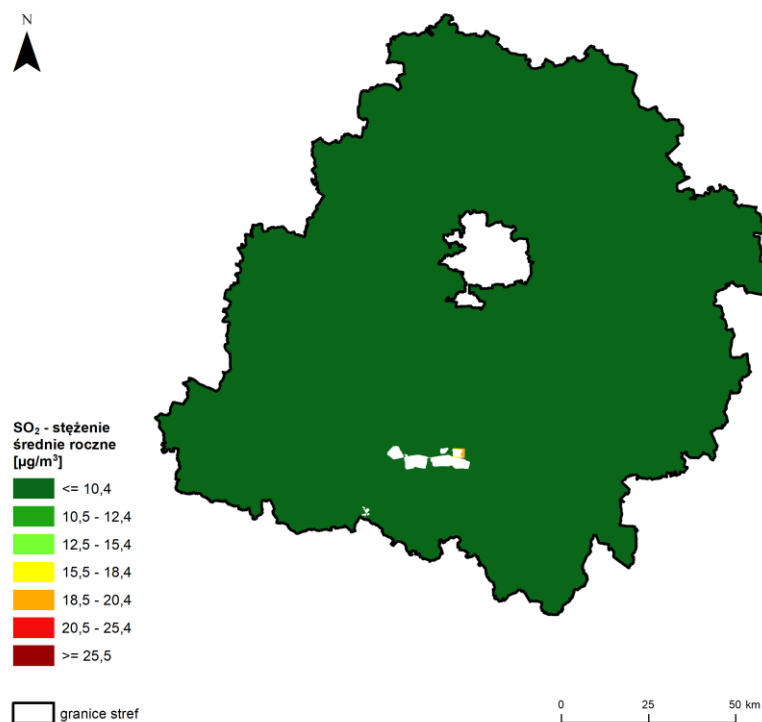
Rysunek 7.59. Rozkład przestrzenny wartości stężenia średniego rocznego SO 2 w województwie łódzkim w 2024 roku, opracowany z wykorzystaniem metody szacowania w oparciu o wyniki modelowania jakości powietrza dla roku 2024 wykonanego przez IOŚ-PIB [źródło: GIOŚ, IOŚ-PIB]
