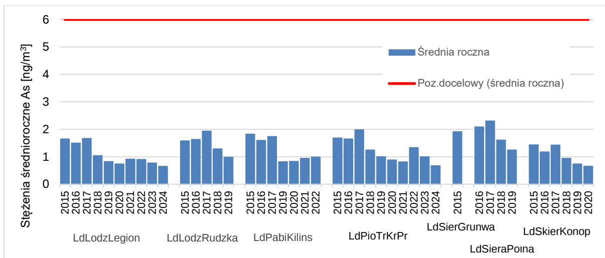
Rysunek 7.43. Przebieg wartości średnich rocznych stężeń As w pyłe zawieszonym PM10, na poszczególnych stanowiskach pomiarowych w województwie łódzkim, na tle poziomu docelowego w latach 2015 - 2024 [źródło: GIOŚ]
