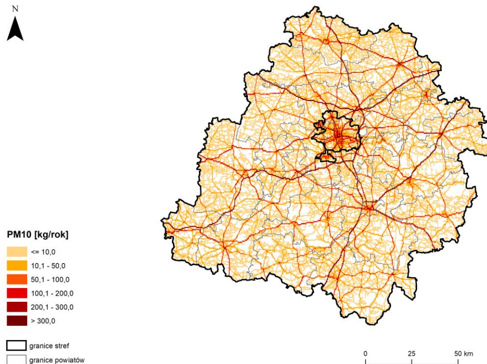
Rysunek 6.6. Zróżnicowanie wielkości emisji pyłu PM10 ze źródeł liniowych na obszarze województwa łódzkiego [opracowanie GIOŚ, źródło: KOBiZE / IOŚ-PIB]
