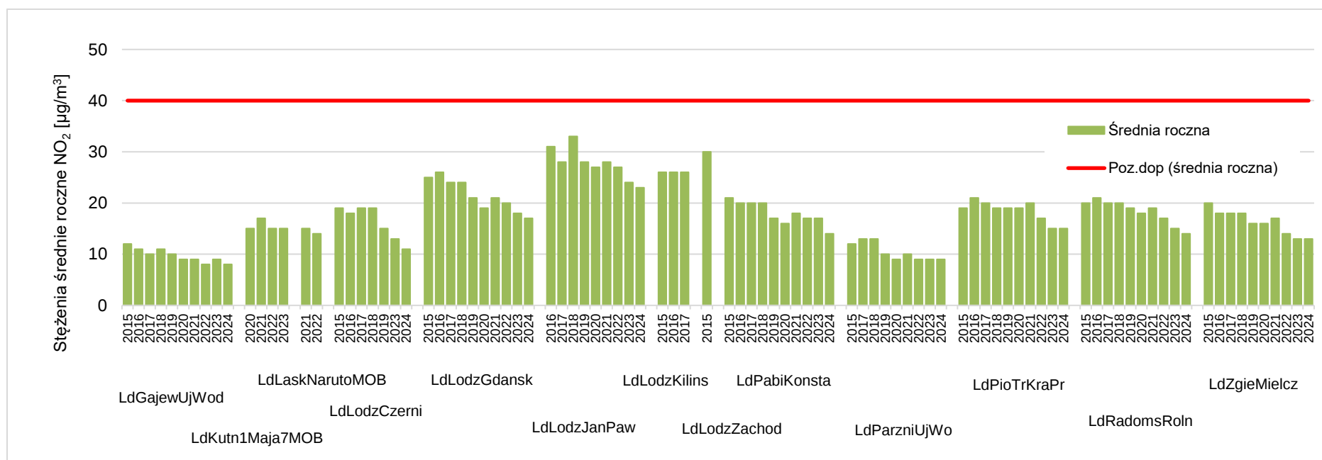
Rysunek 7.10. Przebieg wartości średniej rocznej stężenia NO 2 , na poszczególnych stanowiskach pomiarowych w województwie łódzkim, na tle poziomu dopuszczalnego w latach 2015 - 2024 [źródło: GIOŚ]
