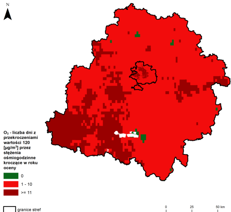
Rysunek 7.23. Rozkład przestrzenny liczby dni z przekroczeniem poziomu celu długoterminowego O 3 na obszarze województwa łódzkiego w 2024 roku, opracowany z wykorzystaniem metody szacowania w oparciu o wyniki modelowania jakości powietrza dla roku 2024 wykonanego przez IOŚ-PIB [źródło: GIOŚ, IOŚ-PIB]
