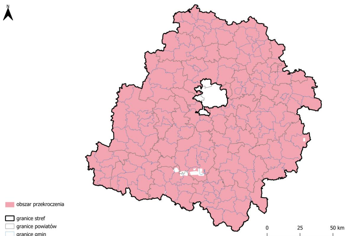
Rysunek 7.70. Zasięg obszaru przekroczenia poziomu celu długoterminowego (wskaznika AOT40) dla O 3 ustanowionego ze względu na ochronę roślin w województwie łódzkim w 2024 roku [źródło: GIOŚ]
