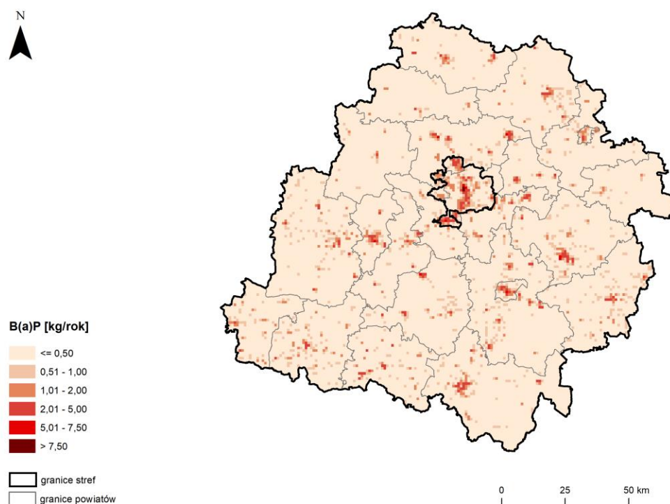
Rysunek 6.8. Zróżnicowanie wielkości emisji B(a)P ze źródeł komunalno-bytowych na obszarze województwa łódzkiego [opracowanie GIOŚ, źródło: KOBiZE / IOŚ-PIB]
