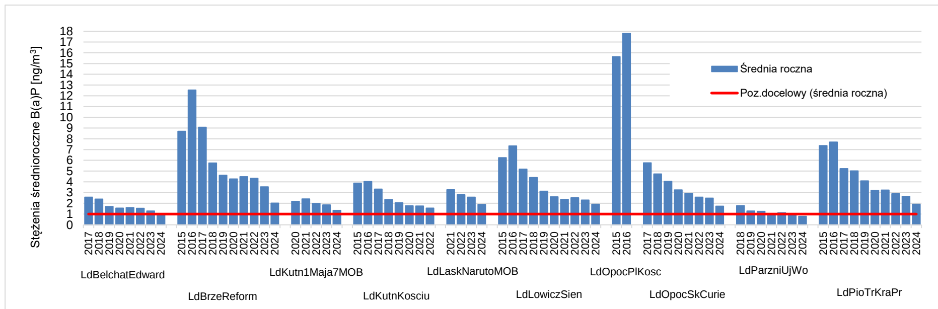
Rysunek 7.51. Przebieg wartości średnich rocznych stężeń B(a)P w pyłe zawieszonym PM10 na stanowiskach pomiarowych w województwie łódzkim, na tle poziomu docelowego w latach 2015 – 2024 (strefa oceny strefa łódzka – część I)(zgodnie z zasadami zaokrąglania wyników opisanymi w rozdz. 2.2 wartości poniżej 1,5 ng/m 3 nie stanowią przekroczenia poziomu docelowego benzo(a)pirenu w pyłe zawieszonym PM10) [źródło: GIOŚ]
