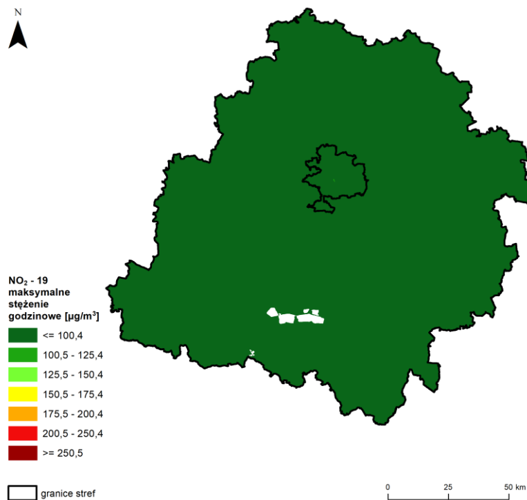
Rysunek 7.11. Rozkład przestrzenny 19 maksymalnej wartości stężenia 1-godzinowego NO 2 w województwie łódzkim w 2024 roku, opracowany z wykorzystaniem metody szacowania w oparciu o wyniki modelowania jakości powietrza dla roku 2024 wykonanego przez IOŚ-PIB [źródło: GIOŚ, IOŚ-PIB]
