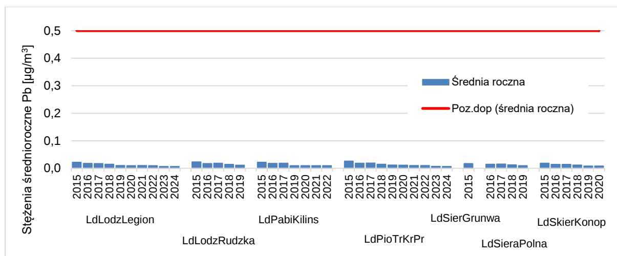
Rysunek 7.41. Przebieg wartości średnich rocznych stężeń Pb w pyłe zawieszonym PM10 na poszczególnych stanowiskach pomiarowych w województwie łódzkim na tle poziomu dopuszczalnego w latach 2015 - 2024 [źródło: GIOŚ]
