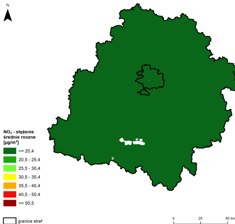
Rysunek 7.12. Rozkład przestrzenny wartości stężenia średniego rocznego NO 2 w województwie łódzkim w 2024 roku, opracowany z wykorzystaniem metody szacowania w oparciu o wyniki modelowania jakości powietrza dla roku 2024 wykonanego przez IOŚ-PIB [źródło: GIOŚ, IOŚ-PIB]
