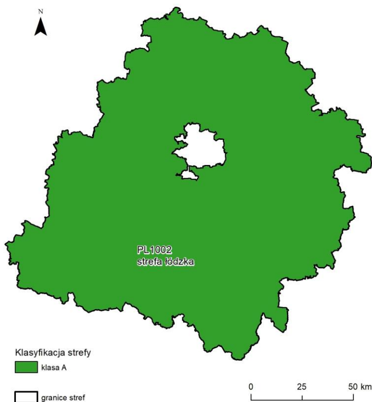
Rysunek 7.61. Klasyfikacja strefy w województwie łódzkim za 2024 rok dla \text{NO}_x dla czasu uśredniania - rok, z uwzględnieniem kryteriów określonych w celu ochrony roślin [źródło: GIOŚ]
