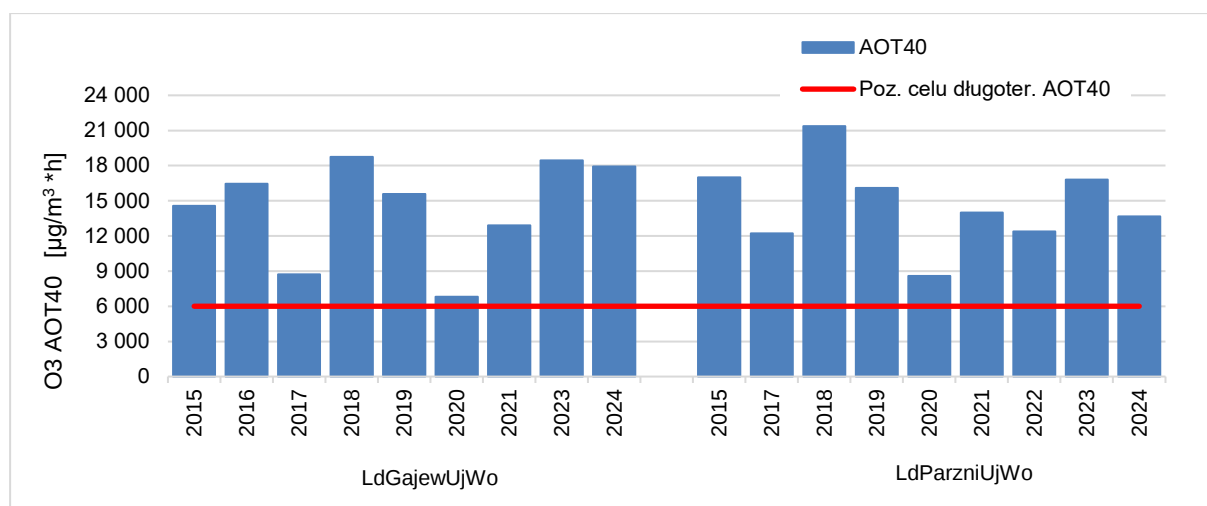
Rysunek 7.67. Przebieg wartości wskaźnika AOT40 dla O 3 , na stanowiskach pomiarowych w województwie łódzkim, uwzględnionych w ocenie pod kątem ochrony roślin, na tle poziomu celu długoterminowego w latach 2015 - 2024 (wartości dla danego roku) [źródło: GIOŚ]
