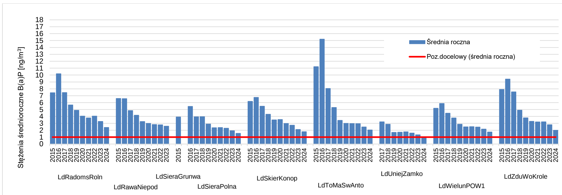
Rysunek 7.52. Przebieg wartości średnich rocznych stężeń B(a)P w pyłe zawieszonym PM10 na stanowiskach pomiarowych w województwie łódzkim, na tle poziomu docelowego w latach 2015 – 2024 (strefa oceny strefa łódzka – część II)(zgodnie z zasadami zaokrąglania wyników opisanymi w rozdz. 2.2 wartości poniżej 1,5 ng/m 3 nie stanowią przekroczenia poziomu docelowego benzo(a)pirenu w pyłe zawieszonym PM10) [źródło: GIOŚ]
