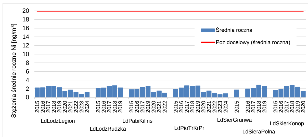
Rysunek 7.48. Przebieg wartości średnich rocznych stężeń Ni w pyłe zawieszonym PM 10 , na poszczególnych stanowiskach pomiarowych w województwie łódzkim, na tle poziomu docelowego w latach 2015 - 2024 [źródło: GIOŚ]
