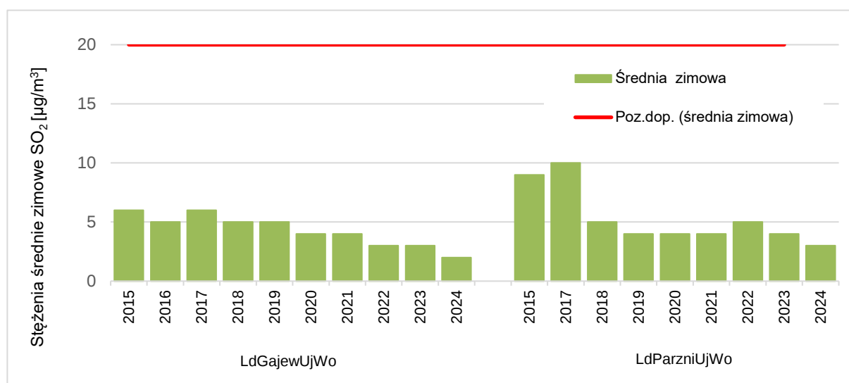
Rysunek 7.58. Przebieg wartości stężeń średnich z pory zimowej \text{SO}_2 , na stanowiskach pomiarowych w województwie łódzkim uwzględnionych w ocenie pod kątem ochrony roślin, na tle poziomu dopuszczalnego w latach 2015 - 2024 [źródło: GIOŚ]
