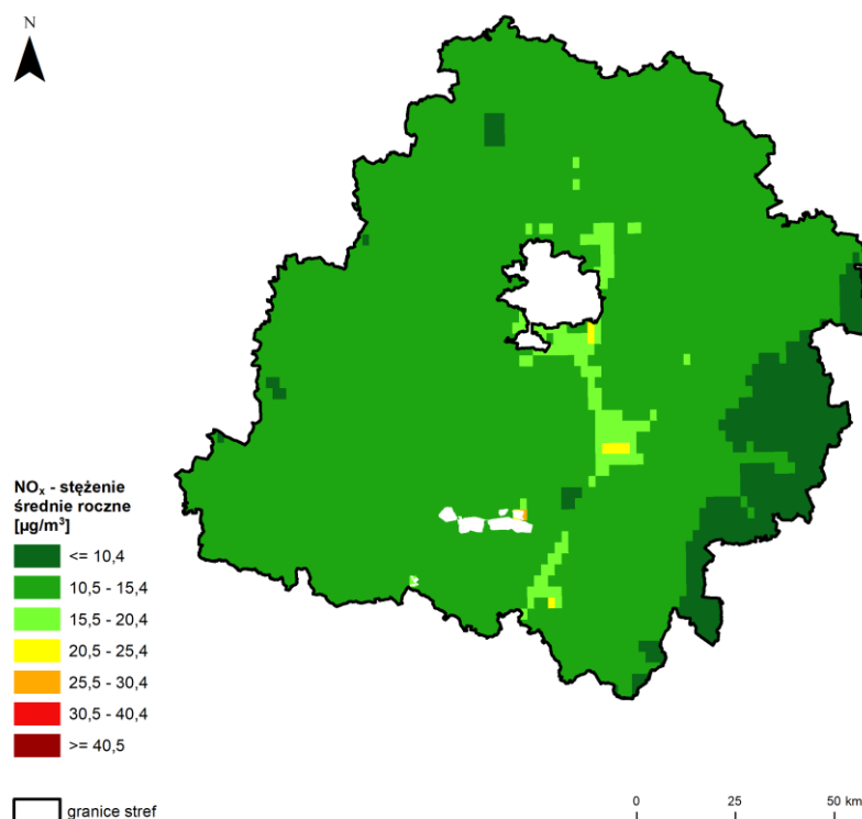
Rysunek 7.63. Rozkład przestrzenny wartości stężenia średniego rocznego NO x w województwie łódzkim w 2024 roku, opracowany z wykorzystaniem metody szacowania w oparciu o wyniki modelowania jakości powietrza dla roku 2024 wykonanego przez IOŚ-PIB [źródło: GIOŚ, IOŚ-PIB]
