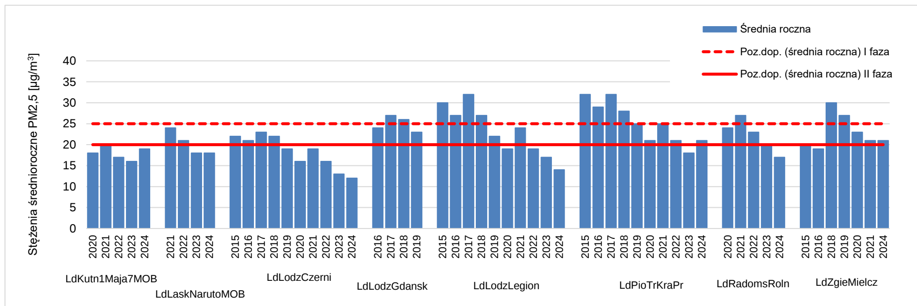
Rysunek 7.37. Przebieg wartości stężenia średniego rocznego pyłu zawieszonego PM 2,5 , na poszczególnych stanowiskach pomiarowych w województwie łódzkim na tle poziomu dopuszczalnego w latach 2015 - 2024 [źródło: GIOŚ]
