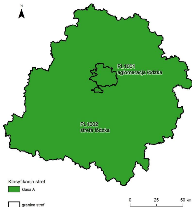
Rysunek 7.36. Klasyfikacja stref w województwie łódzkim za 2024 rok dla pyłu zawieszonego PM 2,5 , dla czasu uśredniania - rok, z uwzględnieniem kryteriów określonych w celu ochrony zdrowia ludzi – I faza [źródło: GIOŚ]
