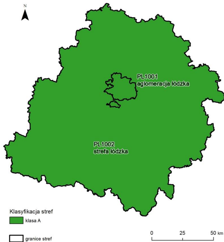
Rysunek 7.2. Klasyfikacja stref w województwie łódzkim za 2024 rok dla \text{SO}_2 dla czasu uśredniania - 24 godz., z uwzględnieniem kryteriów określonych w celu ochrony zdrowia ludzi [źródło: GIOŚ]
