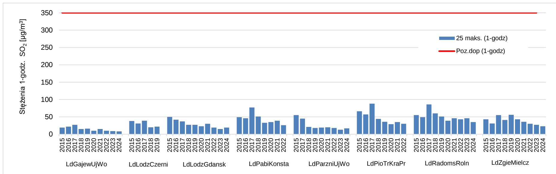
Rysunek 7.3. Przebieg 25 maksymalnej wartości godzinowej stężenia SO 2 , na poszczególnych stanowiskach pomiarowych w województwie łódzkim, na tle poziomu dopuszczalnego w latach 2015 – 2024 [źródło: GIOŚ]
