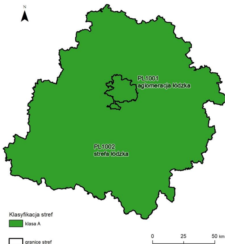
Rysunek 7.15. Klasyfikacja stref w województwie łódzkim za 2024 rok dla C_6H_6 dla czasu uśredniania - rok, z uwzględnieniem kryteriów określonych w celu ochrony zdrowia ludzi [źródło: GIOŚ]
