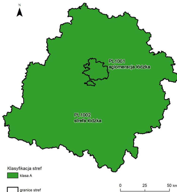
Rysunek 7.45. Klasyfikacja stref w województwie łódzkim za 2024 rok dla Cd w pyle zawieszonym PM10 dla czasu uśredniania - rok, z uwzględnieniem kryteriów określonych w celu ochrony zdrowia ludzi [źródło: GIOŚ]
