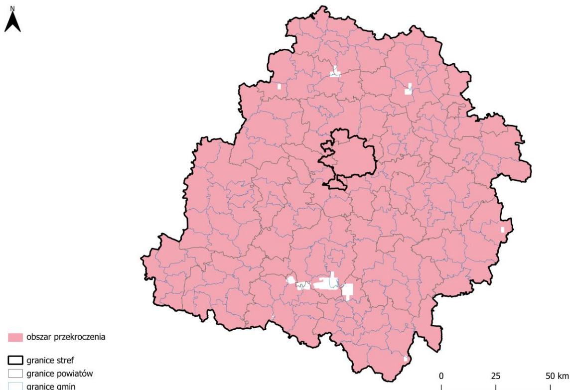
Rysunek 7.24. Zasięg obszaru przekroczenia poziomu celu długoterminowego dla O_3 , określonego ze względu na ochronę zdrowia ludzi, w województwie łódzkim w 2024 roku [źródło: GIOŚ]
