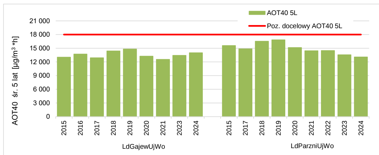
Rysunek 7.66. Przebieg wartości wskaźnika AOT40 5L dla O 3 , na stanowiskach pomiarowych w województwie łódzkim, uwzględnionych w ocenie pod kątem ochrony roślin, na tle poziomu docelowego w latach 2015 - 2024 (wartości uśrednione dla okresów 5-letnich) [źródło: GIOŚ]
