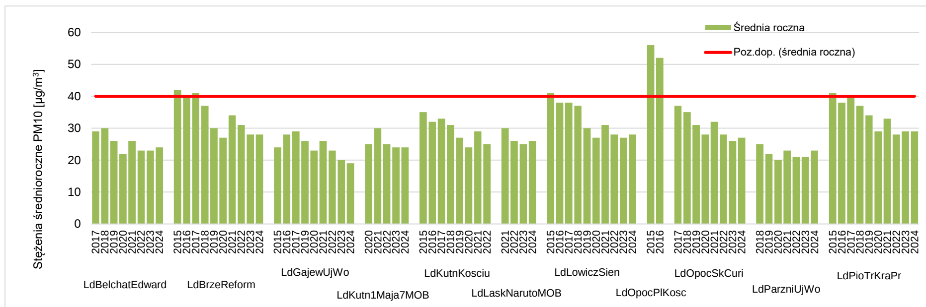
Rysunek 7.31. Przebieg wartości średniej rocznej stężenia pyłu zawieszonego PM10 na poszczególnych stanowiskach pomiarowych w województwie łódzkim, na tle poziomu dopuszczalnego w latach 2015 – 2024 (strefa oceny strefa łódzka – część I) [źródło: GIOŚ]
