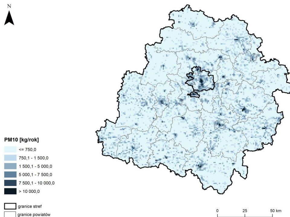
Rysunek 6.7. Zróżnicowanie wielkości emisji pyłu PM10 ze źródeł komunalno-bytowych na obszarze województwa łódzkiego [opracowanie GIOŚ, źródło: KOBiZE / IOŚ-PIB]
