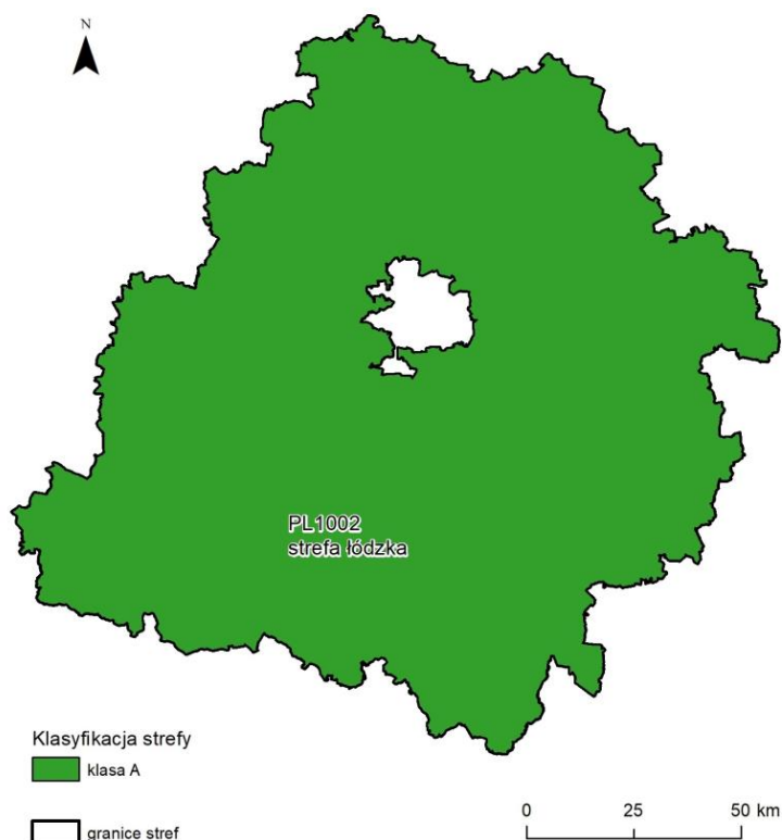
Rysunek 7.55. Klasyfikacja strefy w województwie łódzkim za 2024 rok dla SO 2 dla czasu uśredniania - rok, z uwzględnieniem kryteriów określonych w celu ochrony roślin [źródło: GIOŚ]
