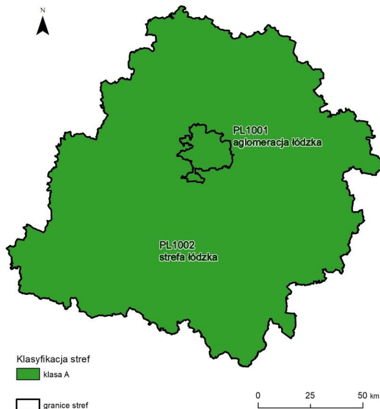
Rysunek 7.40. Klasyfikacja stref w województwie łódzkim za 2024 rok dla Pb w pyłe zawieszonym PM10 dla czasu uśredniania - rok, z uwzględnieniem kryteriów określonych w celu ochrony zdrowia ludzi [źródło: GIOŚ]
