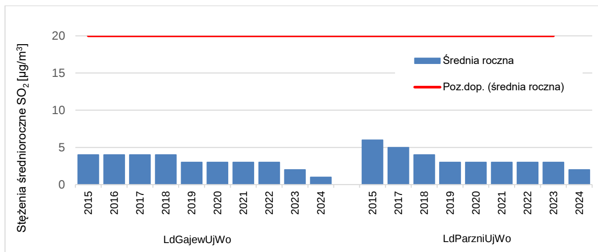
Rysunek 7.57. Przebieg wartości średnich rocznych stężeń \text{SO}_2 , na stanowiskach pomiarowych w województwie łódzkim uwzględnionych w ocenie pod kątem ochrony roślin, na tle poziomu dopuszczalnego w latach 2015 - 2024 [źródło: GIOŚ]
