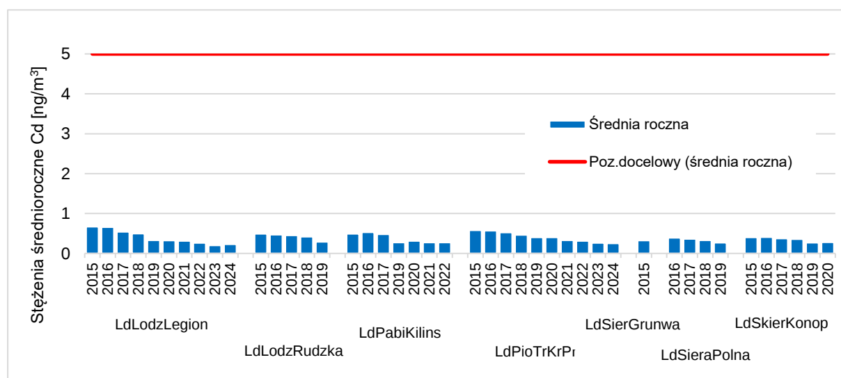
Rysunek 7.46. Przebieg wartości średnich rocznych stężeń Cd w pyłe zawieszonym PM10, na poszczególnych stanowiskach pomiarowych w województwie łódzkim, na tle poziomu docelowego w latach 2015 - 2024 [źródło: GIOŚ]
