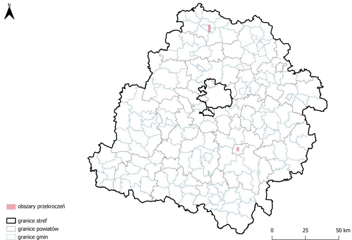
Rysunek 1. Zasięg obszarów przekroczeń poziomu dopuszczalnego pyłu zawieszonego PM 2,5 – faza II w województwie łódzkim w 2024 roku [źródło: GIOŚ]
