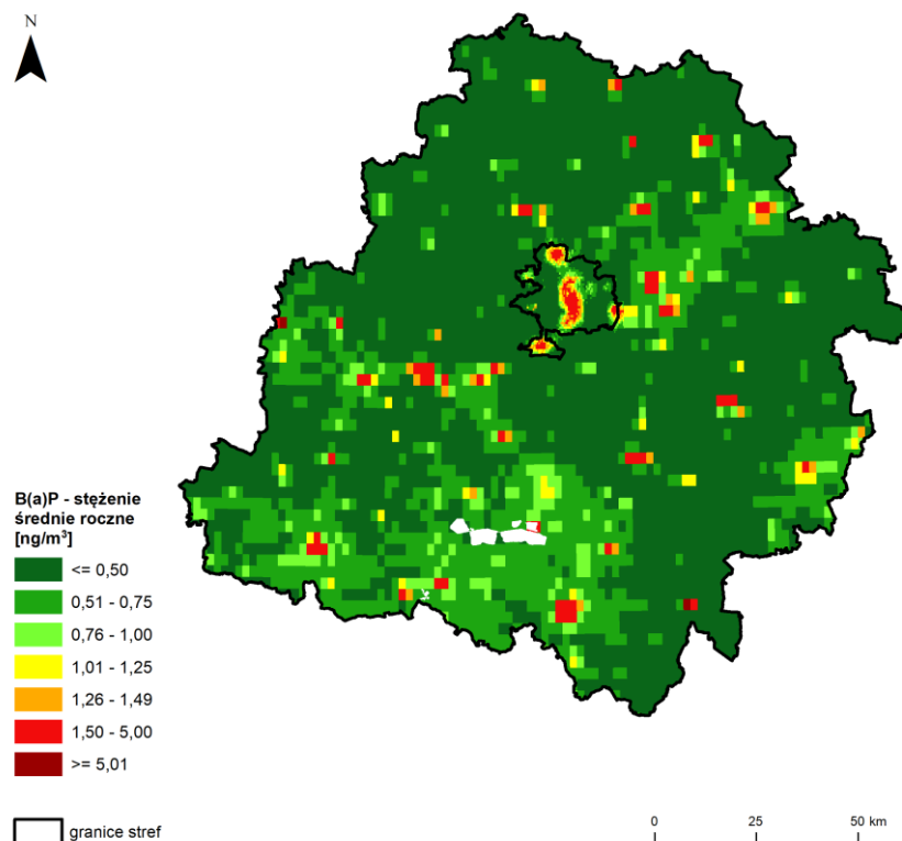
Rysunek 7.53. Rozkład przestrzenny wartości stężenia średniego rocznego B(a)P w pyłe zawieszonym PM10 w województwie łódzkim w 2024 roku, opracowany z wykorzystaniem metody szacowania w oparciu o wyniki modelowania jakości powietrza dla roku 2024 wykonanego przez IOŚ-PIB [źródło: GIOŚ, IOŚ-PIB]
