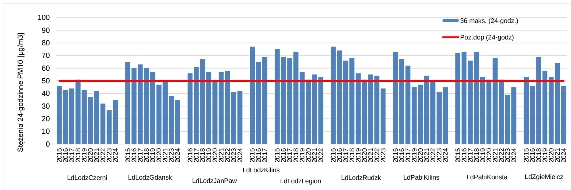
Rysunek 7.27. Przebieg 36 maksymalnej wartości 24-godzinowej stężenia pyłu zawieszonego PM10 na poszczególnych stanowiskach pomiarowych w województwie łódzkim, na tle poziom dopuszczalnego w latach 2015 – 2024 (strefa oceny aglomeracja łódzka)[źródło: GIOŚ]
