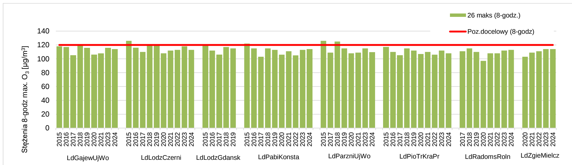
Rysunek 7.20. Przebieg 26-tych maksymalnych rocznych wartości dobowych maksimów ze stężeń średnich 8-godzinnych O 3 , na poszczególnych stanowiskach pomiarowych w województwie łódzkim, na tle poziomu docelowego w latach 2015 - 2024 [źródło: GIOŚ]
