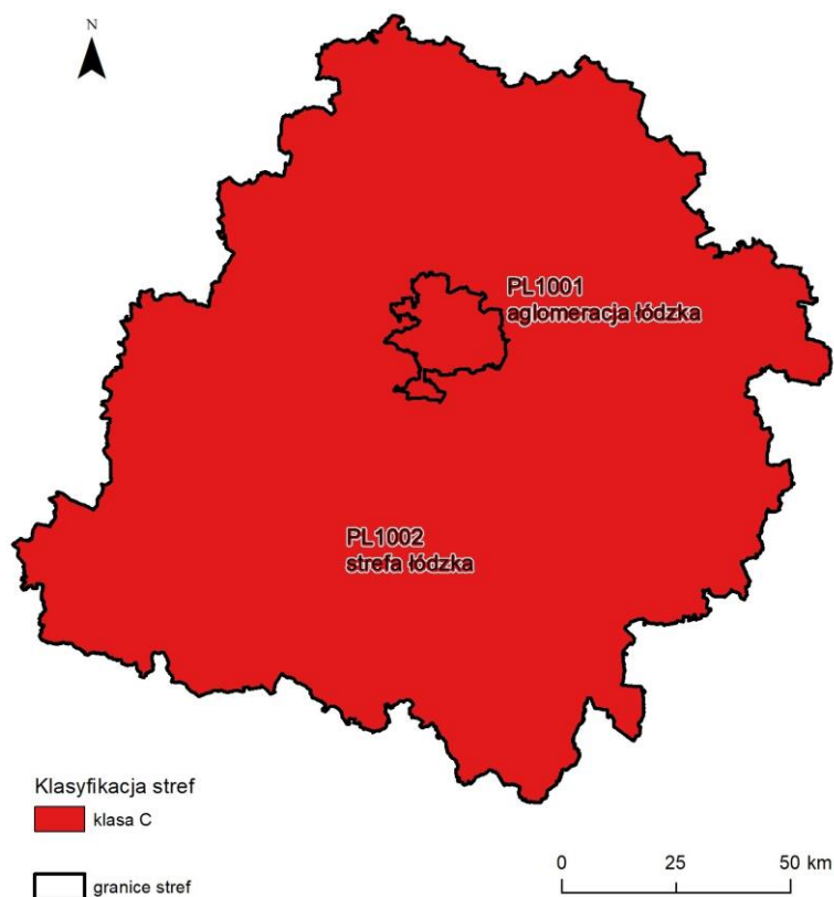
Rysunek 7.49. Klasyfikacja stref w województwie łódzkim za 2024 rok dla B(a)P w pyłe zawieszonym PM10 dla czasu uśredniania - rok, z uwzględnieniem kryteriów określonych w celu ochrony zdrowia ludzi [źródło: GIOŚ]
