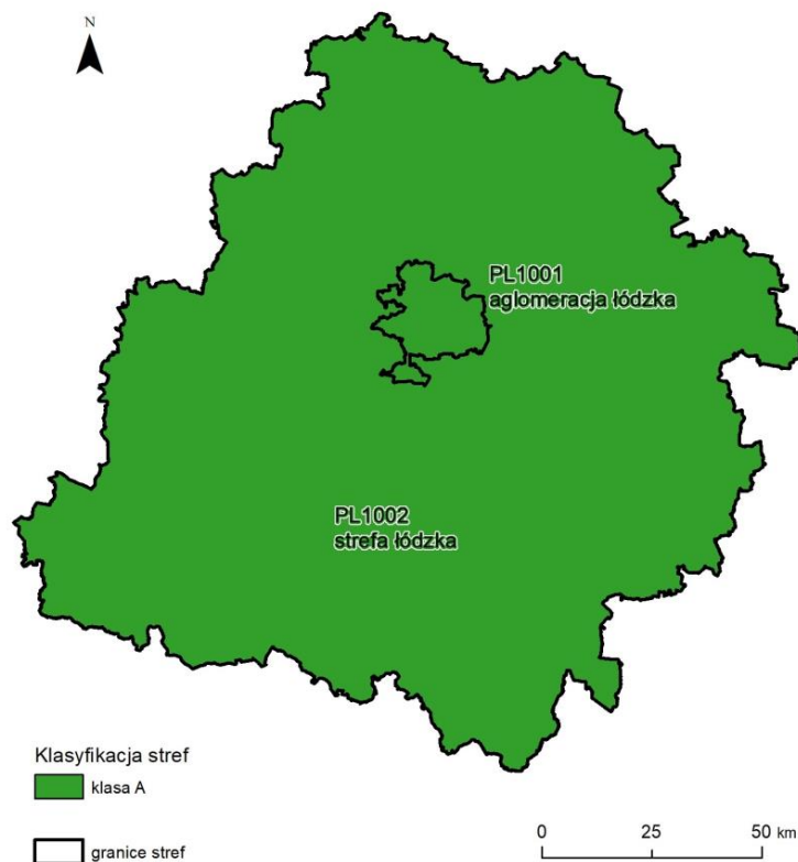
Rysunek 7.25. Klasyfikacja stref w województwie łódzkim za 2024 rok dla pyłu zawieszonego PM10, dla czasu uśredniania - 24 godz., z uwzględnieniem kryteriów określonych w celu ochrony zdrowia ludzi [źródło: GIOŚ]
