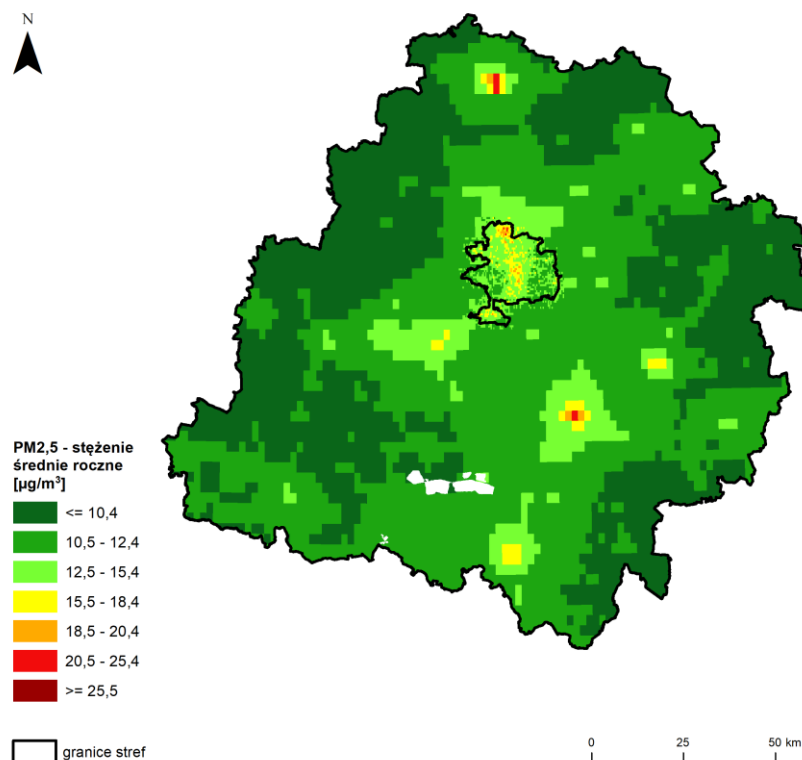
Rysunek 7.38. Rozkład przestrzenny wartości stężenia średniego rocznego pyłu zawieszonego PM2,5 w województwie łódzkim w 2024 roku, opracowany z wykorzystaniem metody szacowania w oparciu o wyniki modelowania jakości powietrza dla roku 2024 wykonanego przez IOŚ-PIB [źródło: GIOŚ, IOŚ-PIB]
