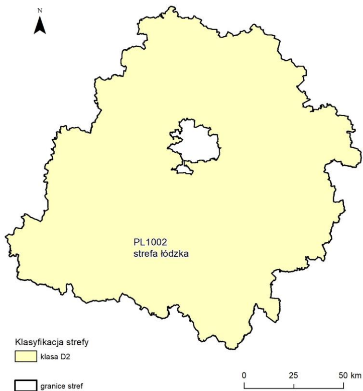
Rysunek 7.65. Klasyfikacja strefy w województwie łódzkim za 2024 rok dla O_3 dla wartości AOT40 , z uwzględnieniem kryterium poziomu celu długoterminowego określonego w celu ochrony roślin [źródło: GIOŚ]
