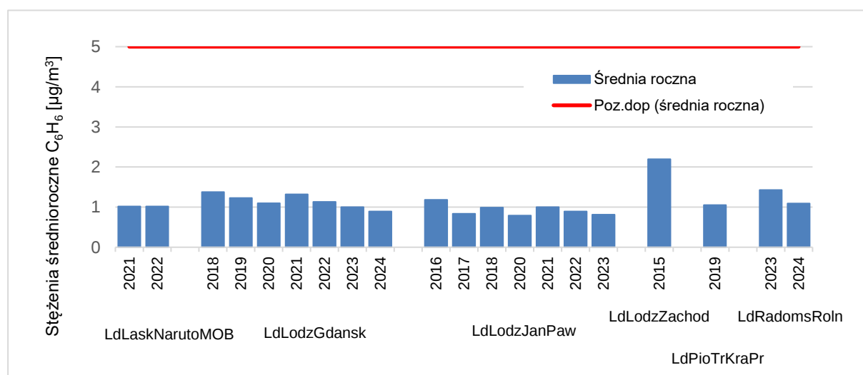
Rysunek 7.16. Przebieg wartości średnich rocznych stężeń C_6H_6 , na poszczególnych stanowiskach pomiarowych w województwie łódzkim, na tle poziomu dopuszczalnego w latach 2015 - 2024 [źródło: GIOŚ]
