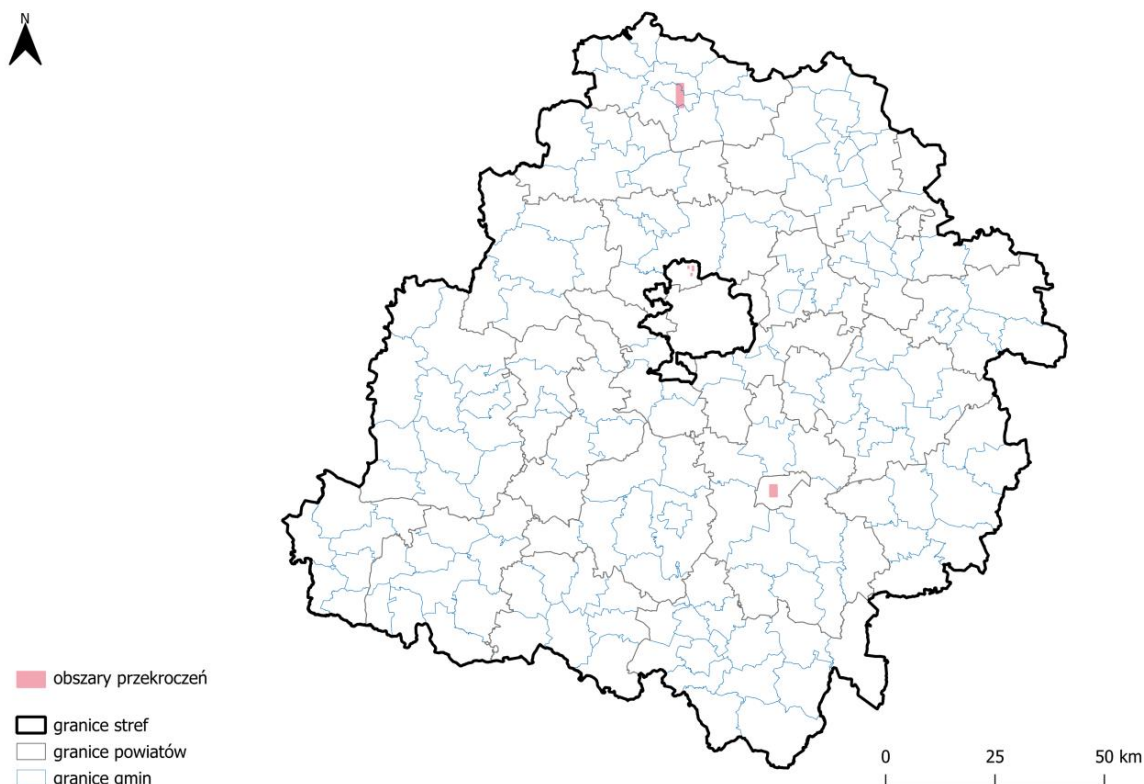
Rysunek 7.39. Zasięg obszarów przekroczeń średniorocznego poziomu dopuszczalnego pyłu zawieszonego PM 2,5 (faza II) określonego w celu ochrony zdrowia ludzi, w województwie łódzkim w 2024 roku [źródło: GIOŚ]
