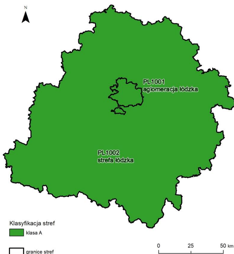
Rysunek 7.47. Klasyfikacja stref w województwie łódzkim za 2024 rok dla Ni w pyle zawieszonym PM10, dla czasu uśredniania - rok, z uwzględnieniem kryteriów określonych w celu ochrony zdrowia ludzi [źródło: GIOŚ]
