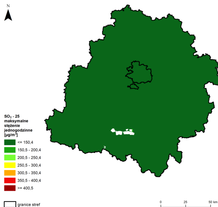
Rysunek 7.5. Rozkład przestrzenny 25 maksymalnej wartości stężenia 1-godzinne SO 2 w województwie łódzkim w 2024 roku, opracowany z wykorzystaniem metody szacowania w oparciu o wyniki modelowania jakości powietrza dla roku 2024 wykonanego przez IOŚ-PIB [źródło: GIOŚ, IOŚ-PIB]
