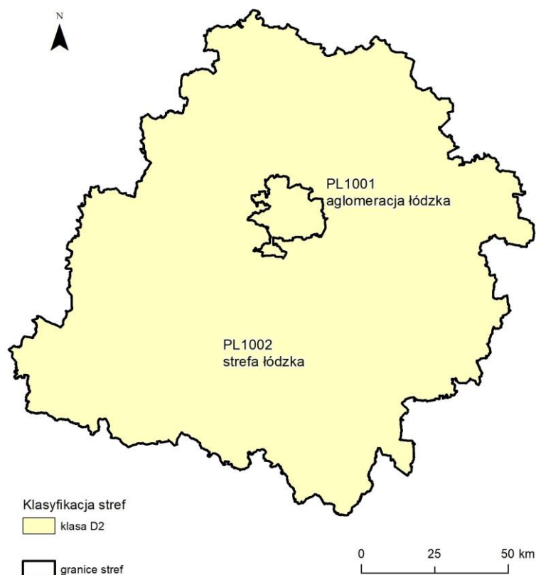
Rysunek 7.18. Klasyfikacja stref w województwie łódzkim za 2024 rok dla O_3 , w odniesieniu do poziomu celu długoterminowego, z uwzględnieniem kryteriów określonych w celu ochrony zdrowia ludzi [źródło: GIOŚ]
