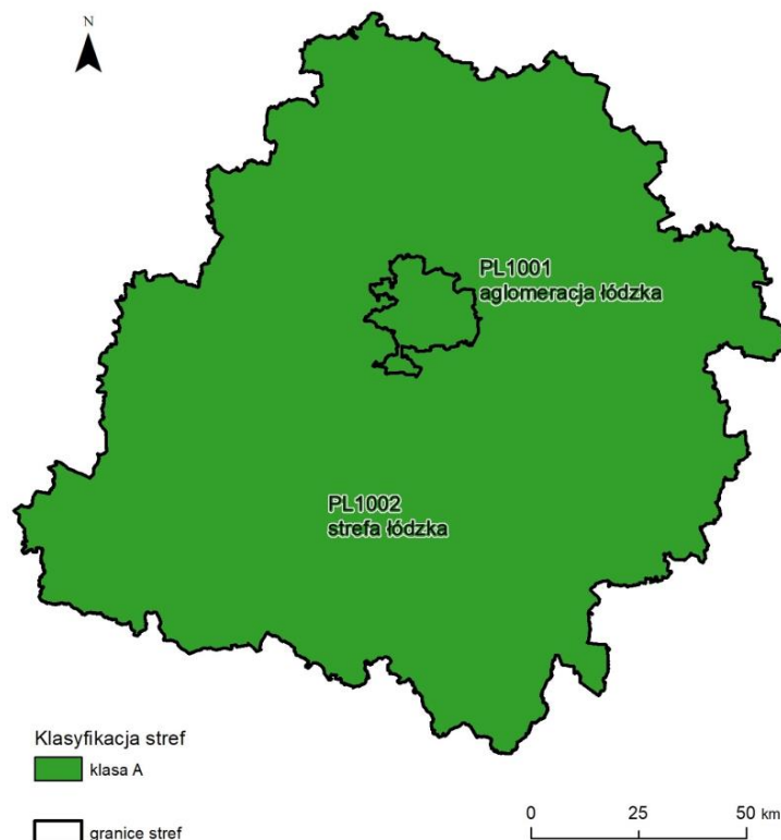
Rysunek 7.13. Klasyfikacja stref w województwie łódzkim za 2024 rok dla CO dla czasu uśredniania - 8 godz., z uwzględnieniem kryteriów określonych w celu ochrony zdrowia ludzi [źródło: GIOŚ]
