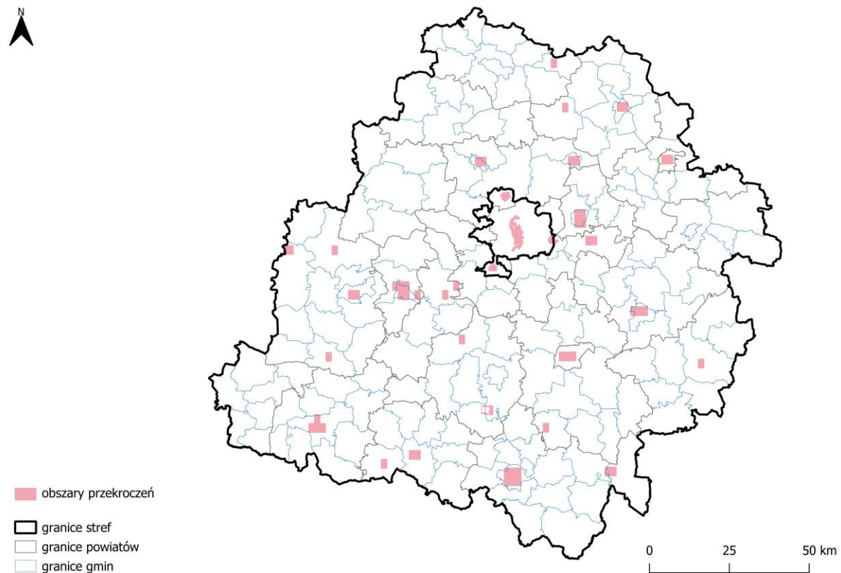
Rysunek 2. Zasięg obszarów przekroczeń poziomu docelowego B(a)P w pyłe zawieszonym PM10 w województwie łódzkim w 2024 roku [źródło: GIOŚ]
