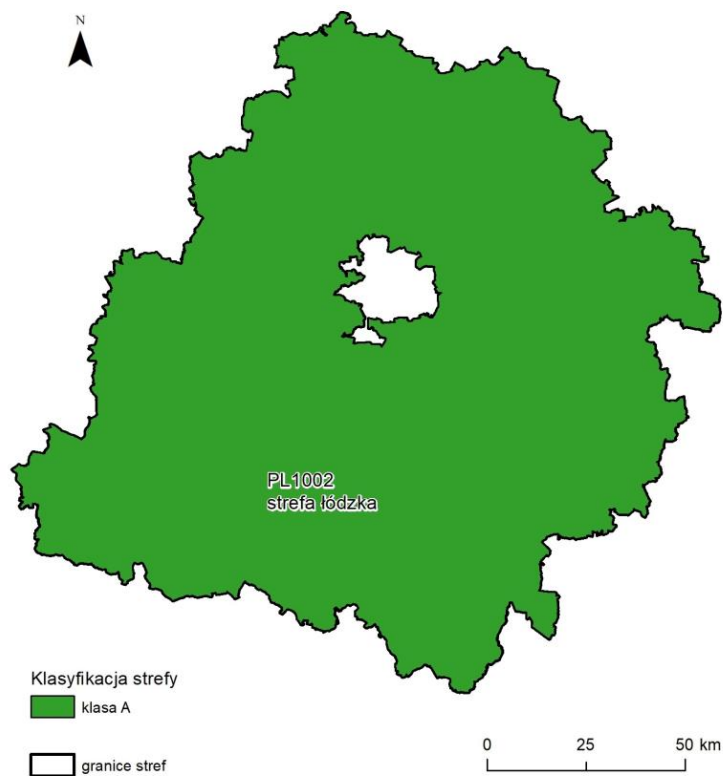
Rysunek 7.64. Klasyfikacja strefy w województwie łódzkim za 2024 rok dla O_3 dla wartości AOT40_{5L} , z uwzględnieniem kryterium poziomu docelowego określonego w celu ochrony roślin [źródło: GIOŚ]
