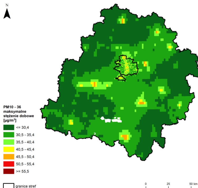
Rysunek 7.33. Rozkład przestrzenny 36 maksymalnej wartości stężenia 24-godzinnego pyłu zawieszonego PM10 w województwie łódzkim w 2024 roku, opracowany z wykorzystaniem metody szacowania w oparciu o wyniki modelowania jakości powietrza dla roku 2024 wykonanego przez IOŚ-PIB [źródło: GIOŚ, IOŚ-PIB]
