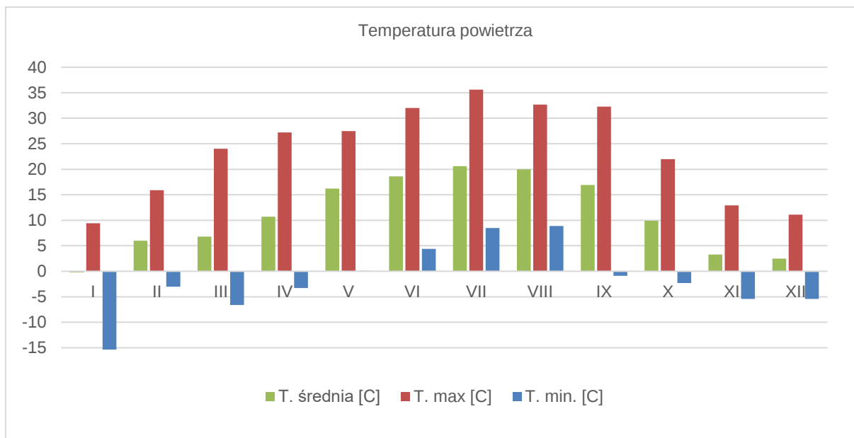
Rysunek 5.3. Miesięczna temperatura powietrza w Łodzi w 2024 roku [opracowanie GIOŚ, źródło: IMGW-PIB]
