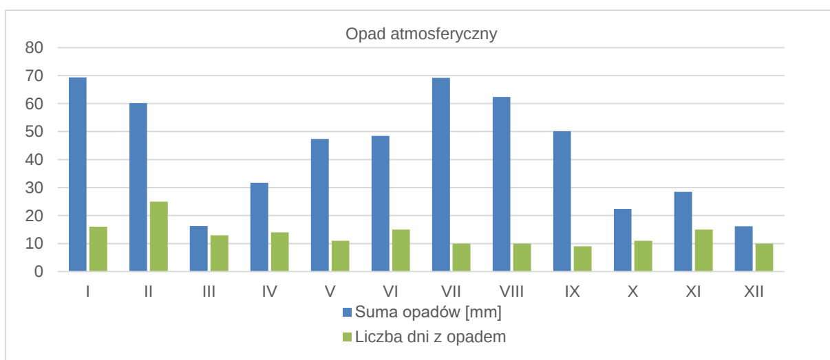
Rysunek 5.4. Miesięczny opad atmosferyczny w Łodzi w 2024 roku [opracowanie GIOŚ, źródło: IMGW-PIB]
