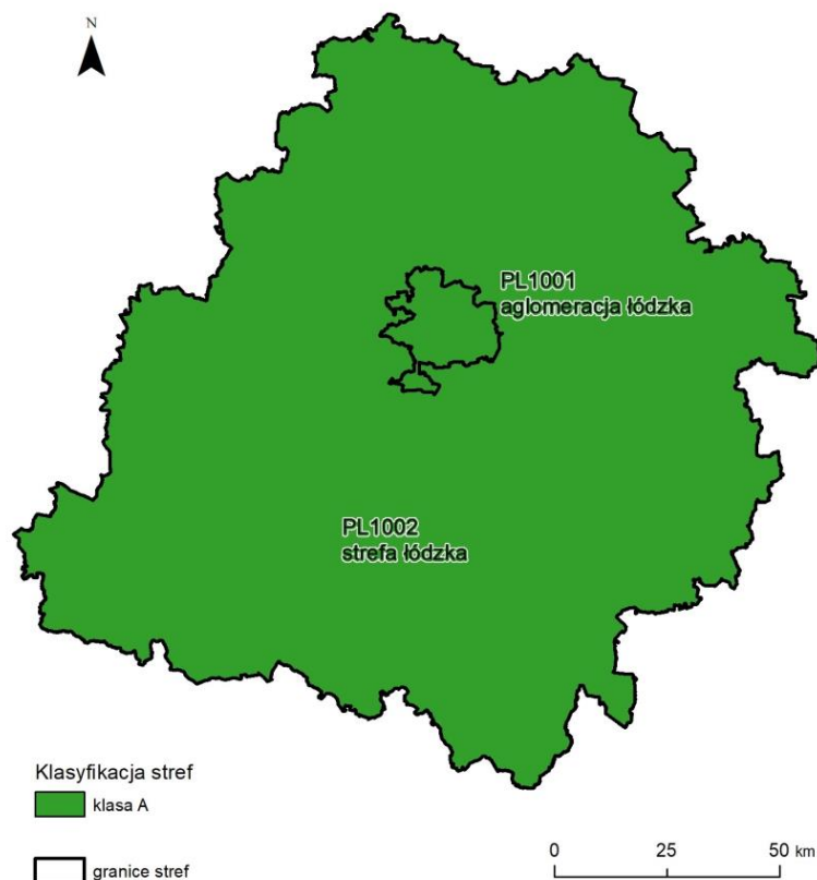
Rysunek 7.42. Klasyfikacja stref w województwie łódzkim za 2024 rok dla As w pyłe zawieszonym PM10, dla czasu uśredniania - rok, z uwzględnieniem kryteriów określonych w celu ochrony zdrowia ludzi [źródło: GIOŚ]
