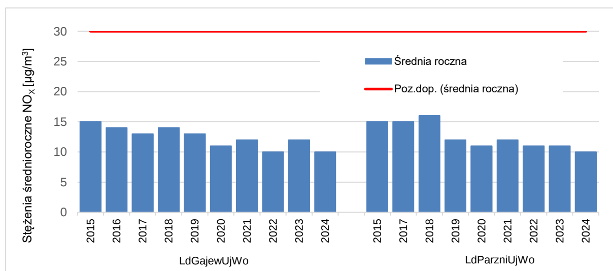
Rysunek 7.62. Przebieg wartości średnich rocznych stężeń NO x , na stanowiskach pomiarowych w województwie łódzkim uwzględnionych w ocenie pod kątem ochrony roślin, na tle poziomu dopuszczalnego w latach 2015 - 2024 [źródło: GIOŚ]
