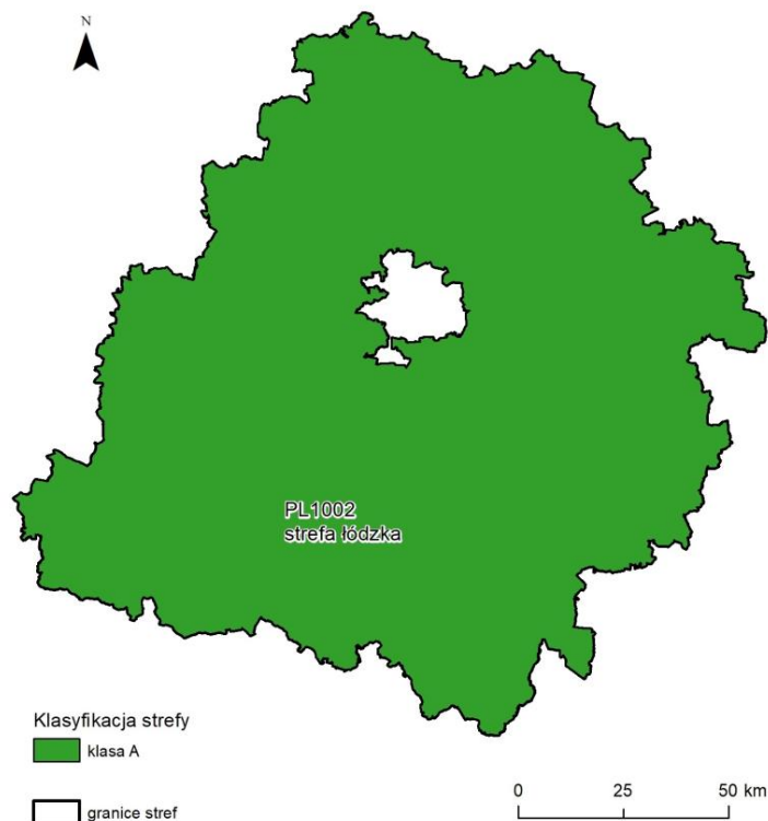
Rysunek 7.56. Klasyfikacja strefy w województwie łódzkim za 2024 rok dla \text{SO}_2 dla czasu uśredniania – pora zimowa, z uwzględnieniem kryteriów określonych w celu ochrony roślin [źródło: GIOŚ]
