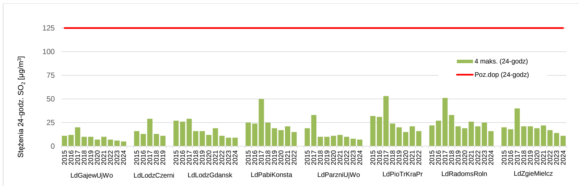
Rysunek 7.4. Przebieg 4 maksymalnej wartości dobowej stężenia SO 2 , na poszczególnych stanowiskach pomiarowych w województwie łódzkim, na tle poziomu dopuszczalnego w latach 2015 – 2024 [źródło: GIOŚ]
