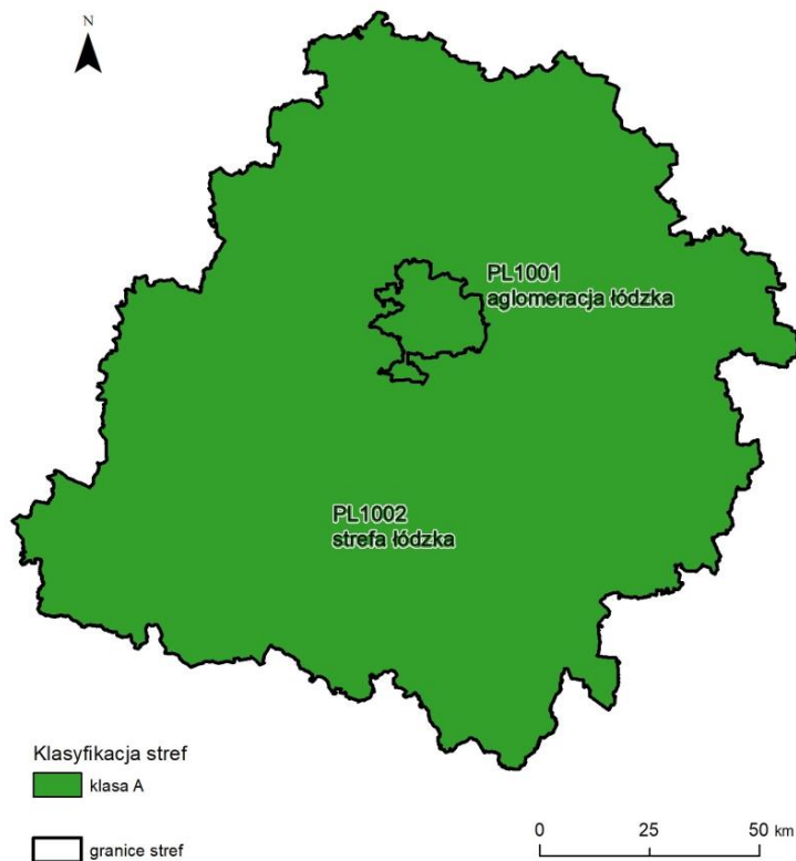
Rysunek 7.26. Klasyfikacja stref w województwie łódzkim za 2024 rok dla pyłu zawieszonego PM10, dla czasu uśredniania - rok, z uwzględnieniem kryteriów określonych w celu ochrony zdrowia ludzi [źródło: GIOŚ]
