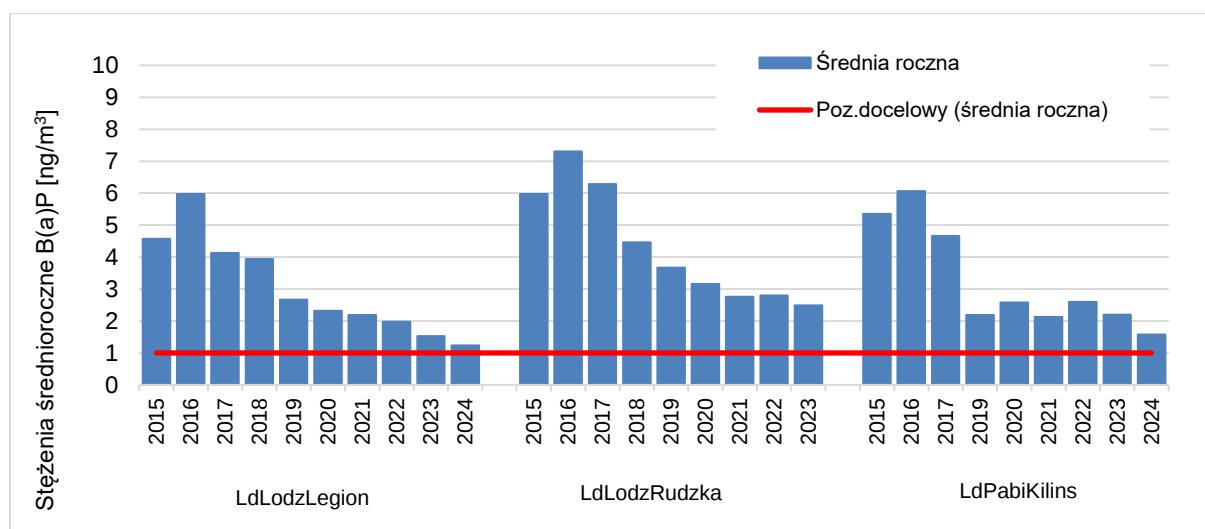
Rysunek 7.50. Przebieg wartości średnich rocznych stężeń B(a)P w pyłe zawieszonym PM10 na stanowiskach pomiarowych w województwie łódzkim, na tle poziomu docelowego w latach 2015 – 2024 (strefa oceny aglomeracja łódzka) (zgodnie z zasadami zaokrąglania wyników opisanymi w rozdz. 2.2 wartości poniżej 1,5 ng/m 3 nie stanowią przekroczenia poziomu docelowego benzo(a)pirenu w pyłe zawieszonym PM10) [źródło: GIOŚ]
