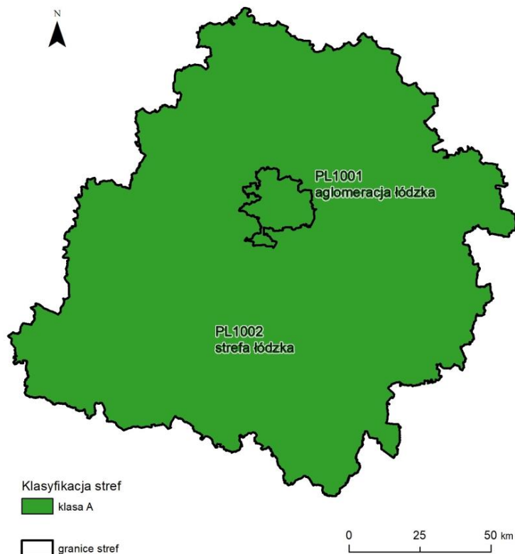
Rysunek 7.7. Klasyfikacja stref w województwie łódzkim za 2024 rok dla NO 2 dla czasu uśredniania - 1 godz., z uwzględnieniem kryteriów określonych w celu ochrony zdrowia ludzi [źródło: GIOŚ]
