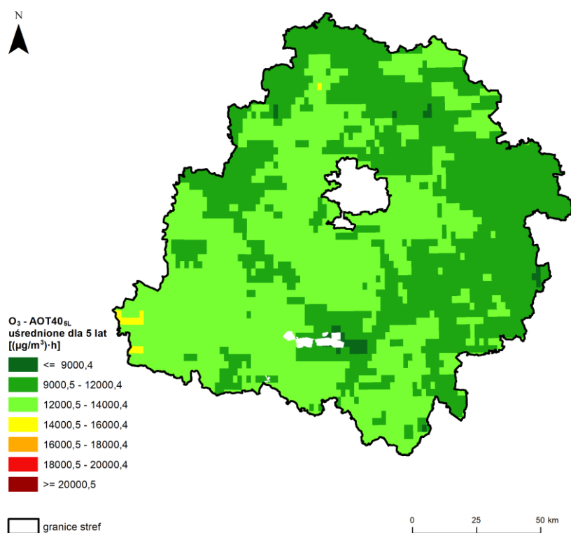
Rysunek 7.68. Rozkład przestrzenny wartości poziomu docelowego (wskaźnik AOT40 5L ) uśrednionego dla okresu 5 lat w województwie łódzkim, opracowany z wykorzystaniem metody szacowania w oparciu o wyniki modelowania jakości powietrza dla roku 2024 wykonanego przez IOŚ-PIB [źródło: GIOŚ, IOŚ-PIB]
