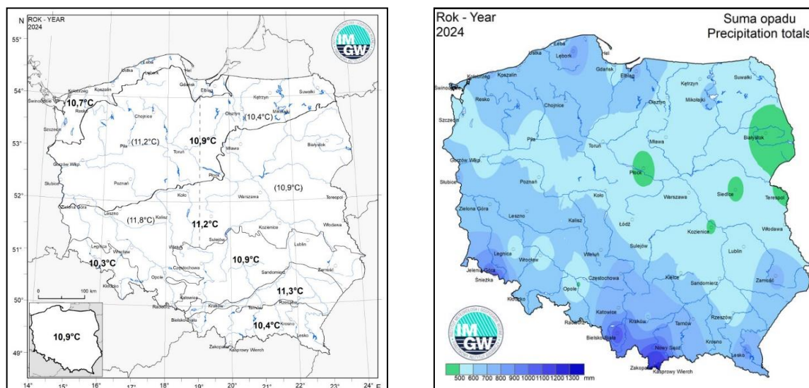
Rysunek 5.2. Przestrzenny rozkład wartości wybranych parametrów meteorologicznych w 2024 r. w Polsce: z lewej strony - wartości średniej obszarowej rocznej temperatury powietrza w poszczególnych regionach klimatycznych Polski, z prawej - roczne sumy opadów atmosferycznych [źródło: IMGW-PIB, https://klimat.imgw.pl/ ]
