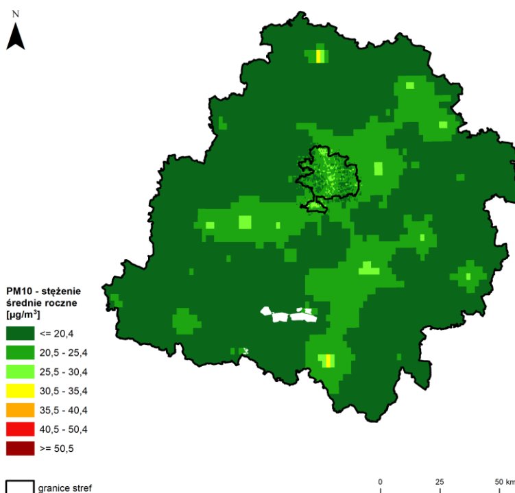
Rysunek 7.34. Rozkład przestrzenny wartości stężenia średniego rocznego pyłu zawieszonego PM10 w województwie łódzkim w 2024 roku, opracowany z wykorzystaniem metody szacowania w oparciu o wyniki modelowania jakości powietrza dla roku 2024 wykonanego przez IOŚ-PIB [źródło: GIOŚ, IOŚ-PIB]
