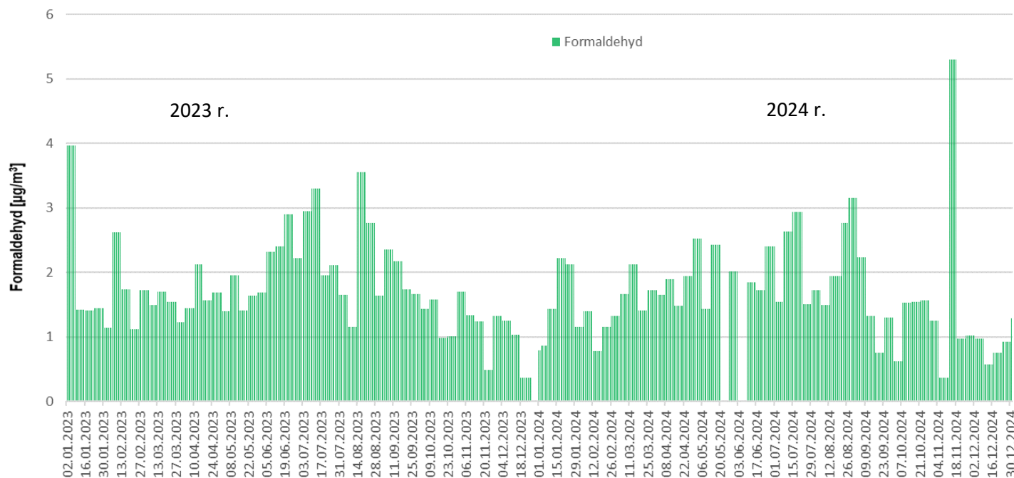
Rys. 3. Stężenia tygodniowe formaldehydu pomierzone w latach 2023-2024 na stacji w Żarach, przy ul. Szymanowskiego
