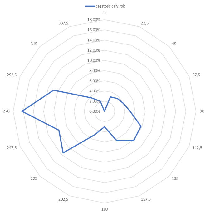
Rys. 4. Róża wiatrów na podstawie pomiarów meteorologicznych uzyskanych w 2024 r. na stacji w Żarach przy ul. Szymanowskiego
