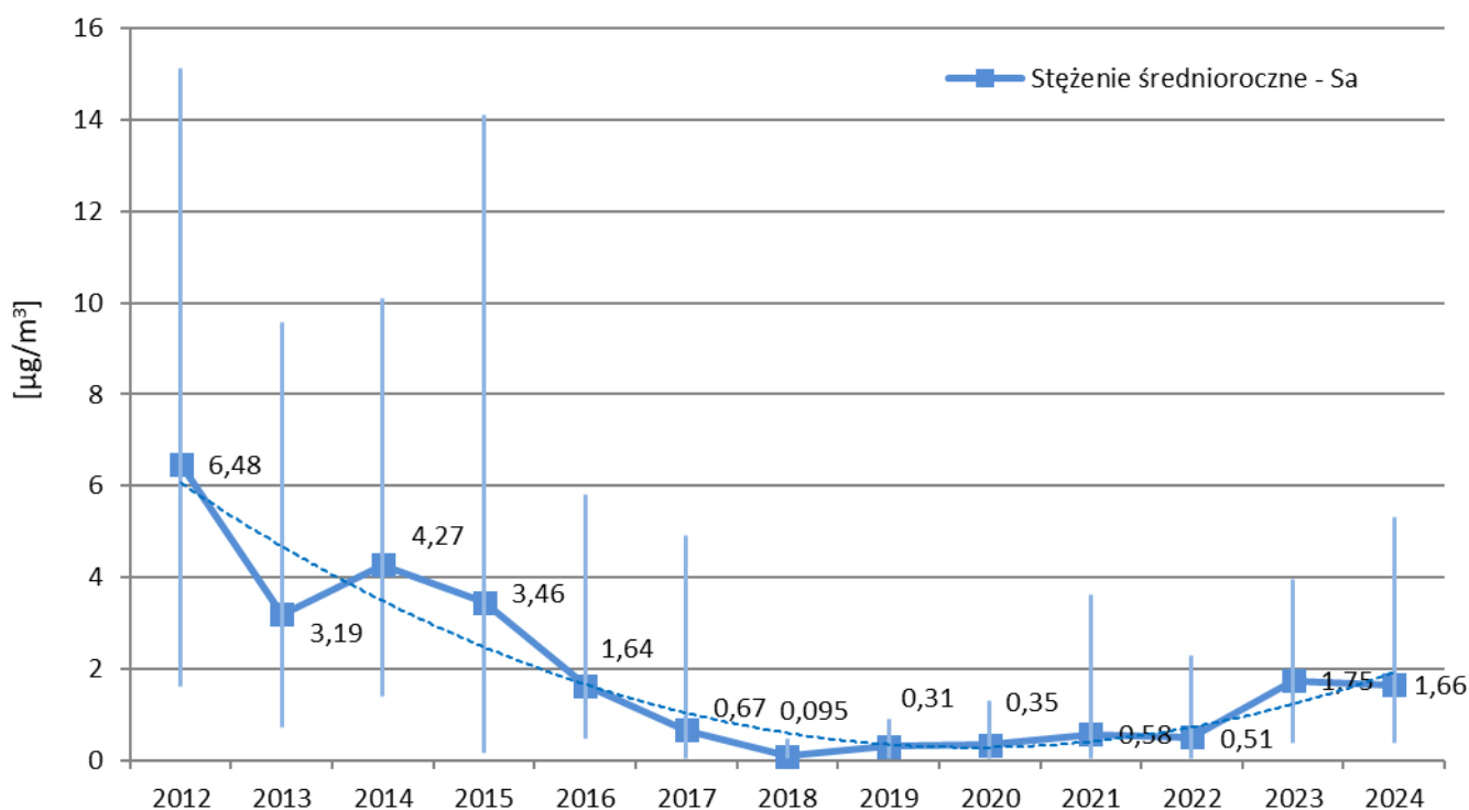
Rys. 1. Stężenia średnioroczne formaldehydu pomierzone w latach 2012-2024 na stacji w Żarach, przy ul. Szymanowskiego, wraz ze stężeniami dobowymi minimalnymi i maksymalnymi w danym roku w latach 2012-2024
