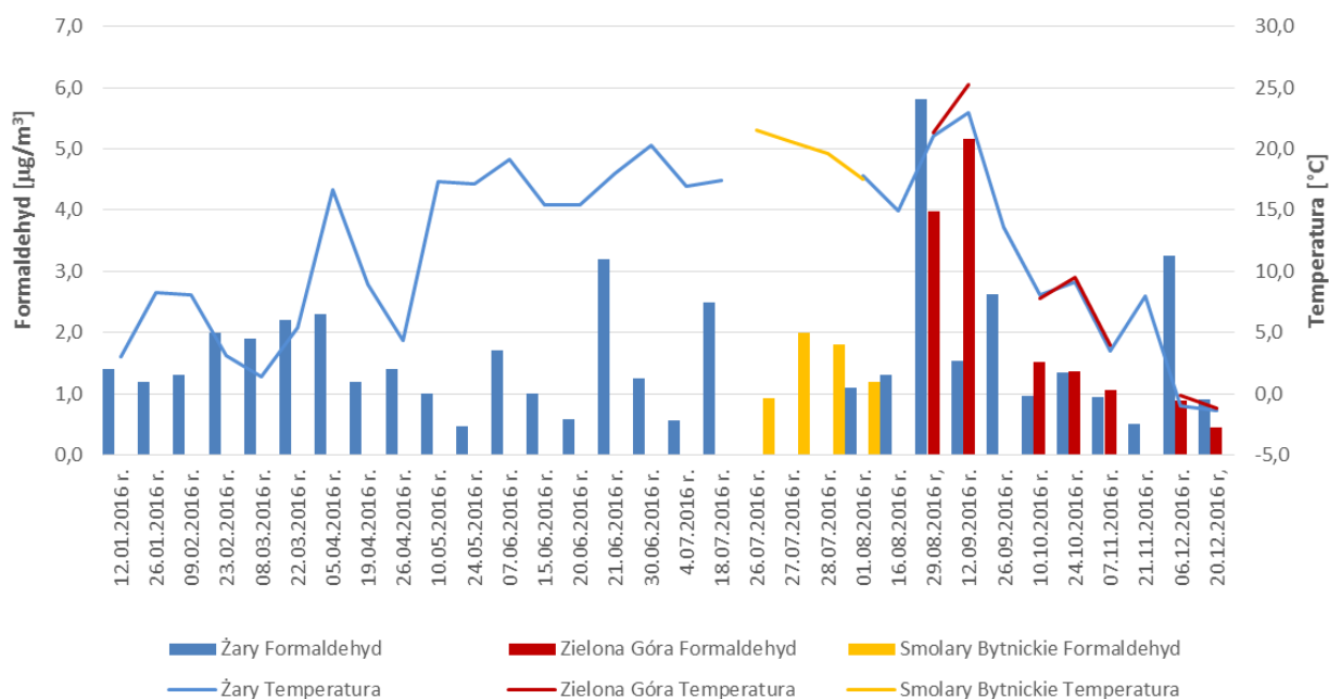
Rys. 5. Stężenia dobowe formaldehydu pomierzone w 2016 r. na stacjach: w Żarach, w Zielonej Górze oraz w Smolarach Bytnickich
