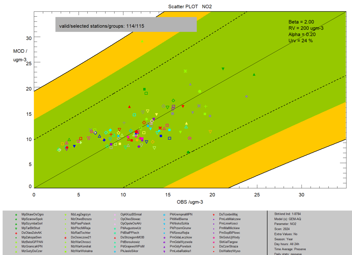
Rysunek 9. Wykres rozrzutu dla NO 2 , wyniki modelu GEM-AQ względem pomiarów, rok 2024
