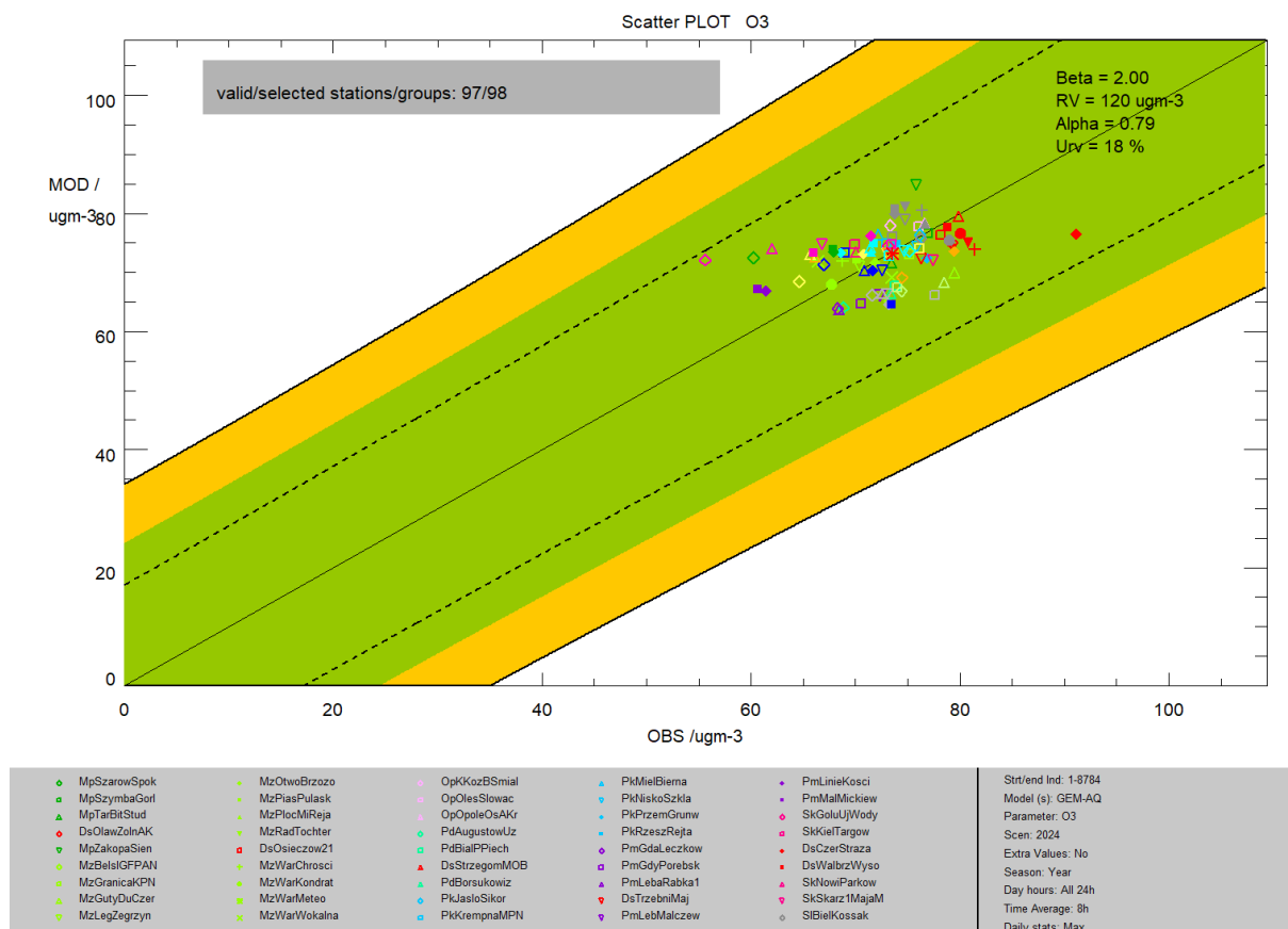
Rysunek 13. Wykres rozrzutu dla O 3 , wyniki modelu GEM-AQ względem pomiarów, rok 2024
