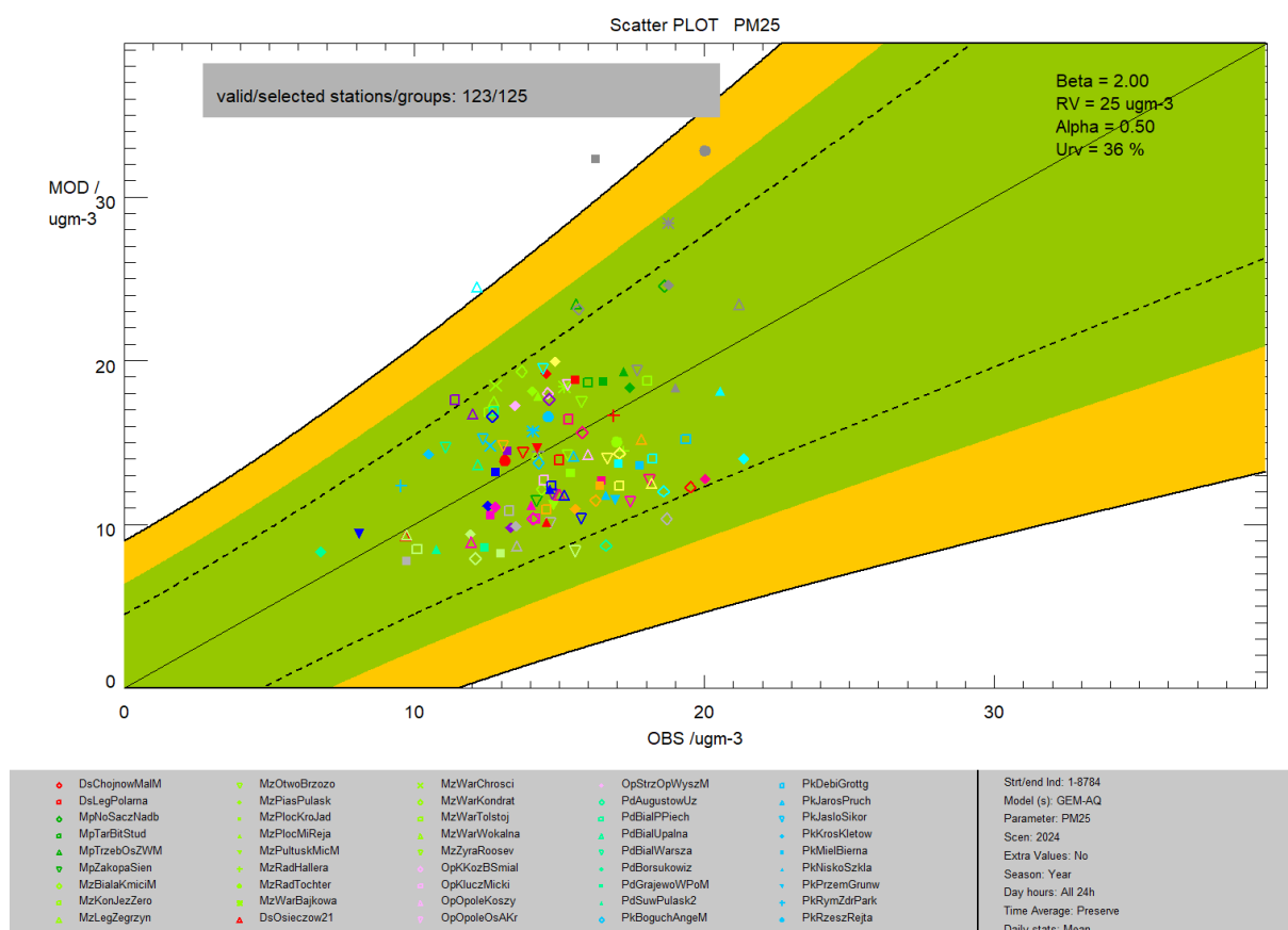
Rysunek 5. Wykres rozrzutu dla pyłu PM2,5, wyniki modelu GEM-AQ względem pomiarów, rok 2024
