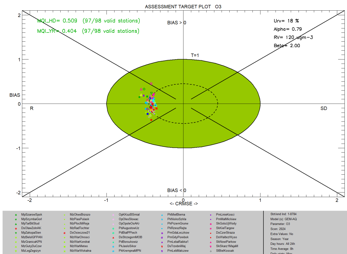
Rysunek 15. Diagram celu dla O 3 , wyniki modelu GEM-AQ względem pomiarów, rok 2024
