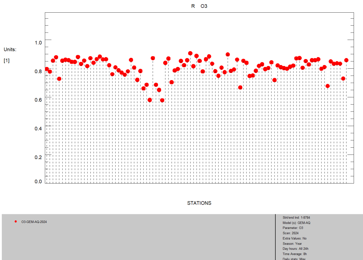
Rysunek 14. Wykres słupkowy współczynnika korelacji dla O 3 , wyniki modelu GEM-AQ względem pomiarów, rok 2024
