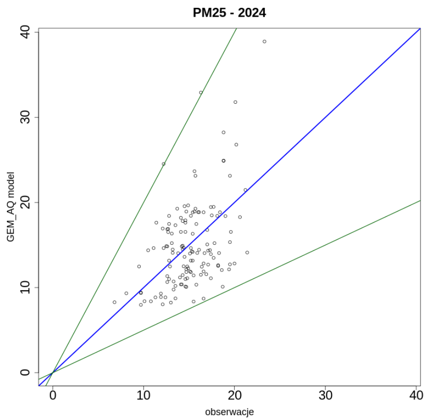
Rysunek 24. Wykres rozrzutu dla średnich rocznych stężeń PM2,5
