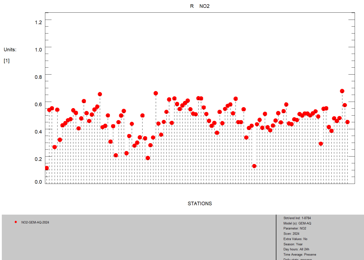
Rysunek 10. Wykres słupkowy współczynnika korelacji dla NO 2 , wyniki modelu GEM-AQ względem pomiarów, rok 2024
