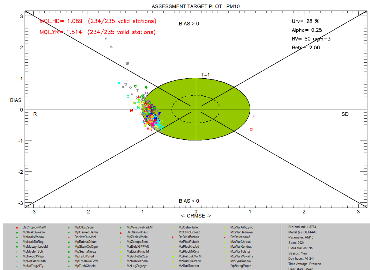
Rysunek 3. Diagram celu dla pyłu PM10, wyniki modelu GEM-AQ względem pomiarów, rok 2024
