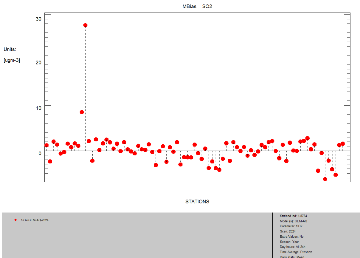
Rysunek 19. Wykres słupkowych średnich błędów dla \text{SO}_2 , wyniki modelu GEM-AQ względem pomiarów, rok 2024
