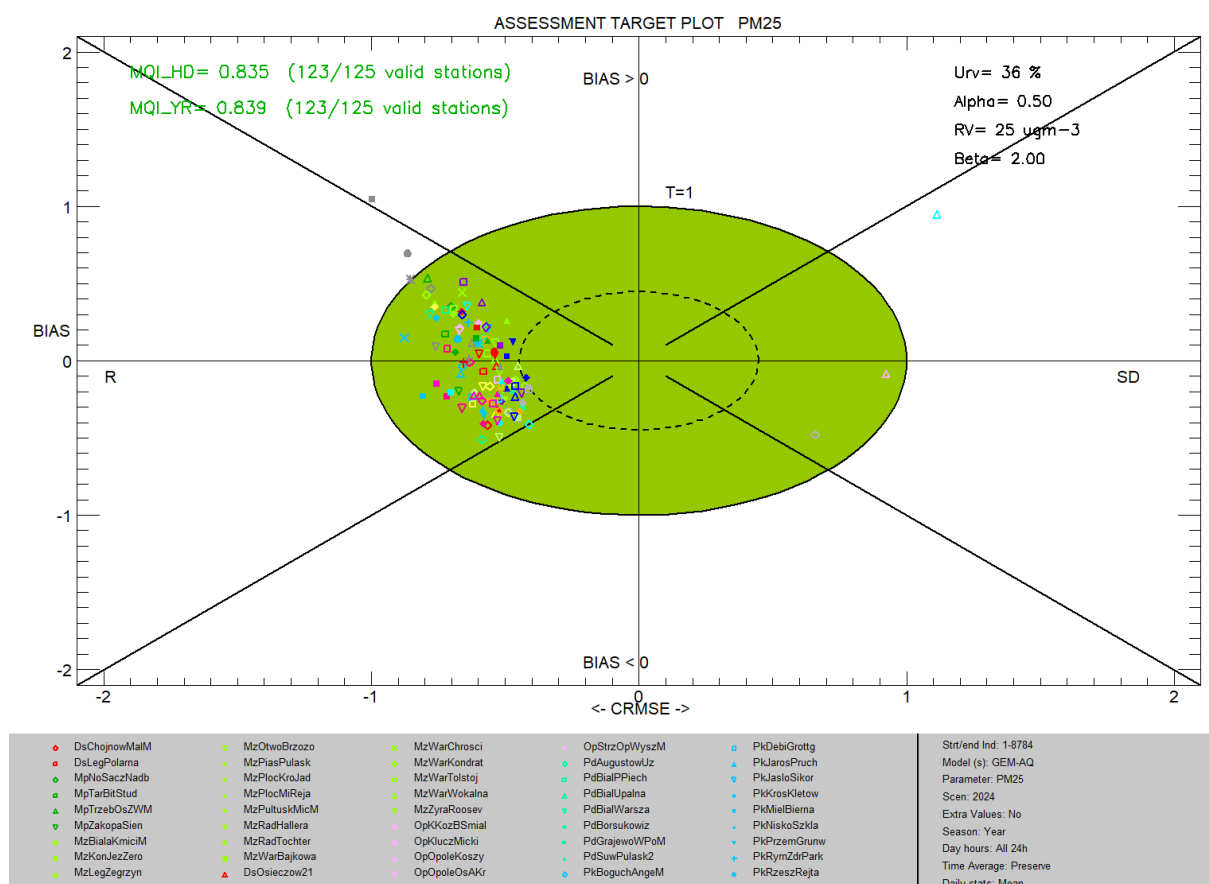
Rysunek 7. Diagram celu dla pyłu PM 2,5 , wyniki modelu GEM-AQ względem pomiarów, rok 2024
