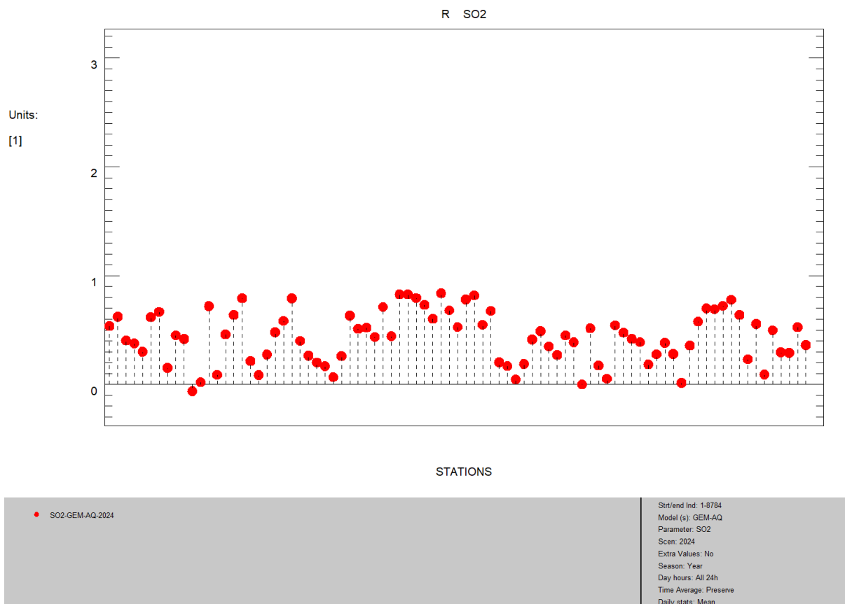
Rysunek 18. Wykres słupkowy współczynnika korelacji dla \text{SO}_2 , wyniki modelu GEM-AQ względem pomiarów, rok 2024
