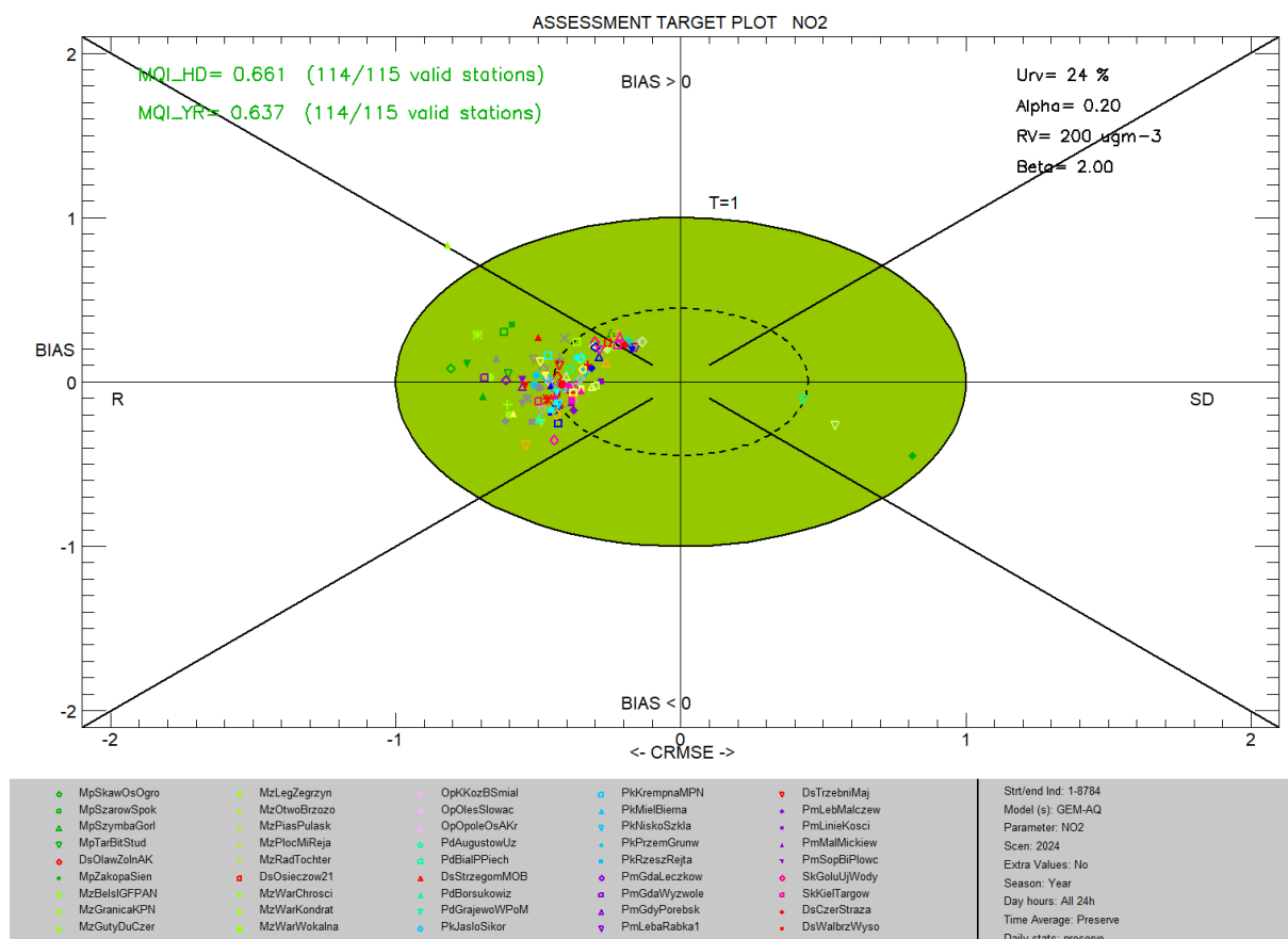
Rysunek 11. Diagram celu dla NO 2 , wyniki modelu GEM-AQ względem pomiarów, rok 2024
