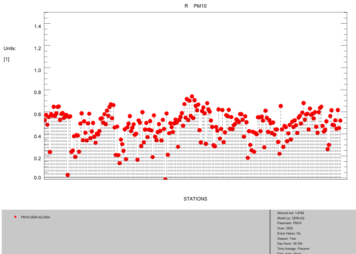
Rysunek 2. Wykres słupkowy współczynnika korelacji dla pyłu PM10, wyniki modelu GEM-AQ względem pomiarów, rok 2024
