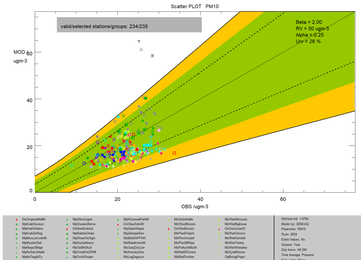
Rysunek 1. Wykres rozrzutu dla pyłu PM10, wyniki modelu GEM-AQ względem pomiarów, rok 2024
