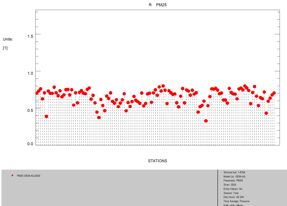
Rysunek 6. Wykres słupkowy współczynnika korelacji dla pyłu PM 2,5 , wyniki modelu GEM-AQ względem pomiarów, rok 2024
