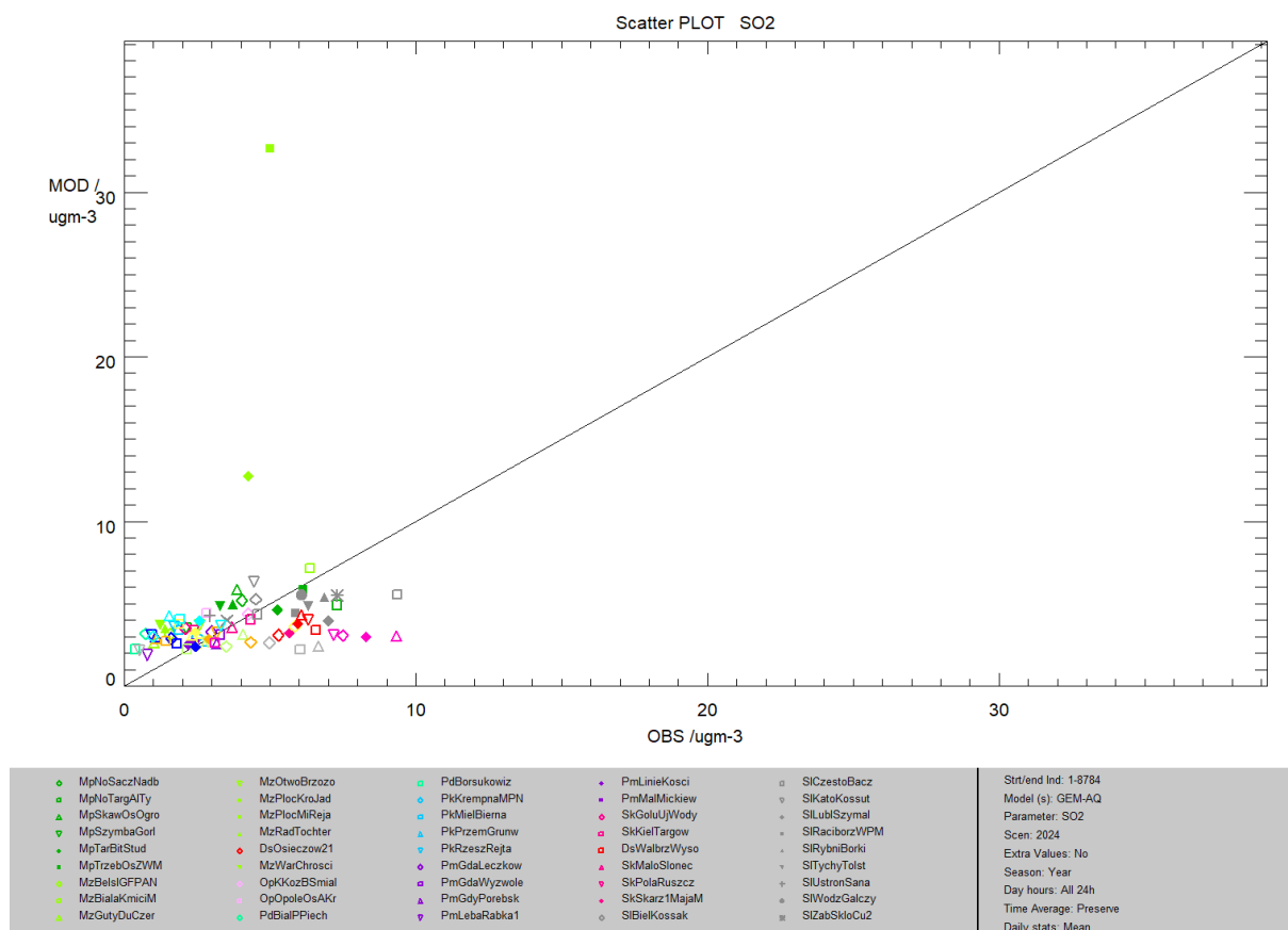
Rysunek 17. Wykres rozrzutu dla SO 2 , wyniki modelu GEM-AQ względem pomiarów, rok 2024
